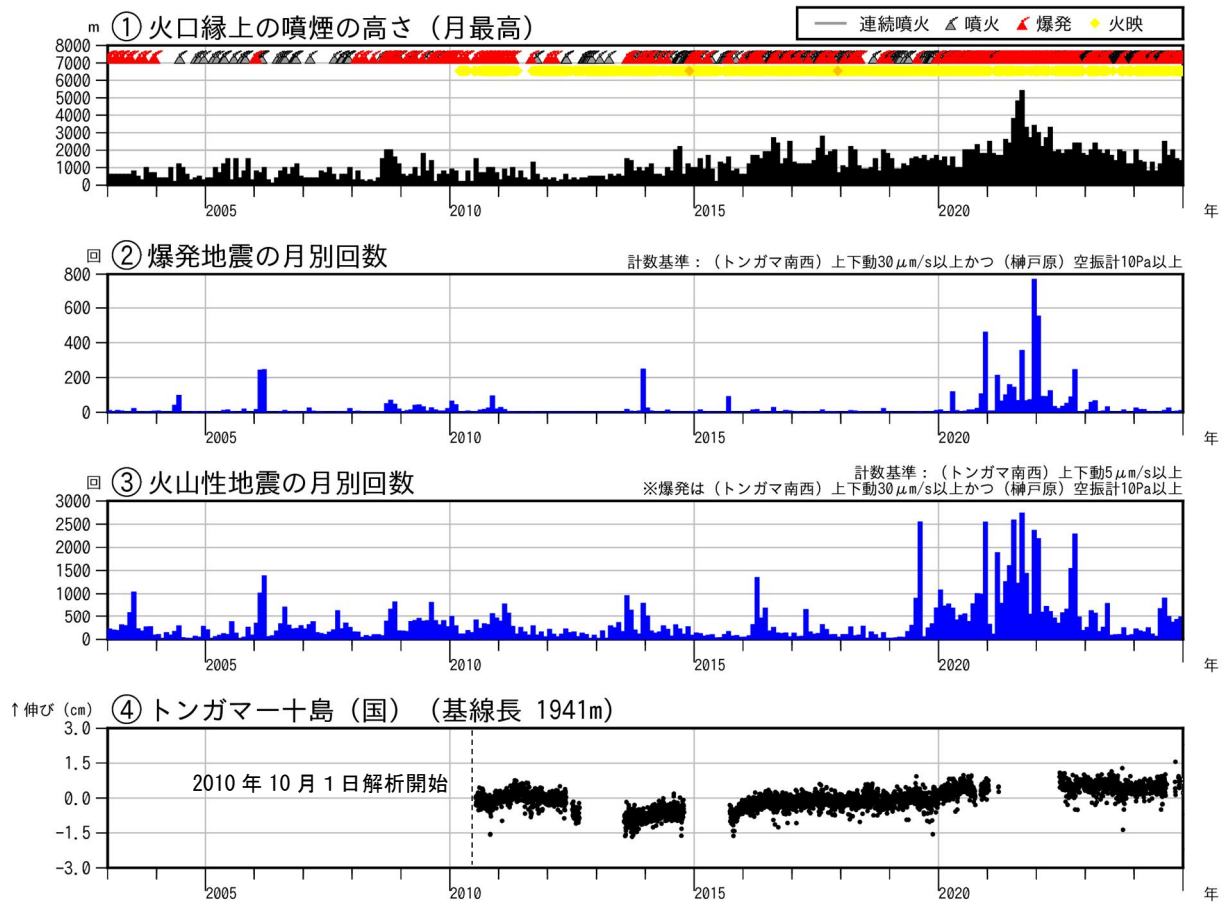
図2 諏訪之瀬島 長期の火山活動経過図（2003年1月～2024年12月）
