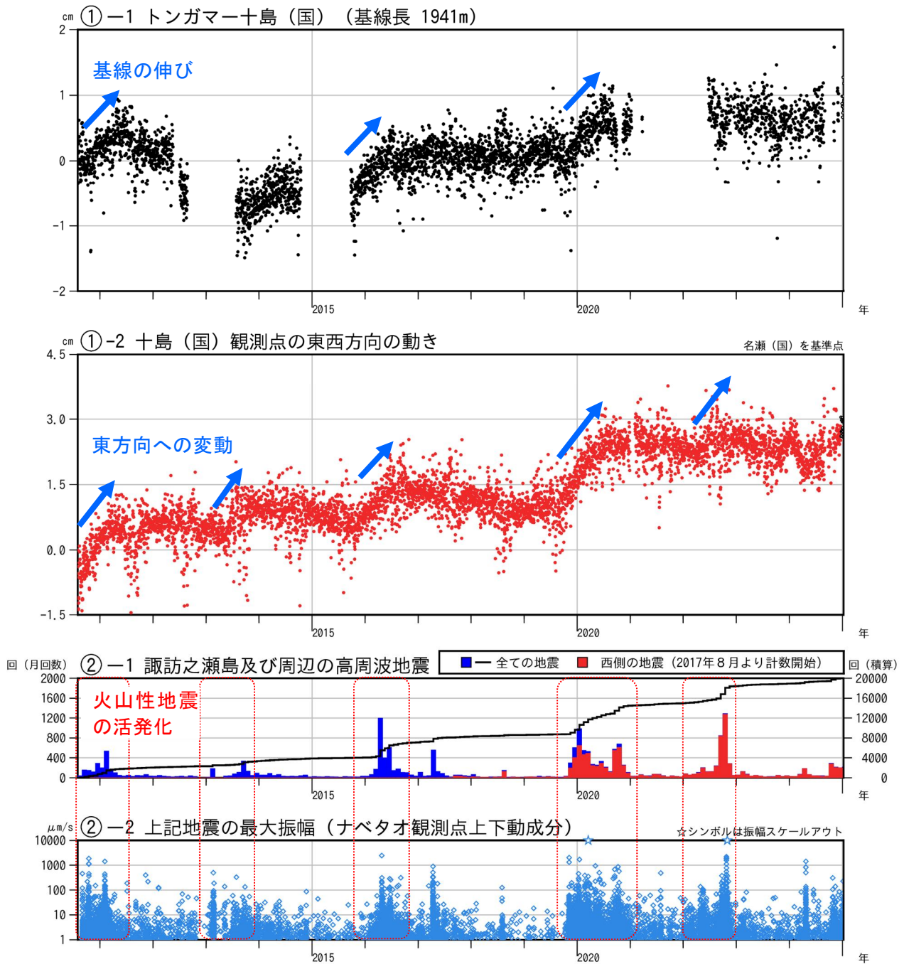
図6 諏訪之瀬島 GNSS連続観測と周辺の火山性地震（2010年8月～2024年12月）
