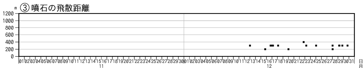
図5 諏訪之瀬島 ナベタオ観測点の傾斜変動と噴火活動（2024年11月～12月）
