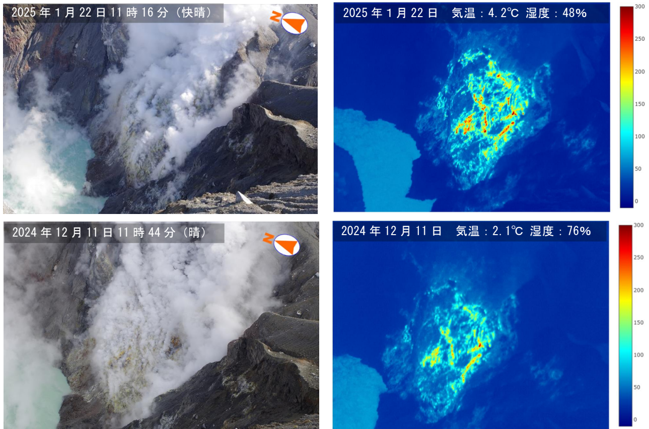
図 2-2 阿蘇山 中岳第一火口 南側火口壁の状況 (火口南西側観測定点から撮影 上図：1月22日、下図：2024年12月11日)
