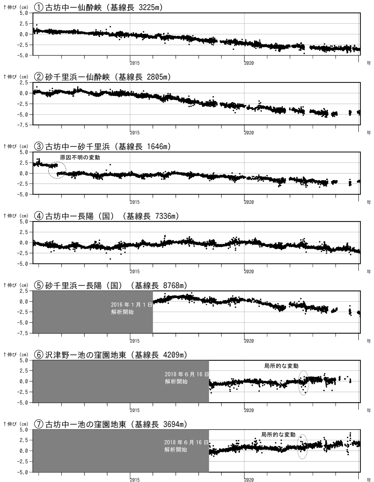
図5 阿蘇山 GNSS 連続観測による基線長変化（2010年11月～2025年1月）
