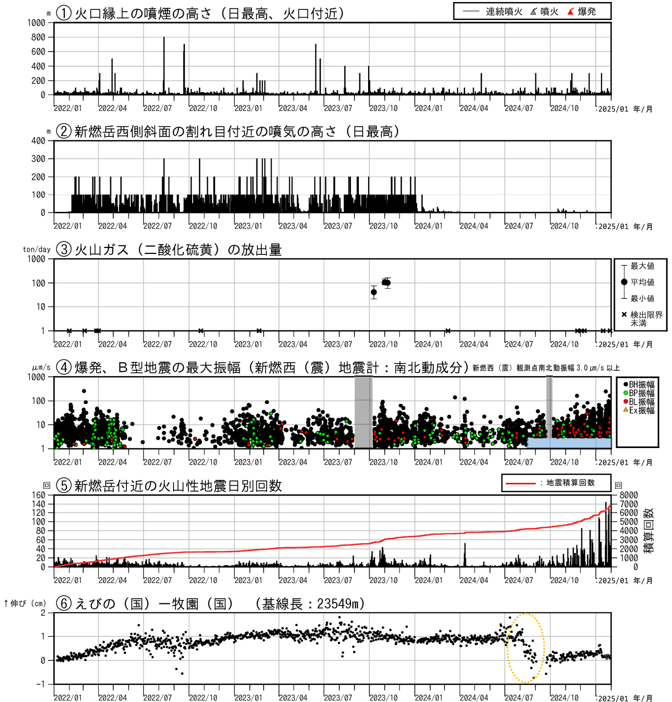
図3 霧島山（新燃岳） 火山活動経過図（2022年1月～2025年1月31日）
