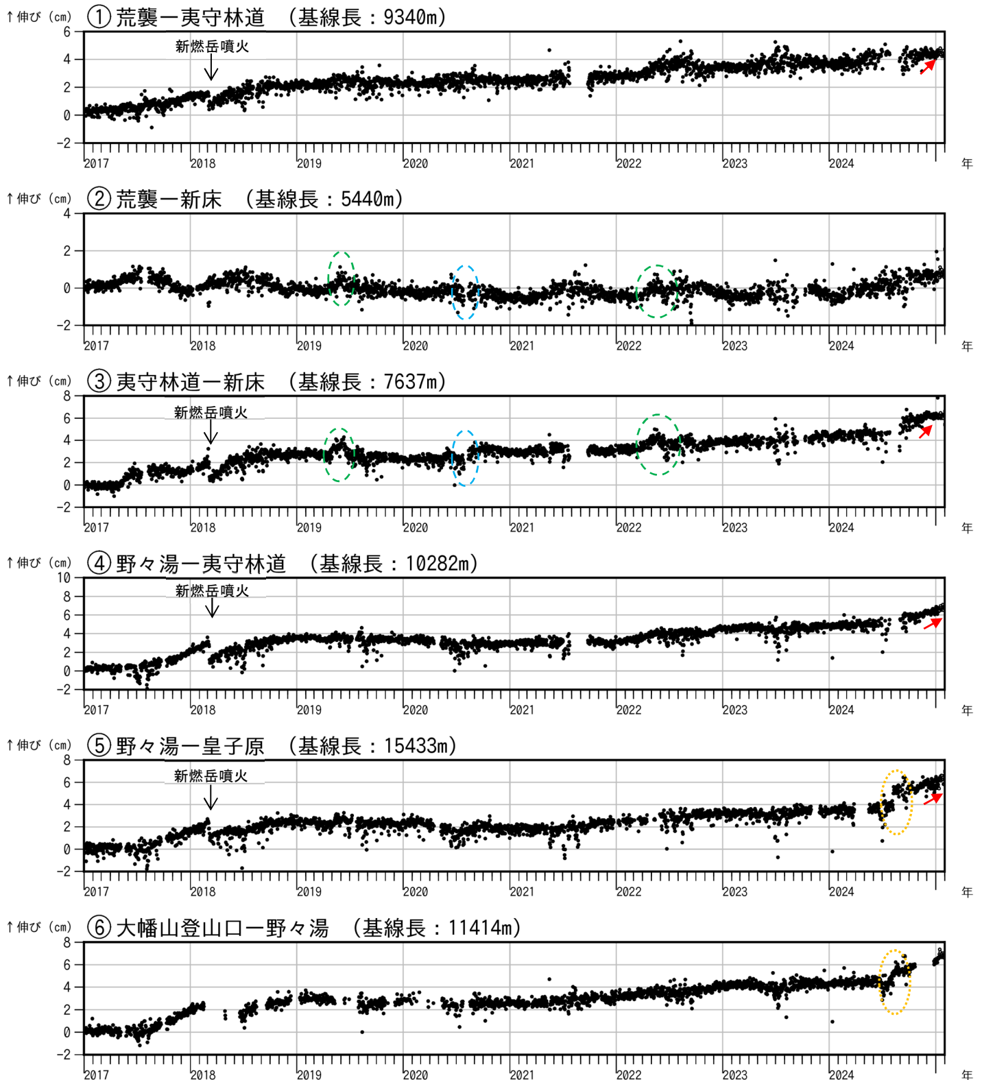
図5 霧島山（新燃岳） GNSS 連続観測による基線長変化（2017年1月～2025年1月）
