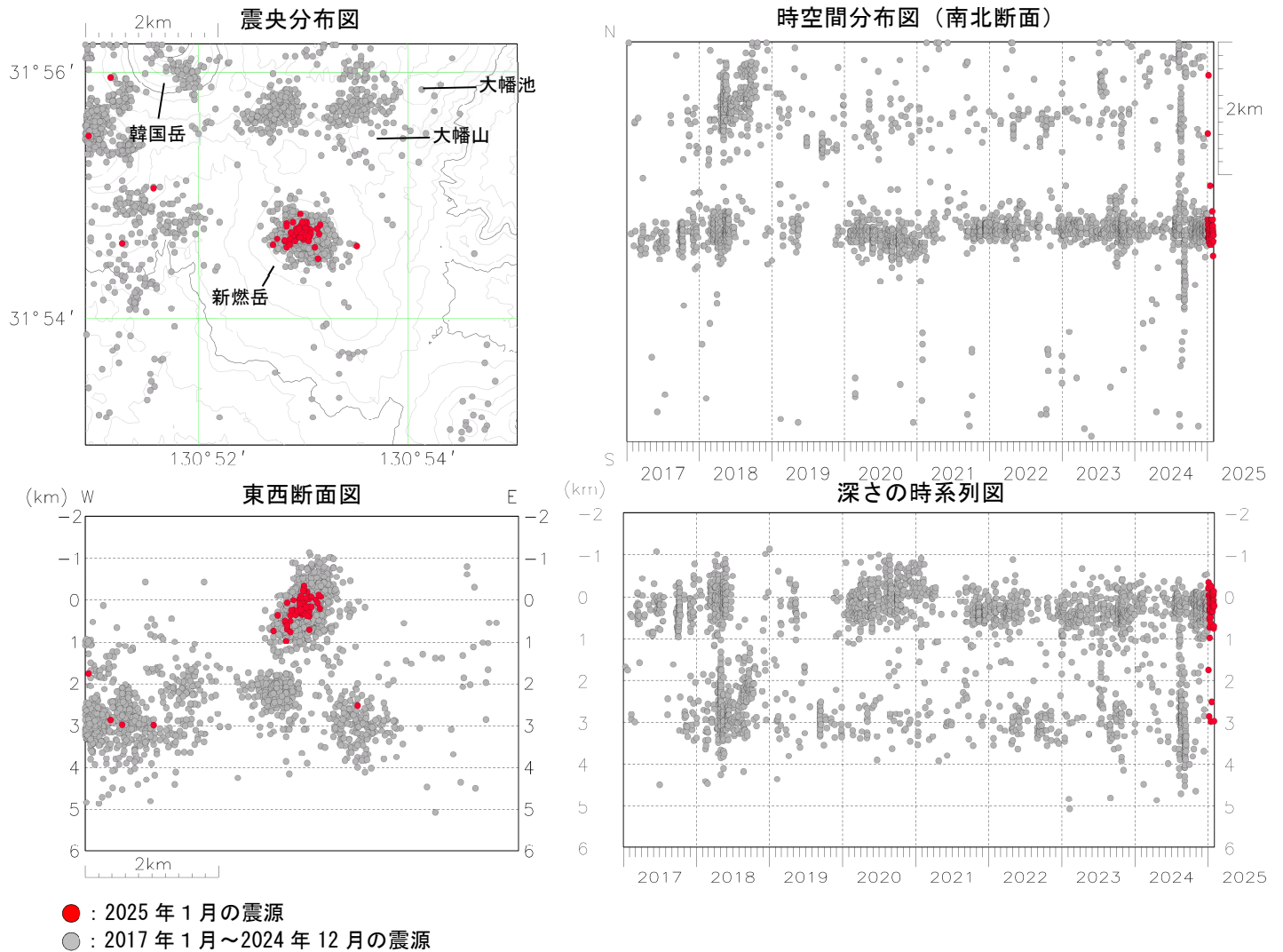
図 4 霧島山（新燃岳） 震源分布図（2017 年 1 月～2025 年 1 月）
