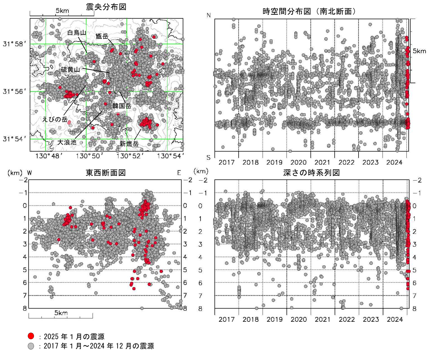
図3 霧島山（えびの高原（硫黄山）周辺） 震源分布図（2017 年 1 月～2025 年 1 月）
