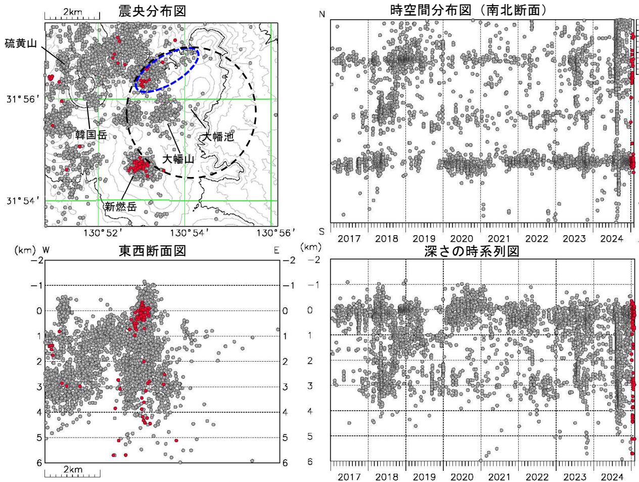
図3 霧島山（大幡池） 震源分布図（2017年1月～2025年1月）
