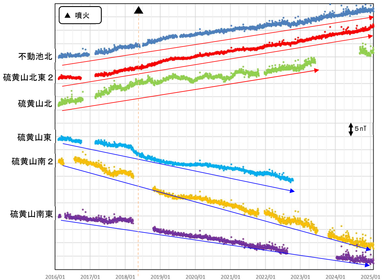
図 6-2 霧島山（えびの高原（硫黄山）周辺） 全磁力観測点で観測された全磁力変動 （2016 年 1 月～2025 年 1 月）
