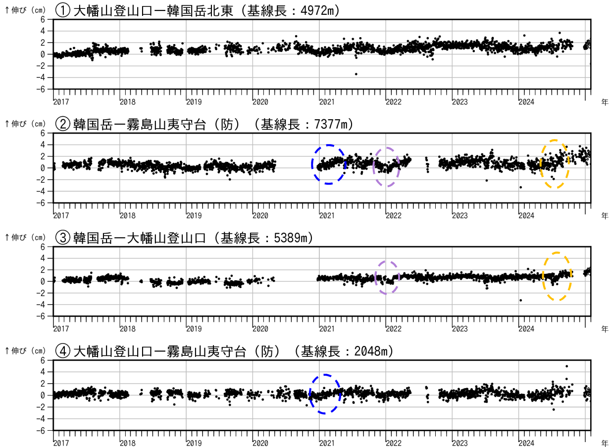
図4 霧島山（大幡池） GNSS 連続観測による基線長変化（2017年1月～2025年1月）
