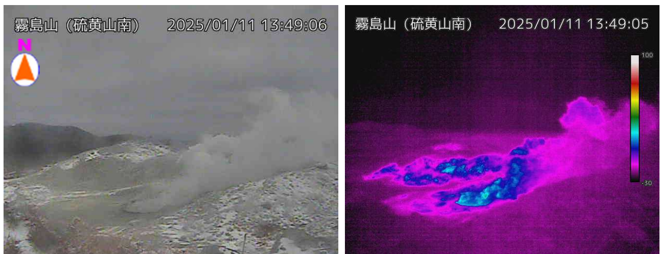
図 1-2 霧島山（えびの高原（硫黄山）周辺） 硫黄山南側の状況（1 月 11 日、硫黄山南監視カメラ）
