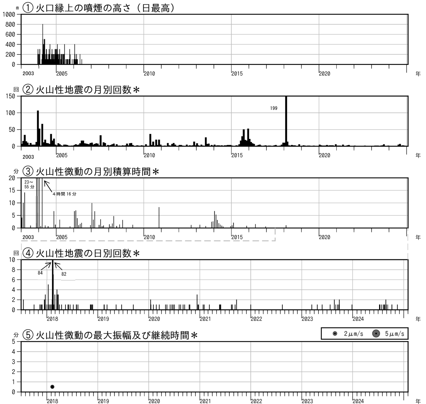
図3 霧島山（御鉢） 火山活動経過図（2003年1月～2025年1月）
