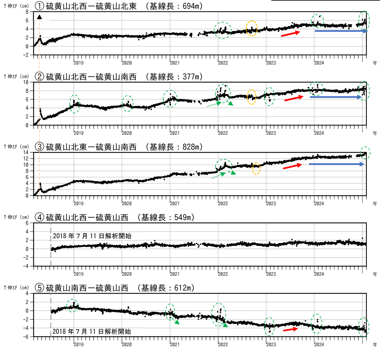
図4 霧島山（えびの高原（硫黄山）周辺） GNSS 連続観測による基線長変化（2018年3月～2025年1月）
