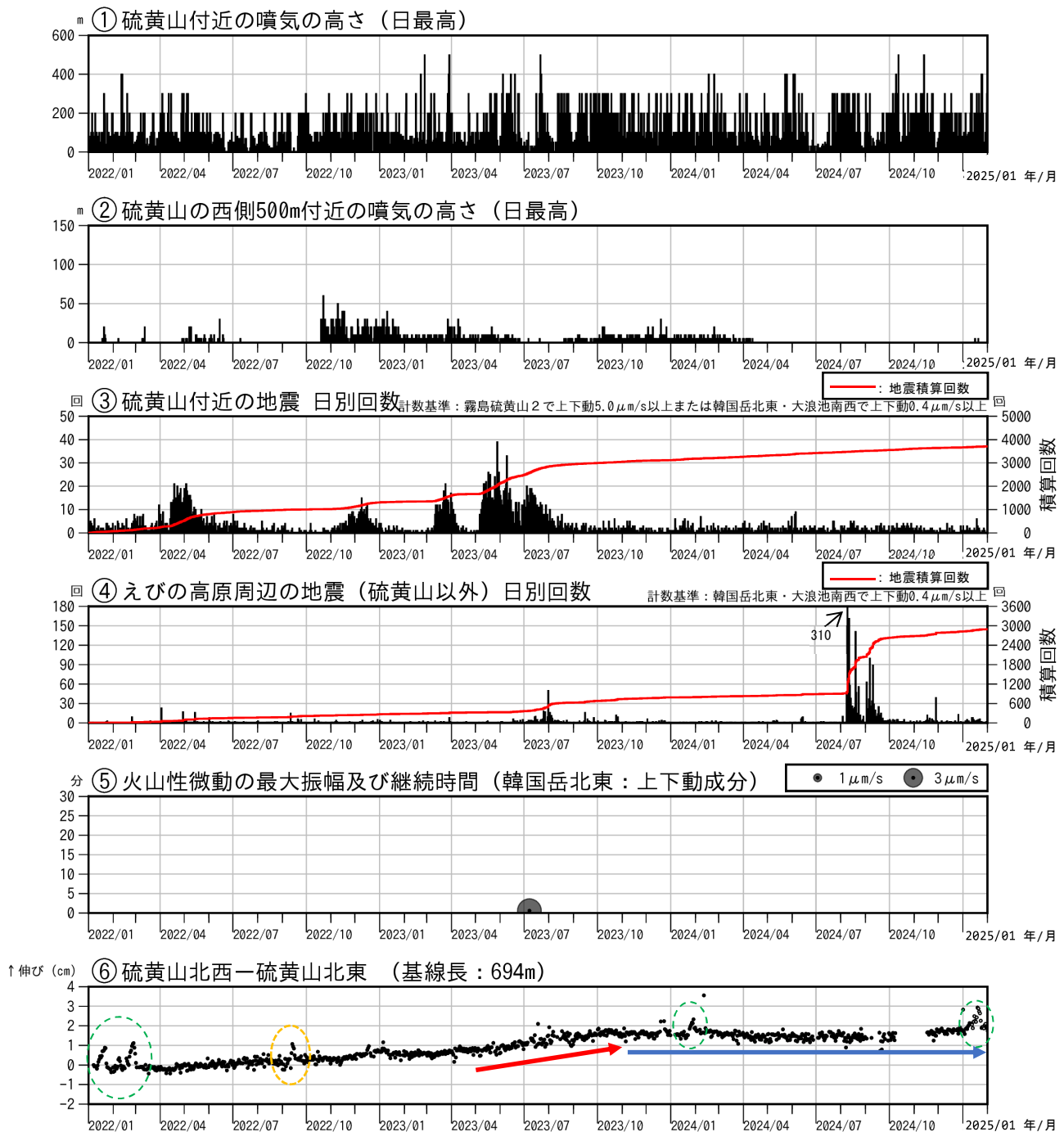
図2 霧島山（えびの高原（硫黄山）周辺） 火山活動経過図（2022年1月～2025年1月）
