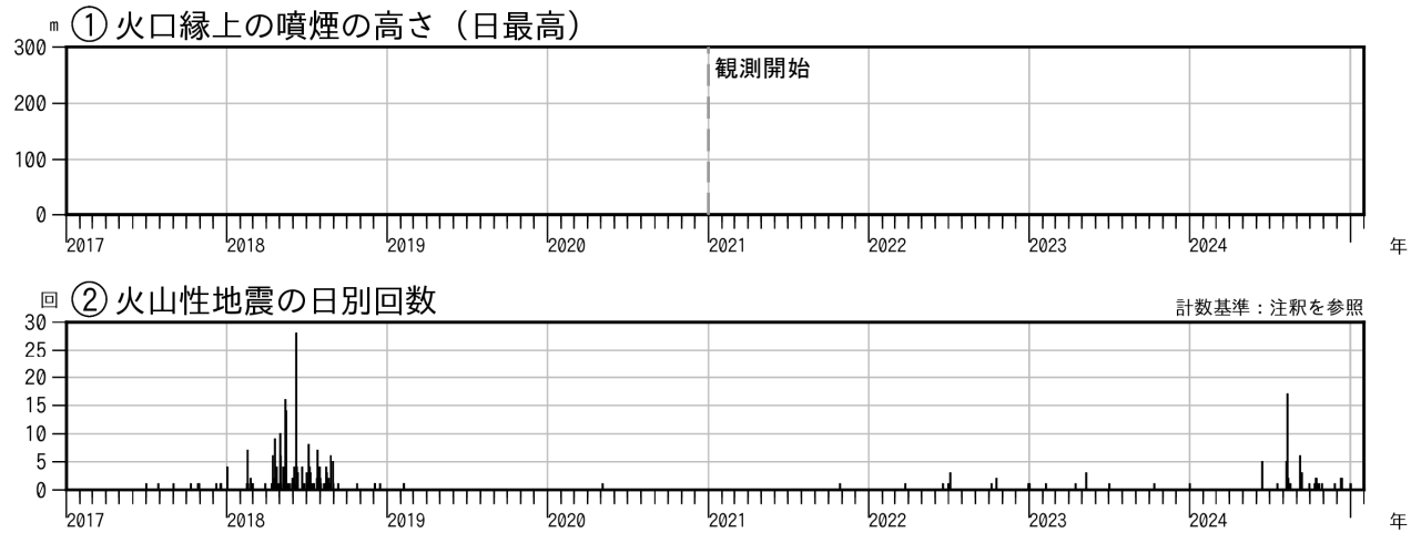
図2 霧島山（大幡池） 火山活動経過図（2017年1月～2025年1月）
