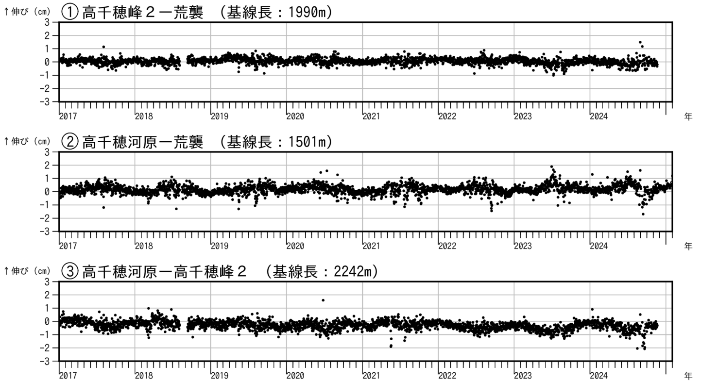
図4 霧島山（御鉢） GNSS 連続観測による基線長変化（2017年1月～2025年1月）
