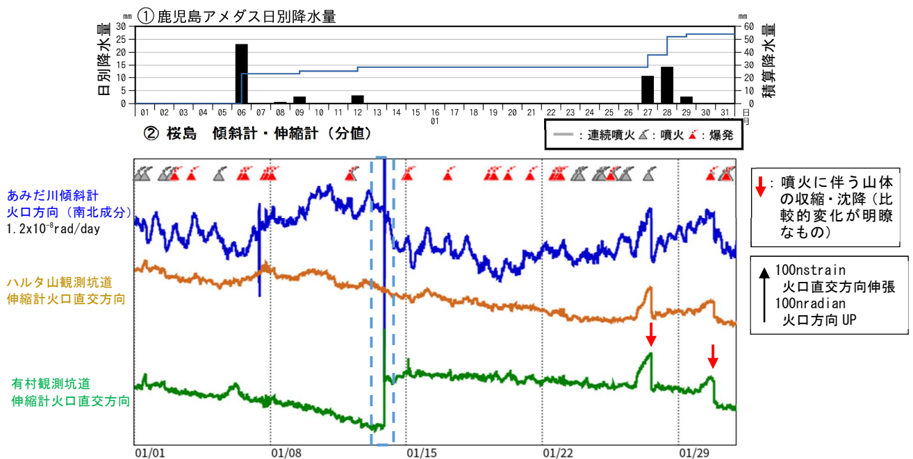
図8 桜島 傾斜計及び伸縮計による地殻変動の状況（2025年1月1日～1月31日）
