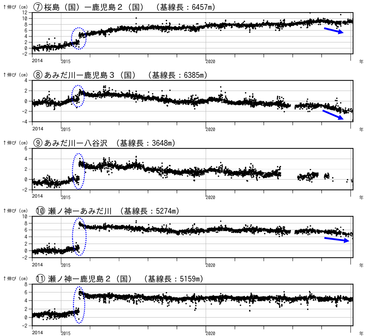
図 9-2 桜島 GNSS 連続観測による基線長変化（2014 年 1 月～2025 年 1 月）
