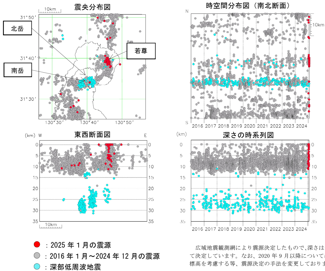
図 4-1 桜島 始良カルデラ周辺の震源分布図（2016 年 1 月～2025 年 1 月）
