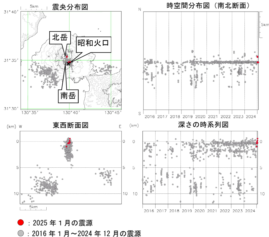
図 4-2 桜島 桜島付近の震源分布図（2016 年 1 月～2025 年 1 月）
