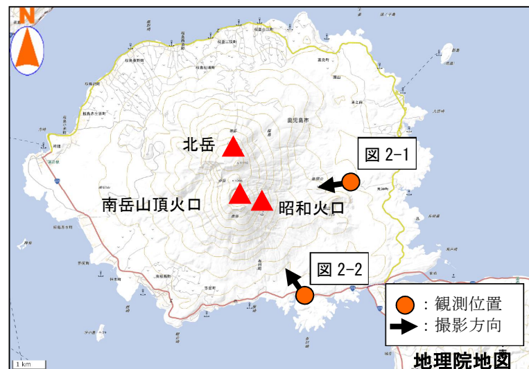
図1 桜島 図2の観測位置及び撮影方向
