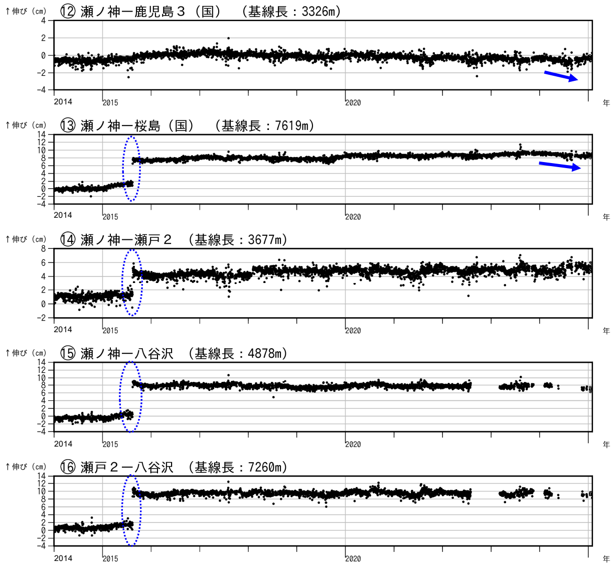
図 9-3 桜島 GNSS 連続観測による基線長変化（2014 年 1 月～2025 年 1 月）
