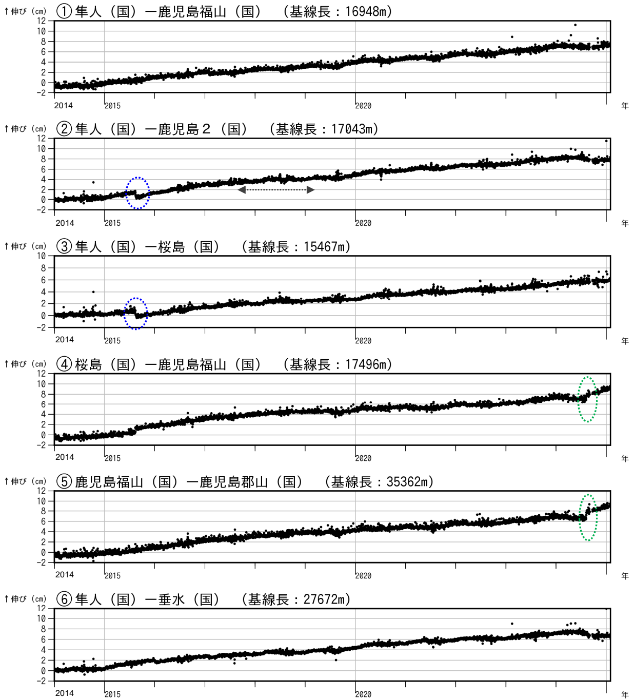
図 9-1 桜島 GNSS 連続観測による基線長変化（2014 年 1 月～2025 年 1 月）
