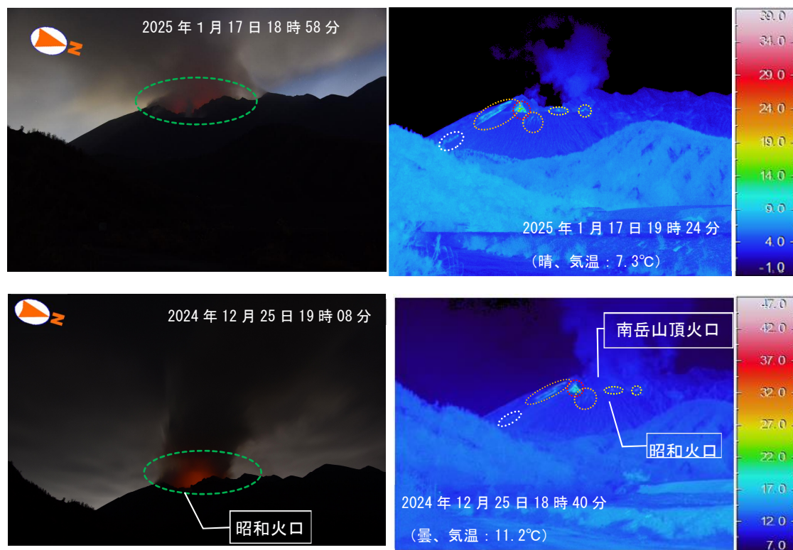
図 2-1 桜島 南岳山頂火口及び昭和火口周辺の状況（黒神町（黒神河原）から観測）
