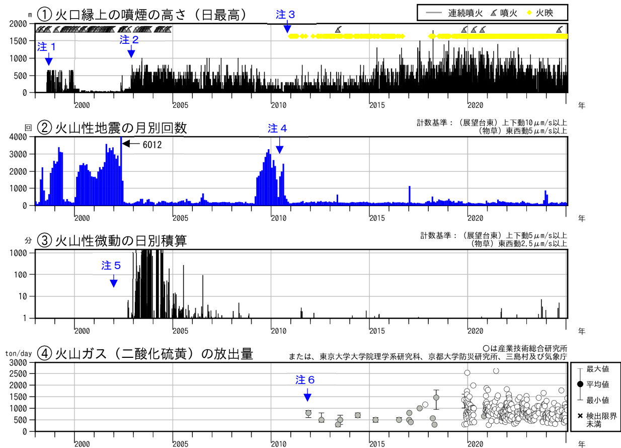
図2 薩摩硫黄島 火山活動経過図（1998年1月～2025年1月）
