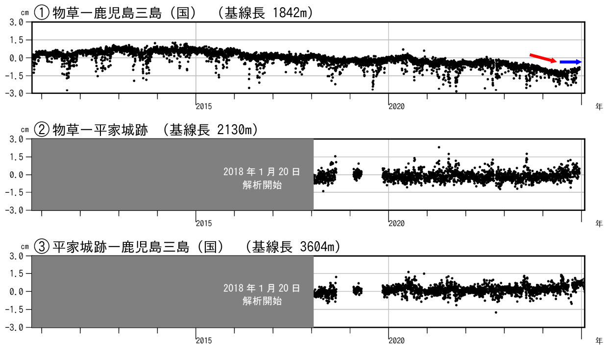
図4 薩摩硫黄島 GNSS連続観測による基線長変化（2010年10月～2025年1月）
