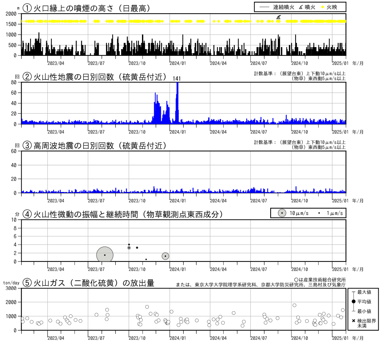
図3 薩摩硫黄島 火山活動経過図（2023年2月～2025年1月）
