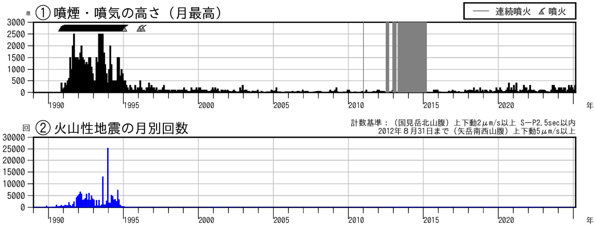
図2 雲仙岳 長期の火山活動経過図（1989年1月～2025年2月）
