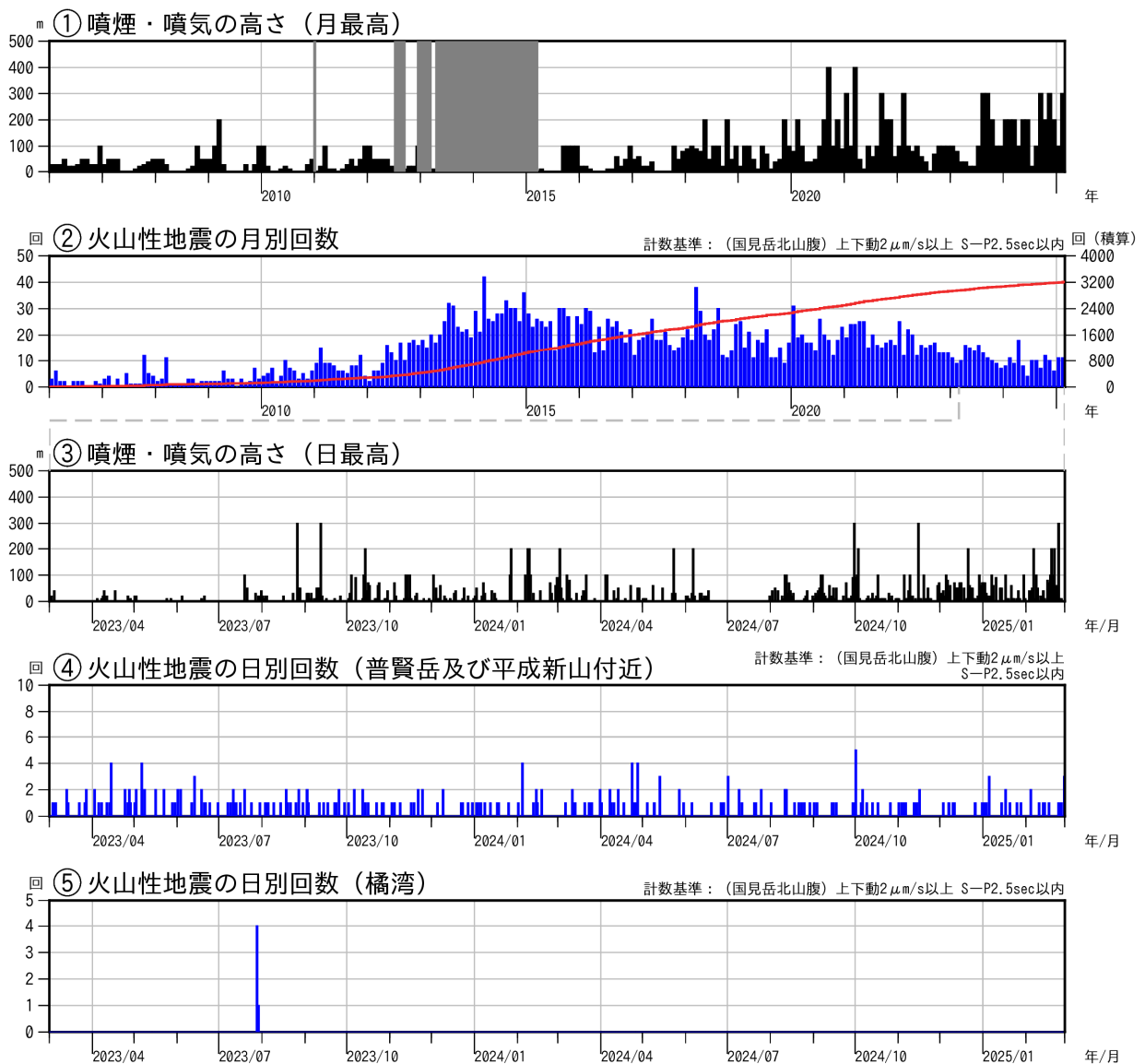
図3 雲仙岳 火山活動経過図（2006年1月～2025年2月）
