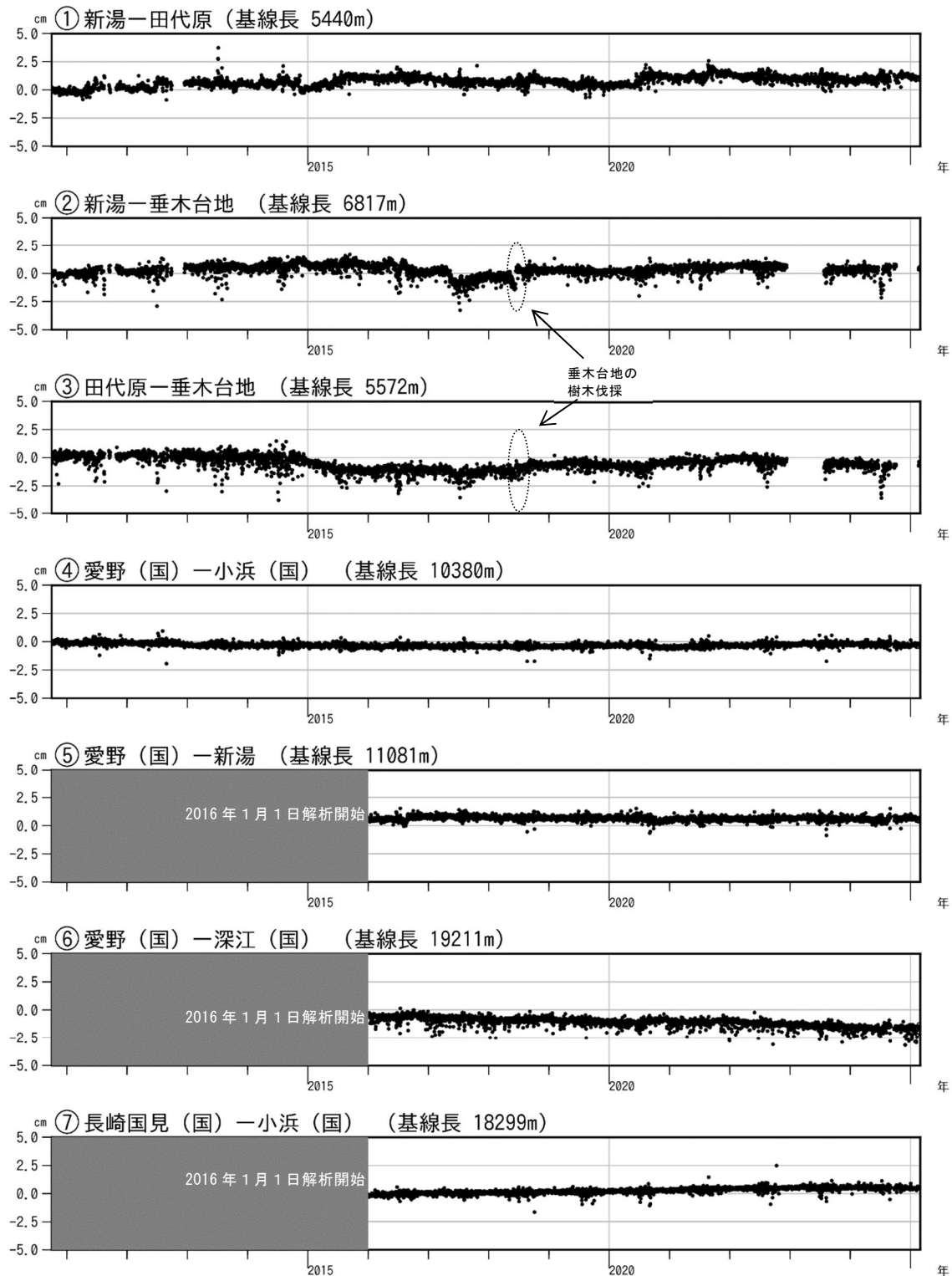
図5 雲仙岳 GNSS連続観測による基線長変化（2010年10月～2025年2月）
