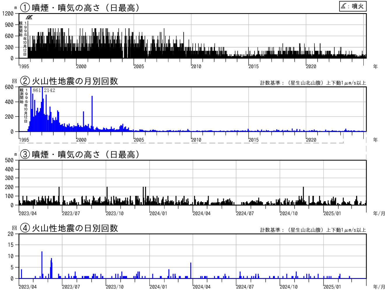
図3 九重山 火山活動経過図（1995年1月～2025年3月）
