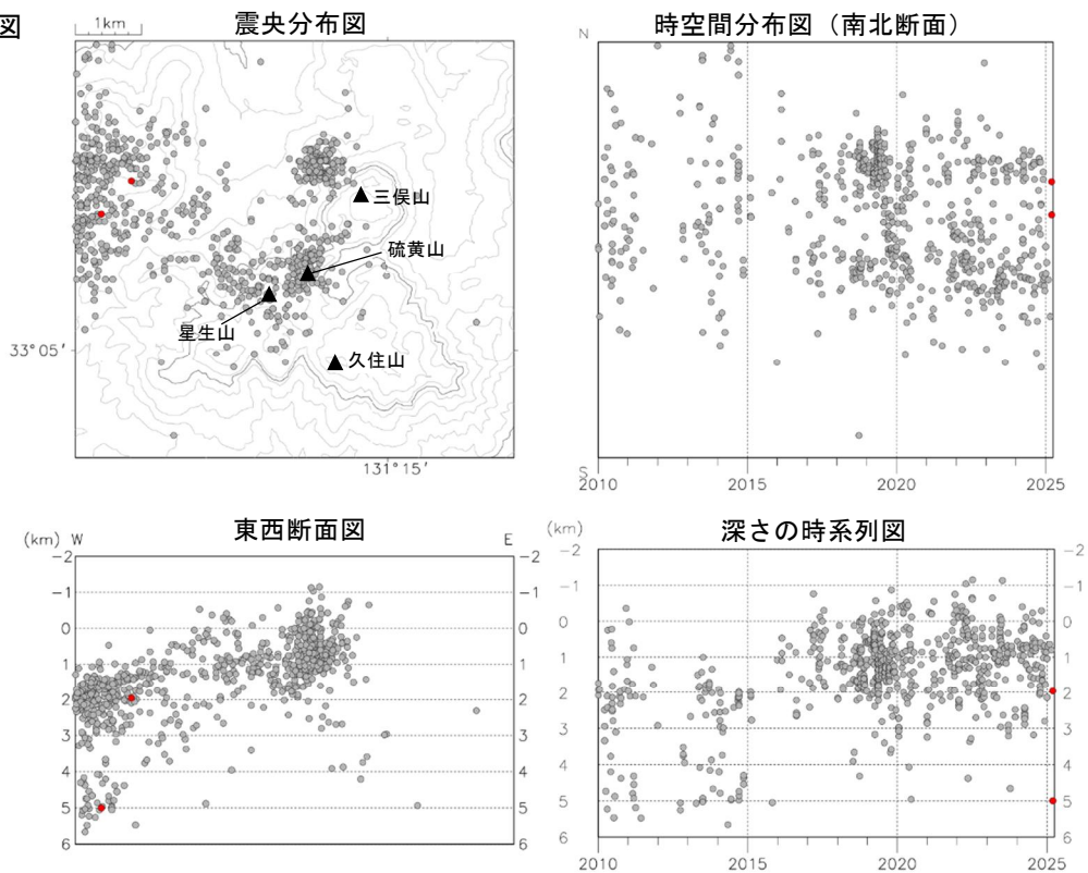
図 4 九重山 震源分布図 ①広域図 ②狭域図（2010 年 1 月～2025 年 3 月）
