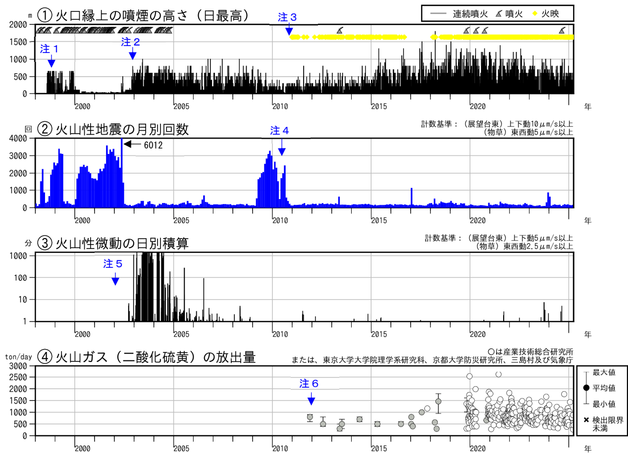
図3 薩摩硫黄島 火山活動経過図（1998年1月～2025年3月）
