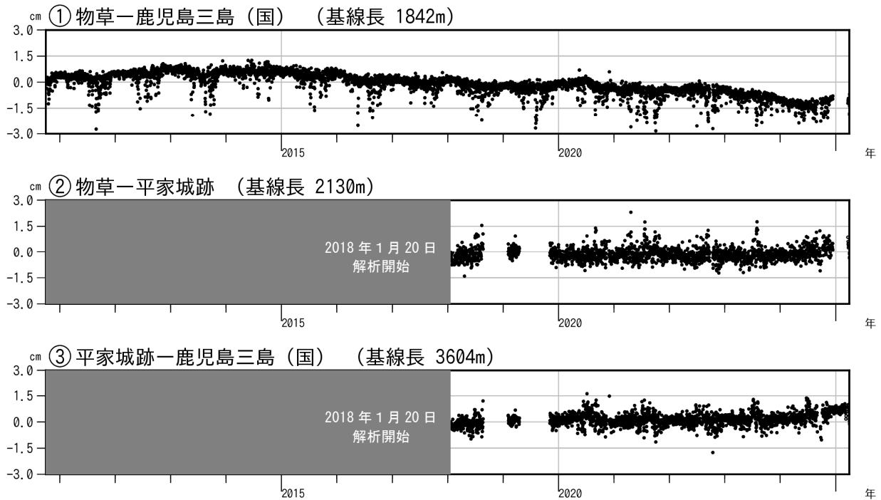
図6 薩摩硫黄島 GNSS連続観測による基線長変化（2010年10月～2025年3月）
