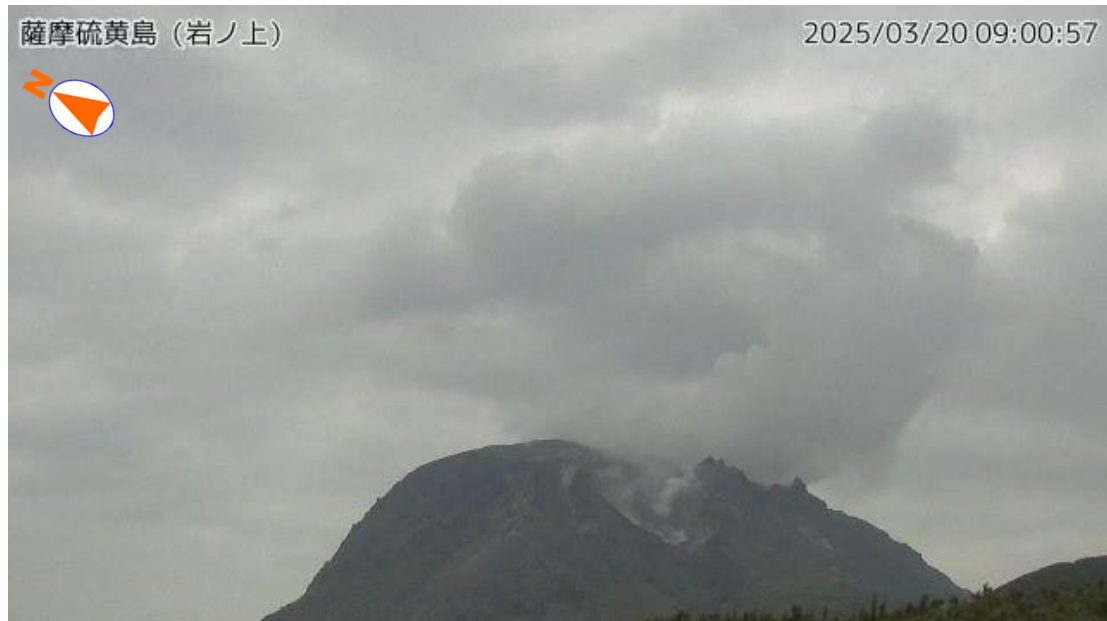
図1-1 薩摩硫黄島 噴煙の状況（3月20日 岩ノ上監視カメラ）
