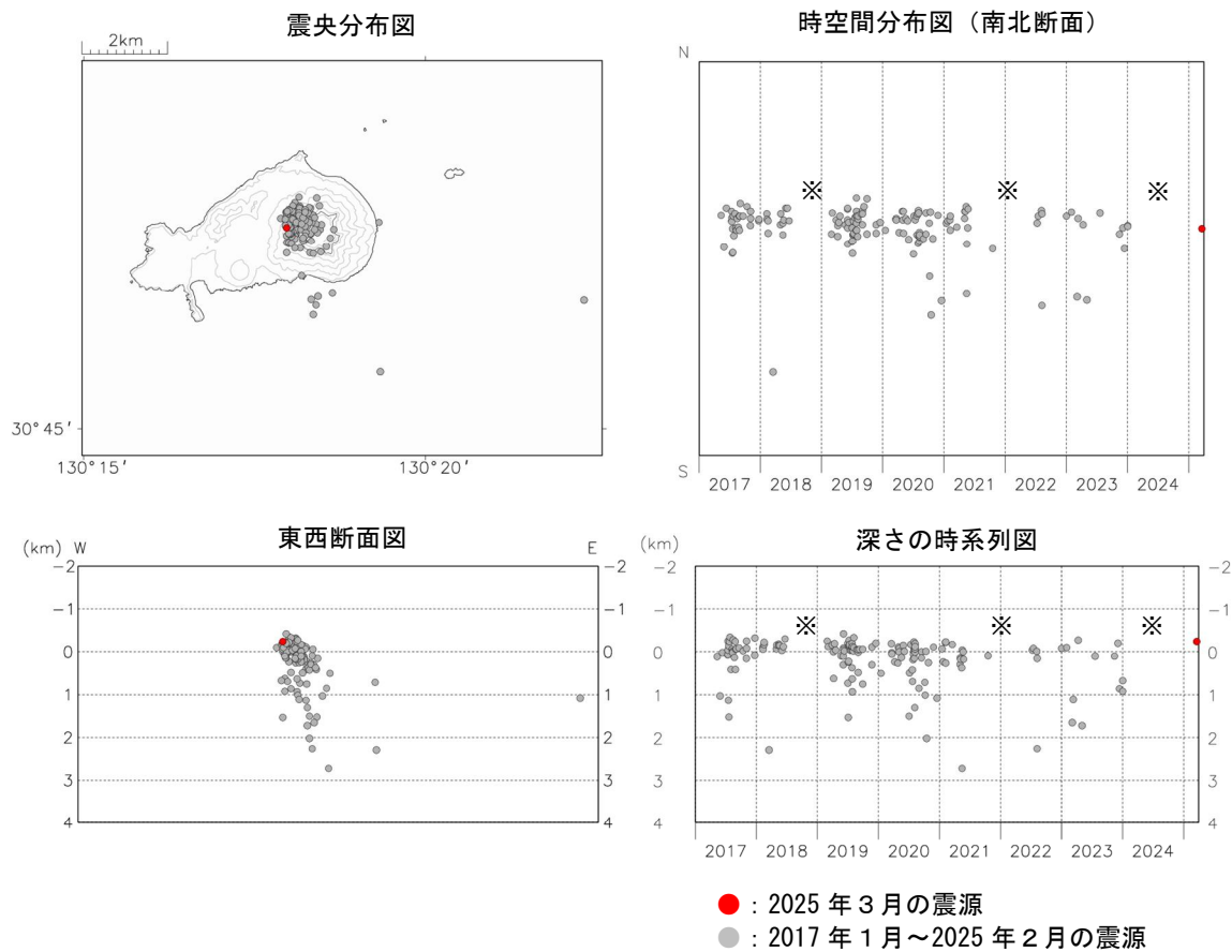
図5 薩摩硫黄島 火山性地震の震源分布図（2017 年 1 月～2025 年 3 月）
