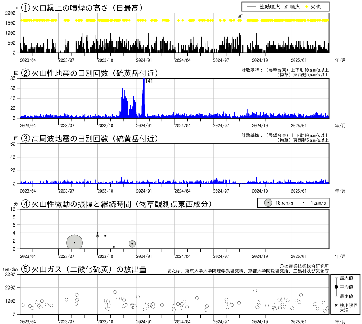
図4 薩摩硫黄島 火山活動経過図（2023年4月～2025年3月）
