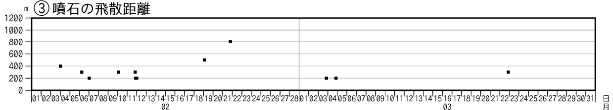
図5 諏訪之瀬島 ナベタオ観測点の傾斜変動と噴火活動（2025年2月～3月）
