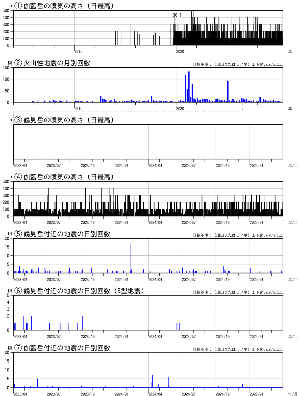
図2 鶴見岳・伽藍岳 火山活動経過図（2012年1月～2025年3月）
