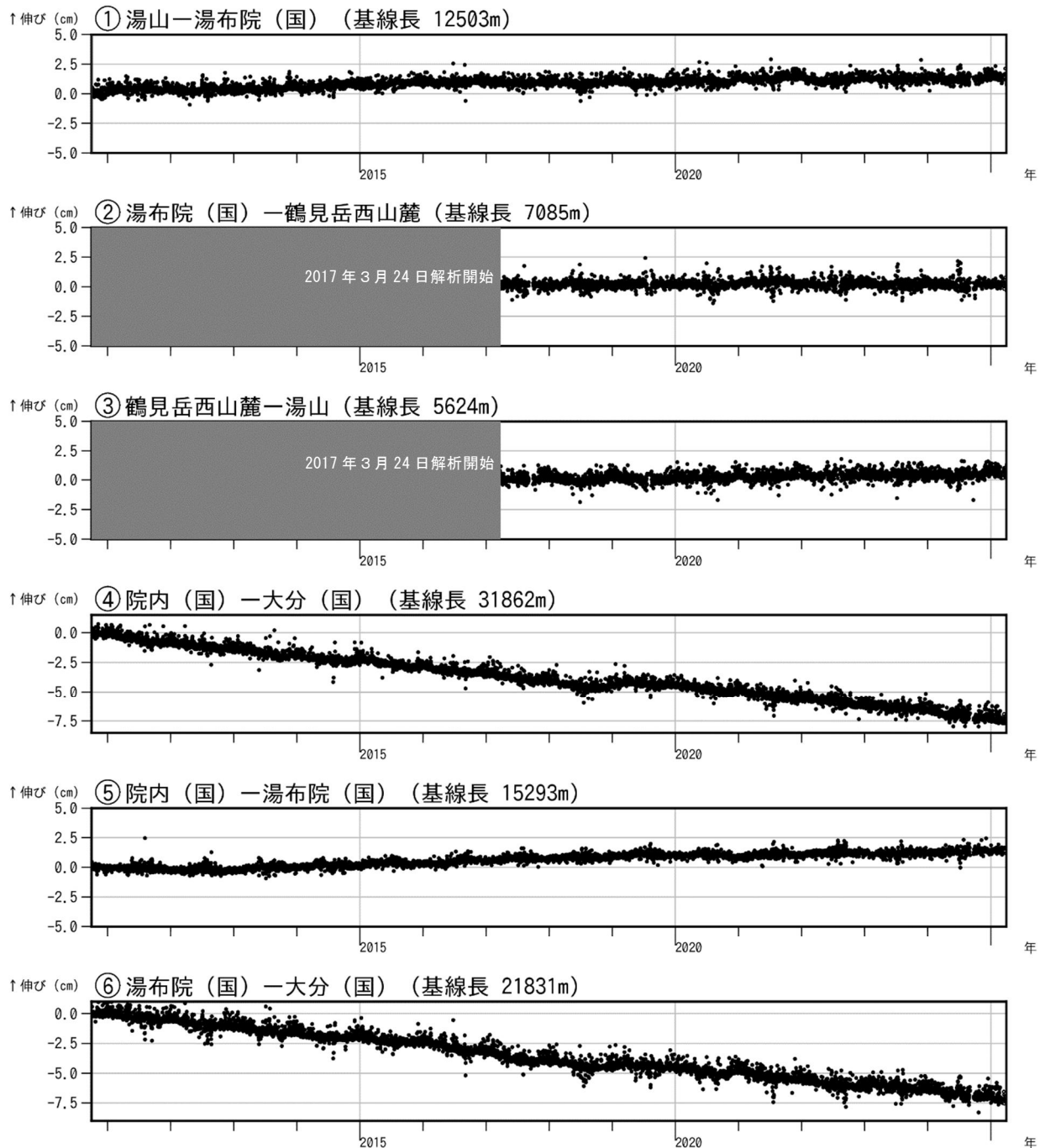
図4 鶴見岳・伽藍岳 GNSS連続観測による基線長変化（2010年10月～2025年3月）
