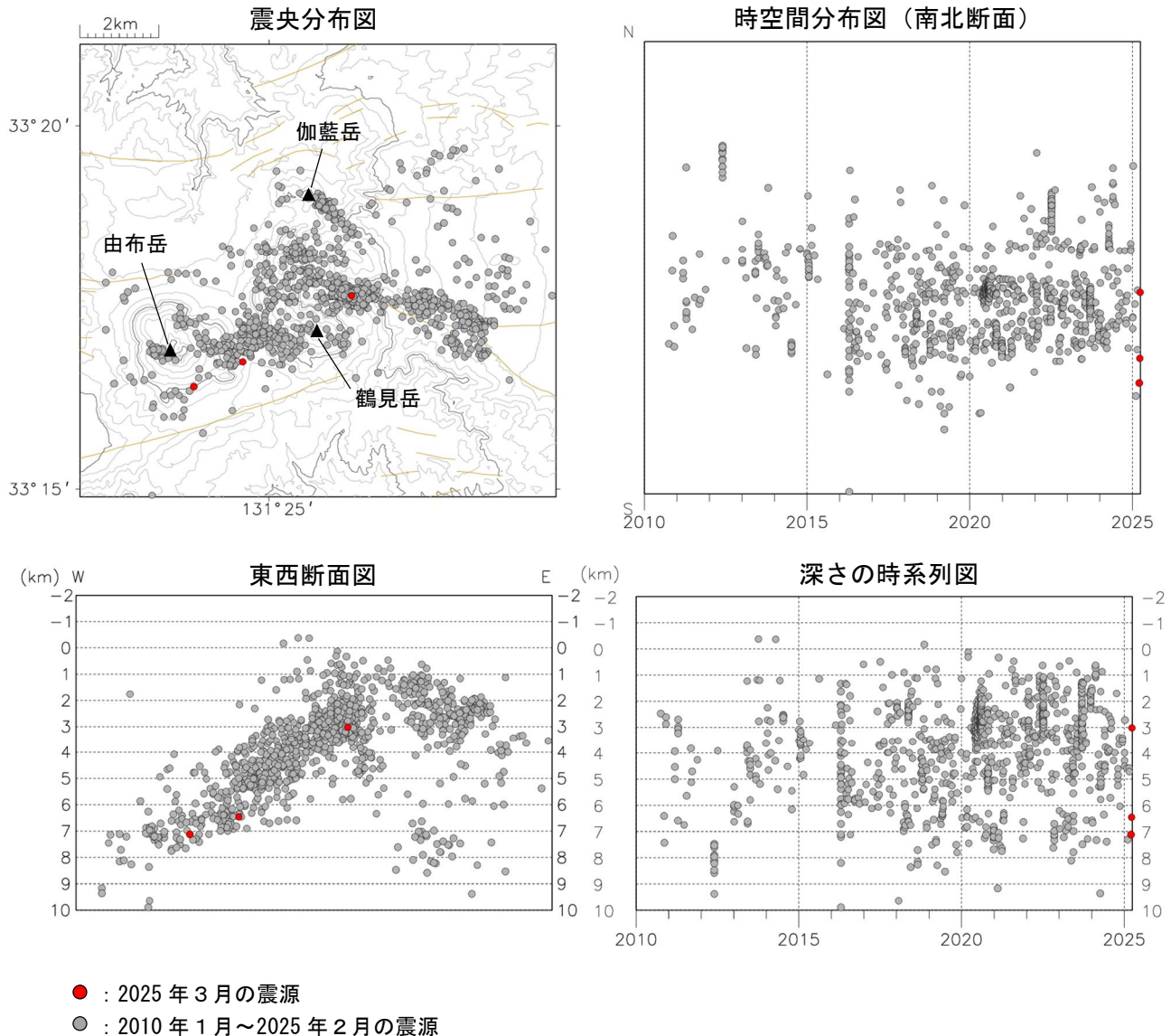
図3 鶴見岳・伽藍岳 震源分布図（2010年1月～2025年3月）
