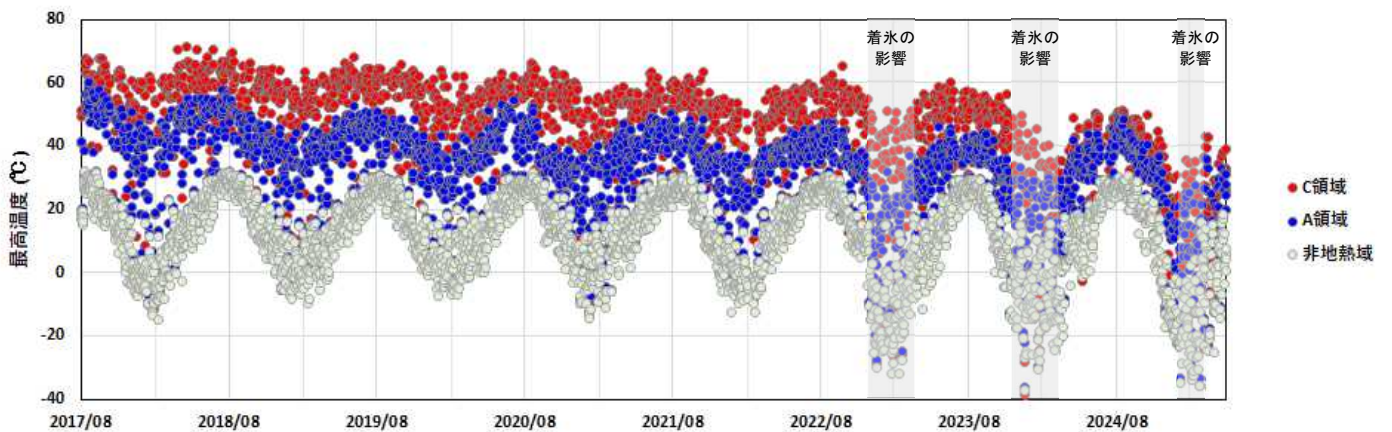
図 1-2 九重山 星生山北尾根の赤外熱映像装置による日別最高温度（2017 年 8 月～2025 年 4 月）
