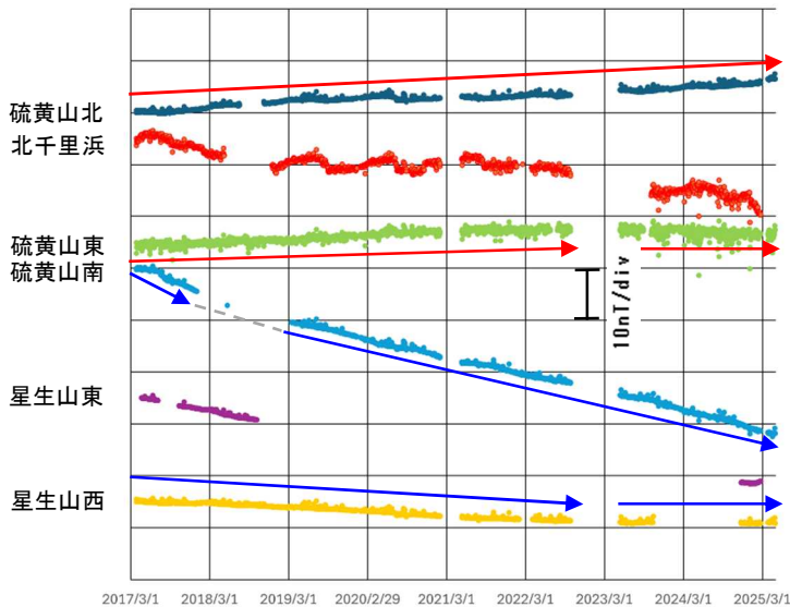
図 4-1 九重山 連続観測による全磁力の変化 (2017年3月～2025年4月)
