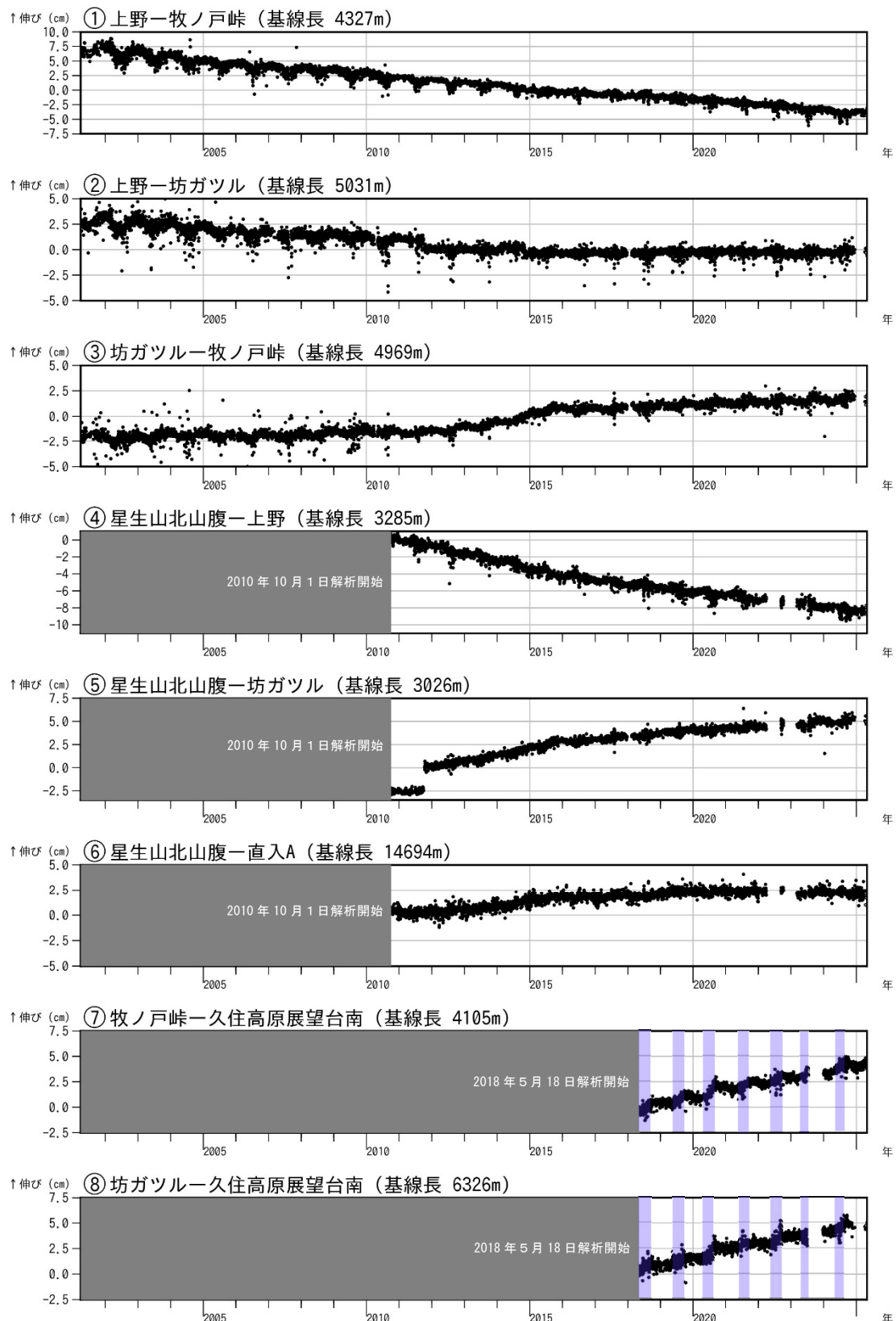
図5 九重山 GNSS 連続観測による基線長変化（2001年4月～2025年4月）
