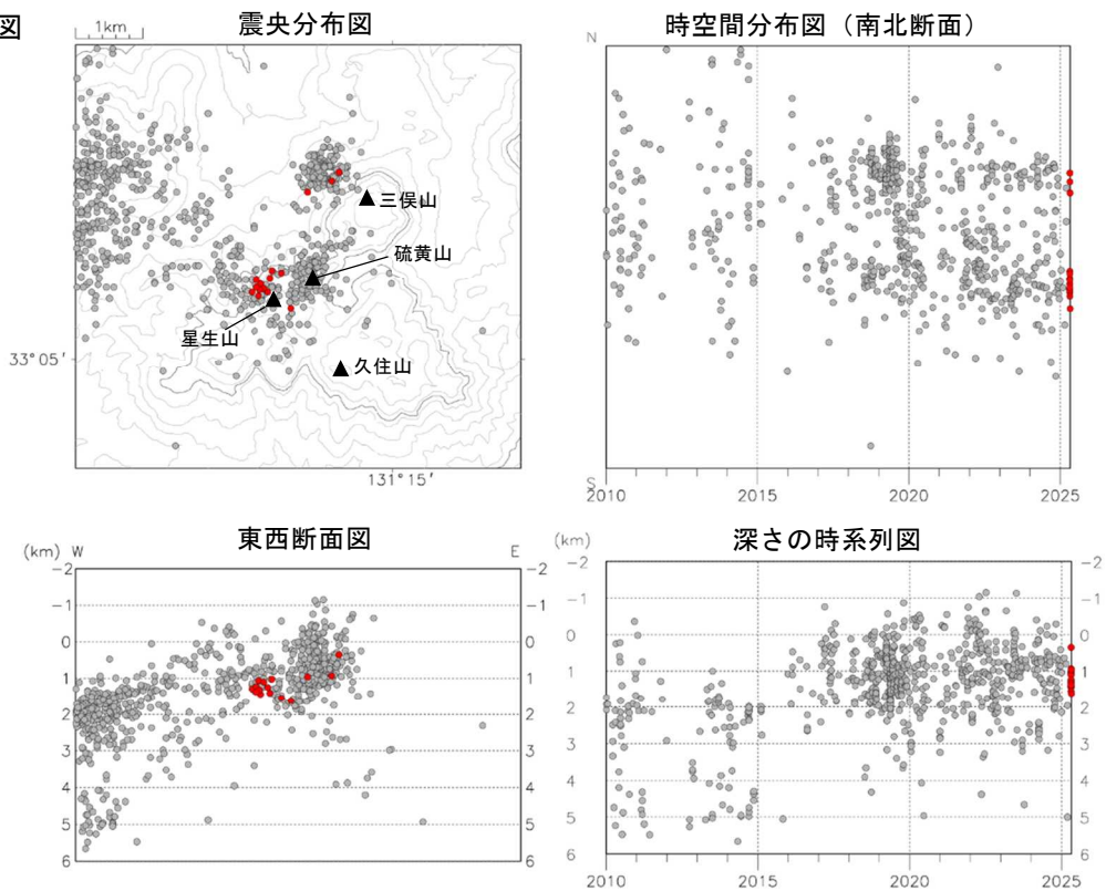
図 3 九重山 震源分布図 ①広域図 ②狭域図（2010 年 1 月～2025 年 4 月）
