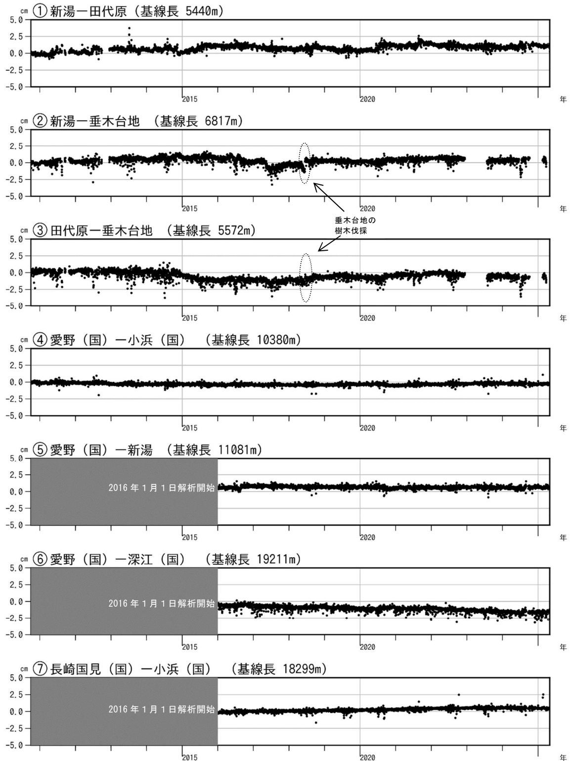
図5 雲仙岳 GNSS連続観測による基線長変化（2010年10月～2025年4月）
