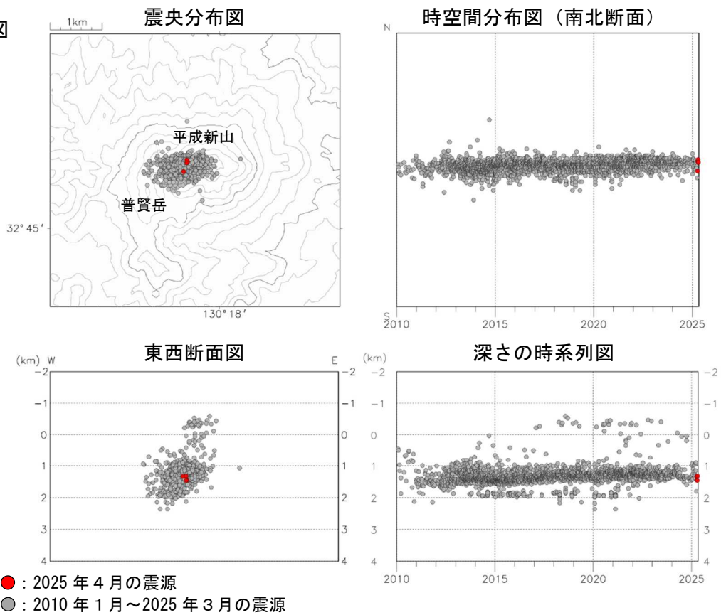
図4 雲仙岳 震源分布図 ①広域図 ②狭域図（2010年1月～2025年4月）
