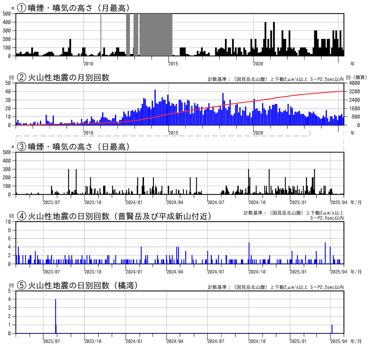
図3 雲仙岳 火山活動経過図（2006年1月～2025年4月）
