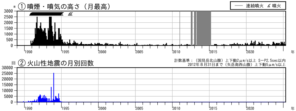
図2 雲仙岳 長期の火山活動経過図（1989年1月～2025年4月）
