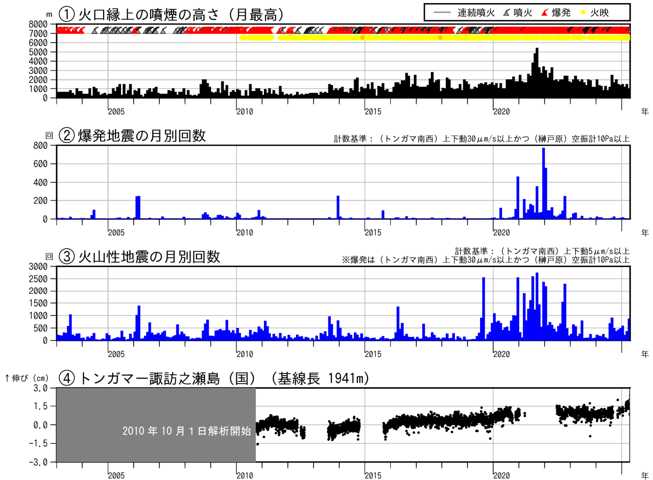
図2 諏訪之瀬島 長期の火山活動経過図（2003年1月～2025年4月）
