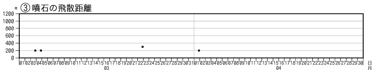
図5 諏訪之瀬島 ナベタオ観測点の傾斜変動と噴火活動（2025年3月～4月）
