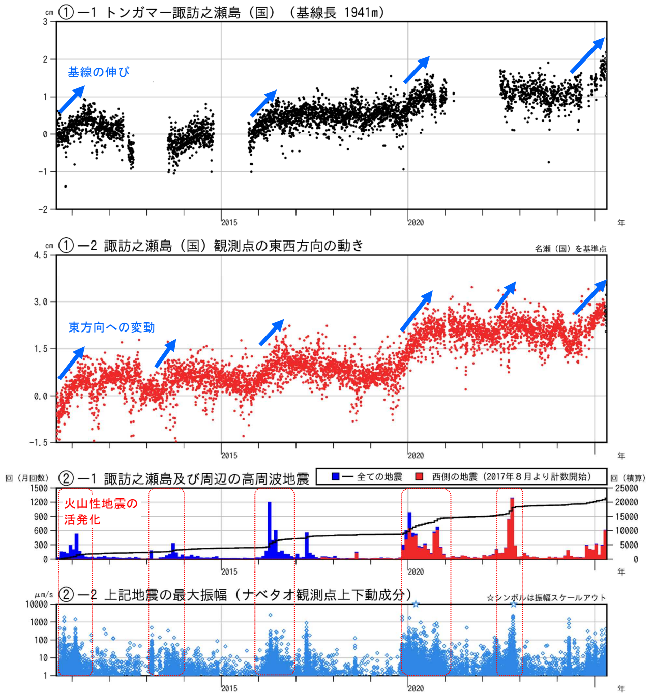
図6 諏訪之瀬島 GNSS連続観測と周辺の火山性地震（2010年8月～2025年4月）
