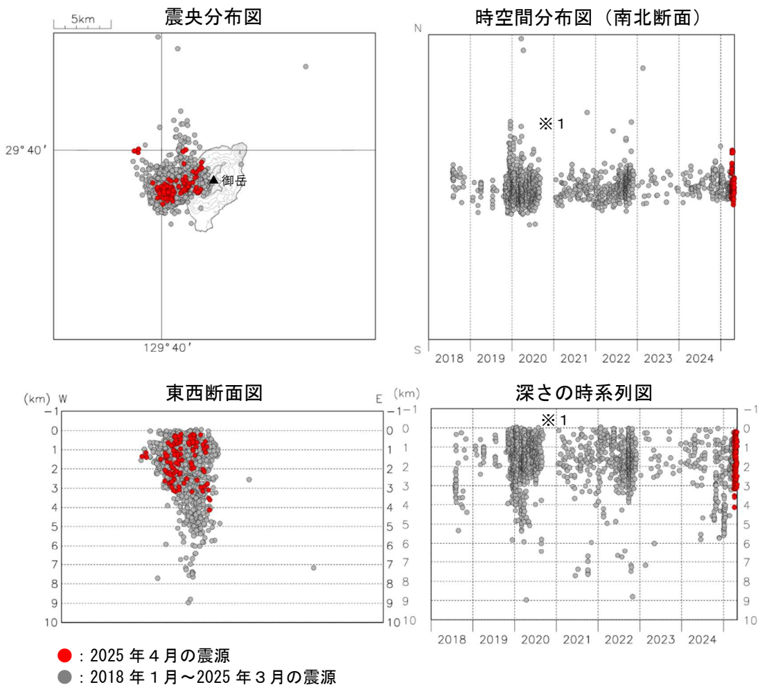
図4 諏訪之瀬島 震源分布図（2018年1月～2025年4月）
