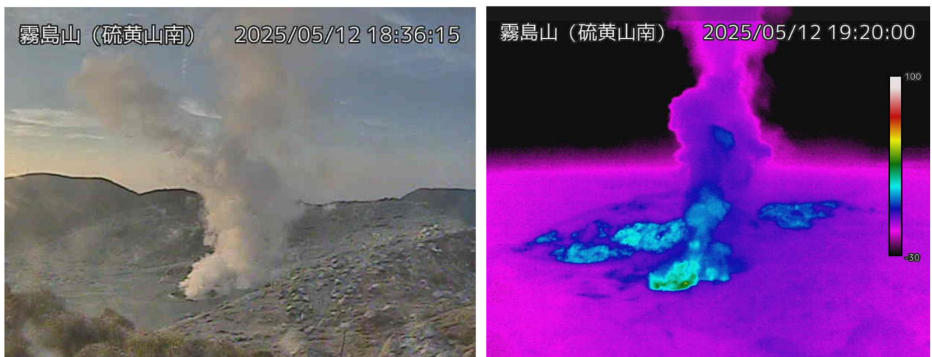
図 1-2 霧島山（えびの高原（硫黄山）周辺） 硫黄山南側の状況（5月12日、硫黄山南監視カメラ）
