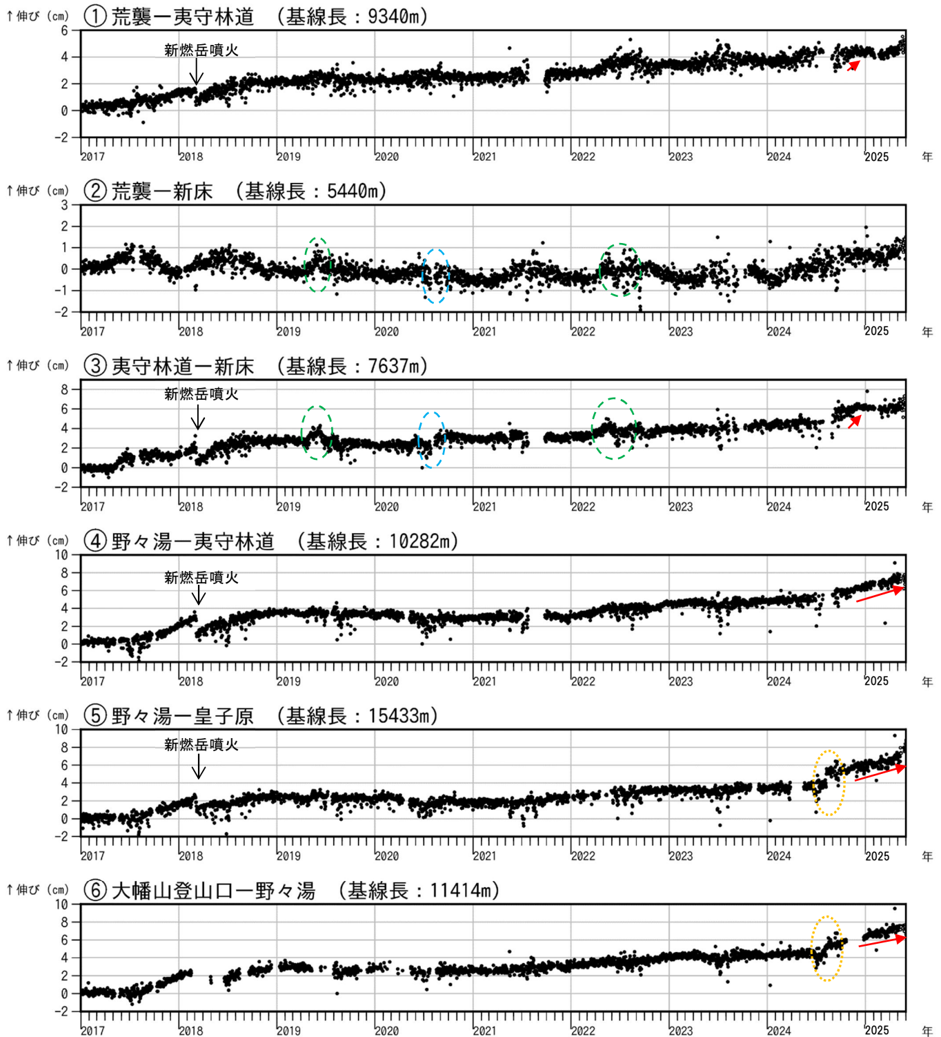
図10 霧島山（新燃岳） GNSS 連続観測による基線長変化（2017年1月～2025年5月）
