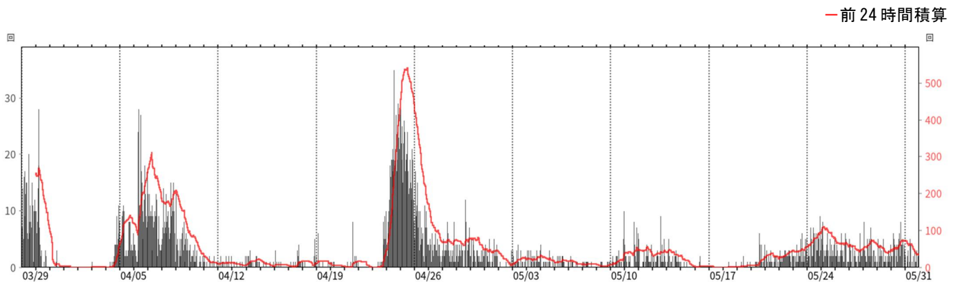
図4 霧島山（新燃岳） 火山性地震の時間別回数及び前24時間積算回数（赤線） (2025年3月29日～5月31日)
