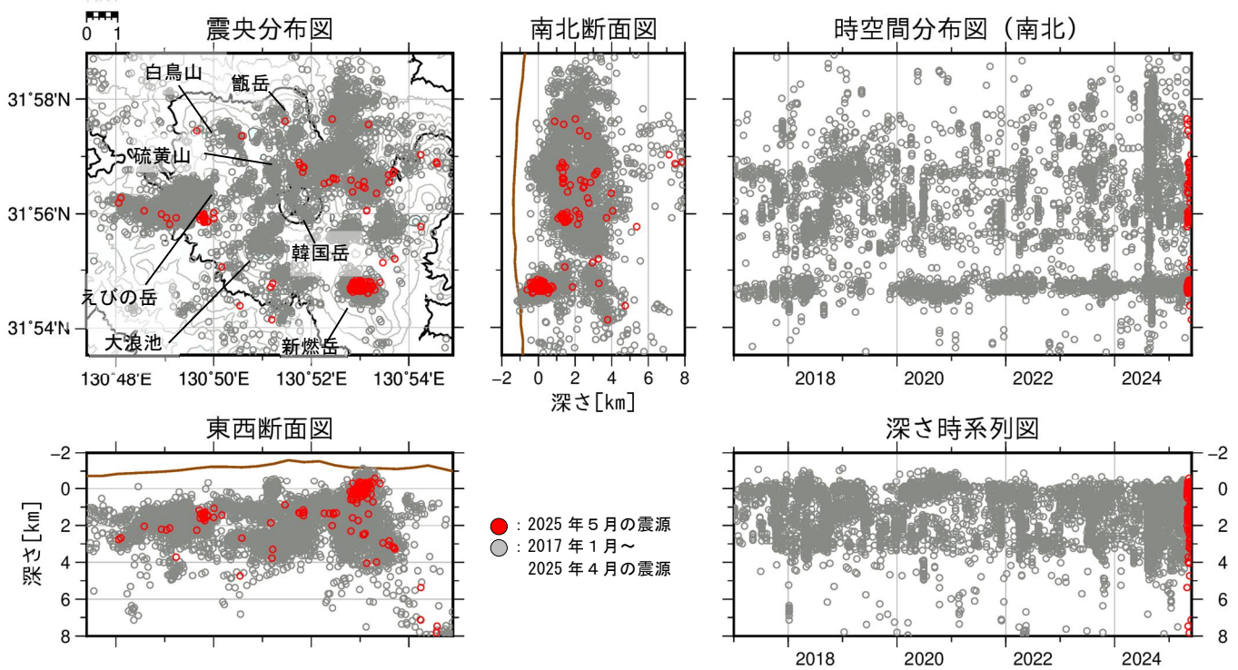
図5 霧島山（えびの高原（硫黄山）周辺） 震源分布図（2017年1月～2025年5月）
