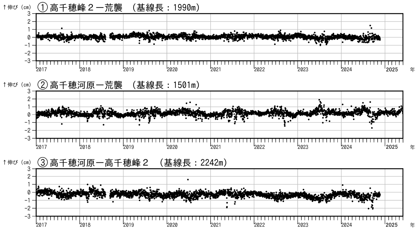
図4 霧島山（御鉢） GNSS 連続観測による基線長変化（2017年1月～2025年5月）
