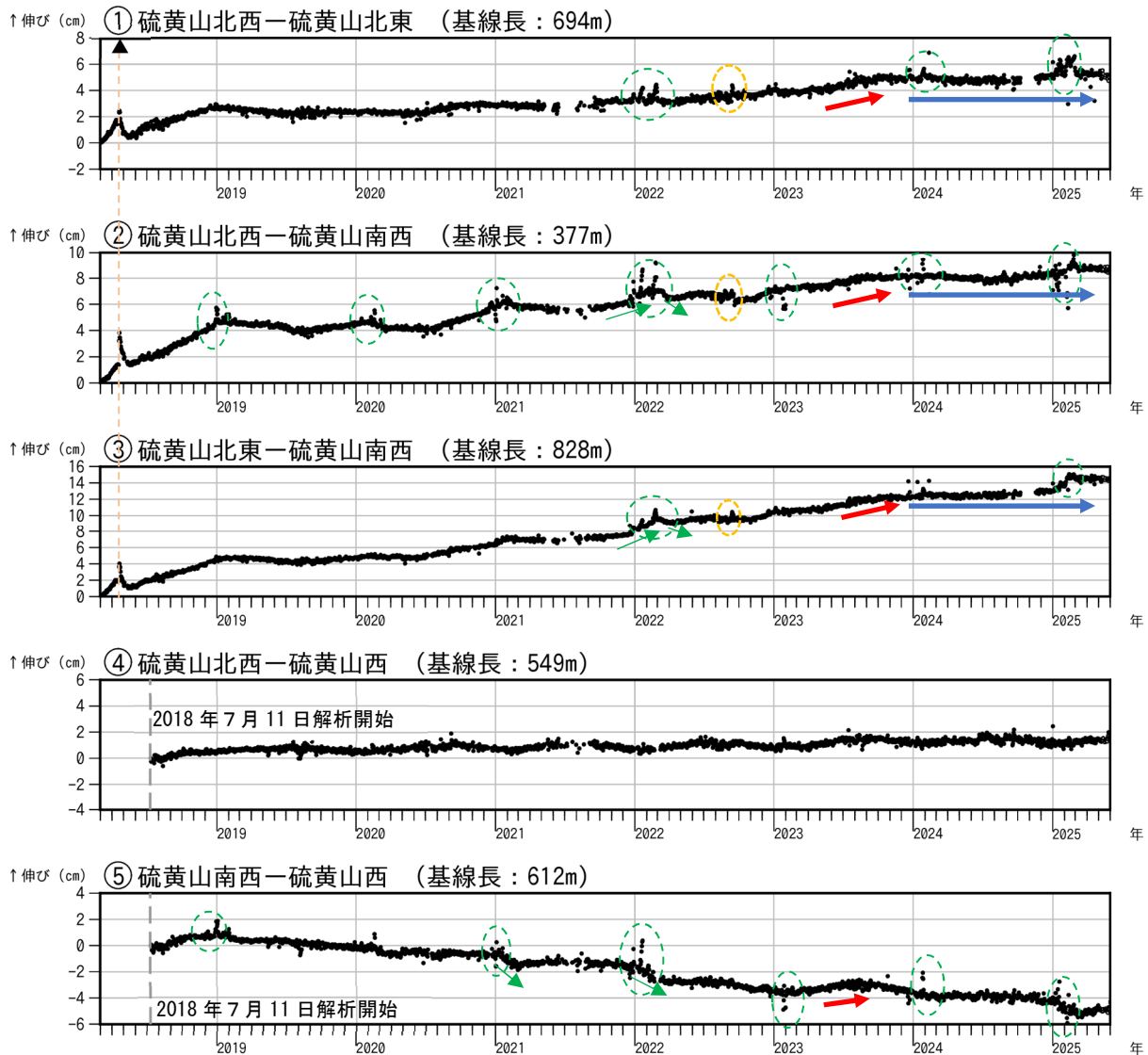
図6 霧島山（えびの高原（硫黄山）周辺） GNSS 連続観測による基線長変化（2018年3月～2025年5月）
