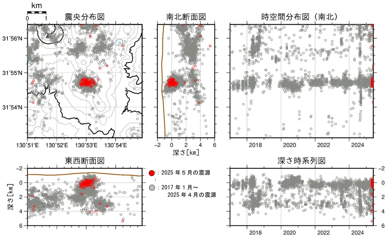
図 8 霧島山（新燃岳） 震源分布図（2017 年 1 月～2025 年 5 月）
