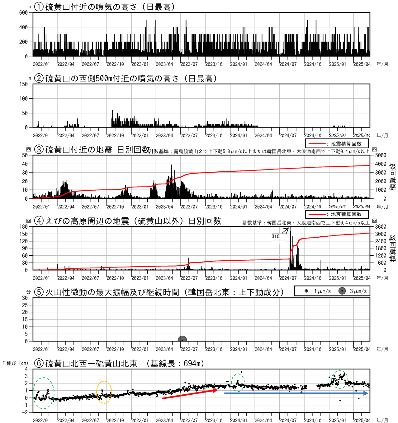
図4 霧島山（えびの高原（硫黄山）周辺）火山活動経過図（2022年1月～2025年5月）
