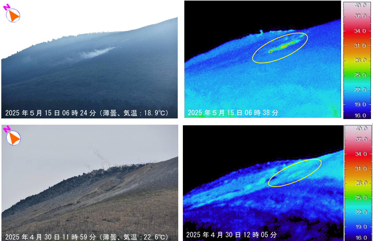
図2 霧島山（新燃岳） 新燃岳西側斜面の割れ目付近の状況（新湯温泉付近からの観測）
