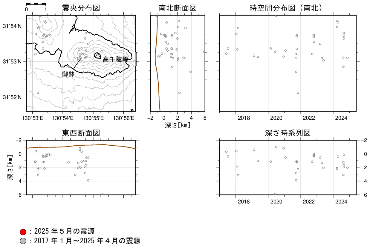
図2 霧島山（御鉢） 震源分布図（2017年1月～2025年5月）
