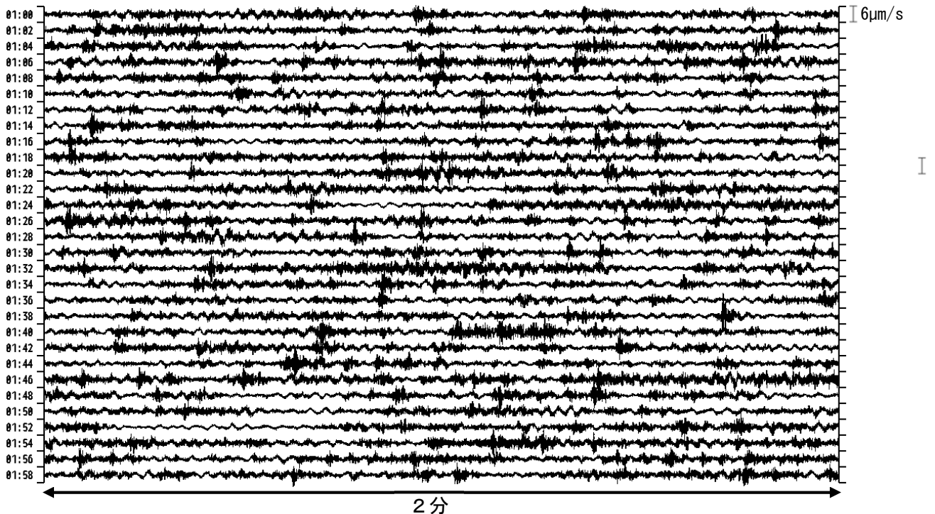
図5 霧島山（新燃岳） 火山性微動の状況（2日01時00分から1時間表示） （新燃西（震）地震計：速度波形南北動成分）
