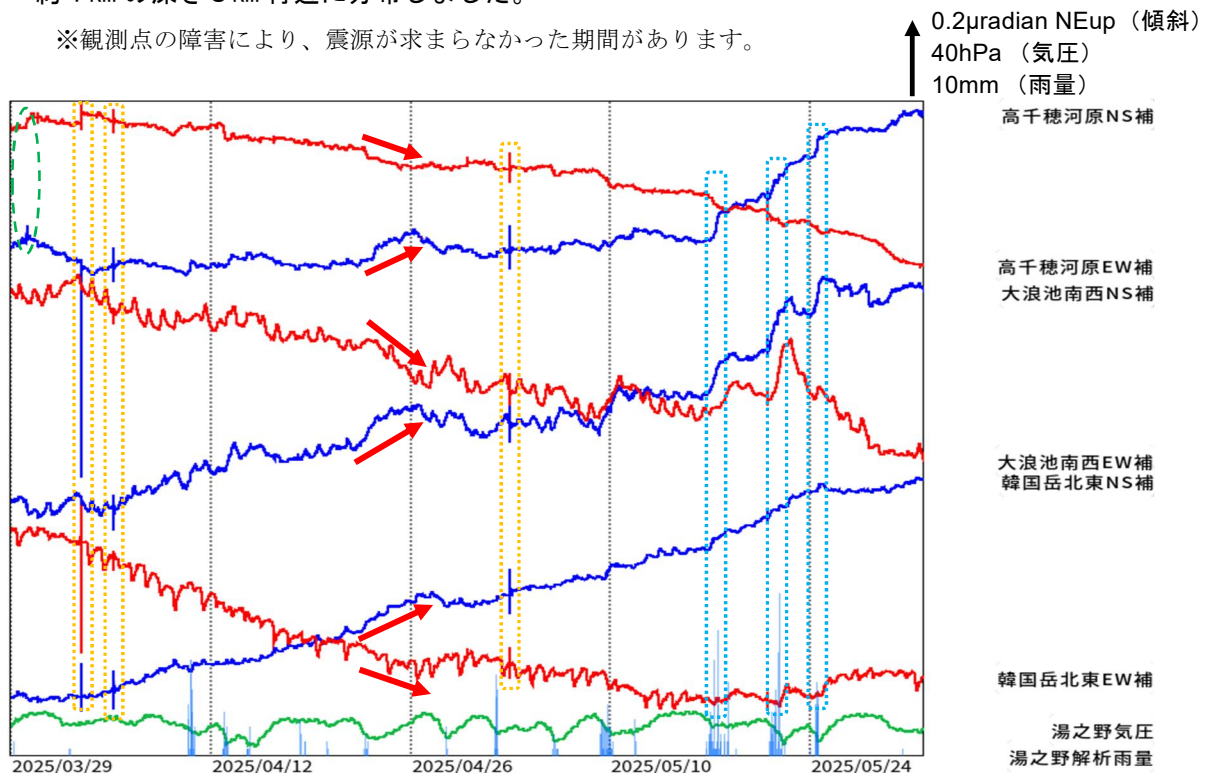
図 9 霧島山（新燃岳） 傾斜計による地殻変動の状況（分値）
