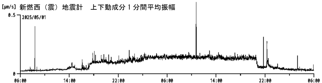
図6 霧島山（新燃岳） 火山性微動発生前後の新燃西（震）地震計の振幅の状況 （1日06時00分～3日06時00分）
