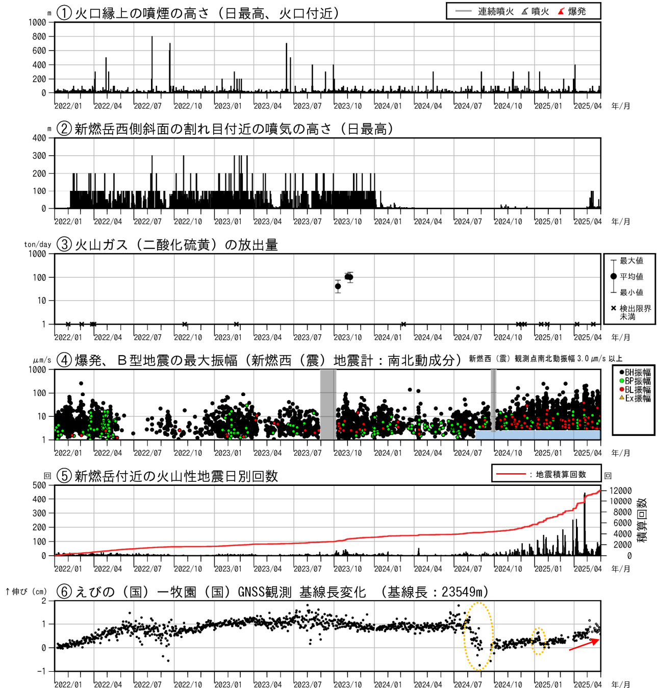
図7 霧島山（新燃岳） 火山活動経過図（2022年1月～2025年5月）
