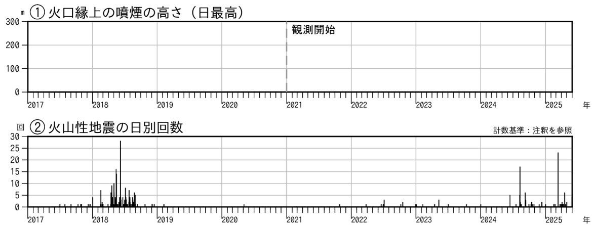
図 2 霧島山（大幡池） 火山活動経過図（2017 年 1 月～2025 年 5 月）
