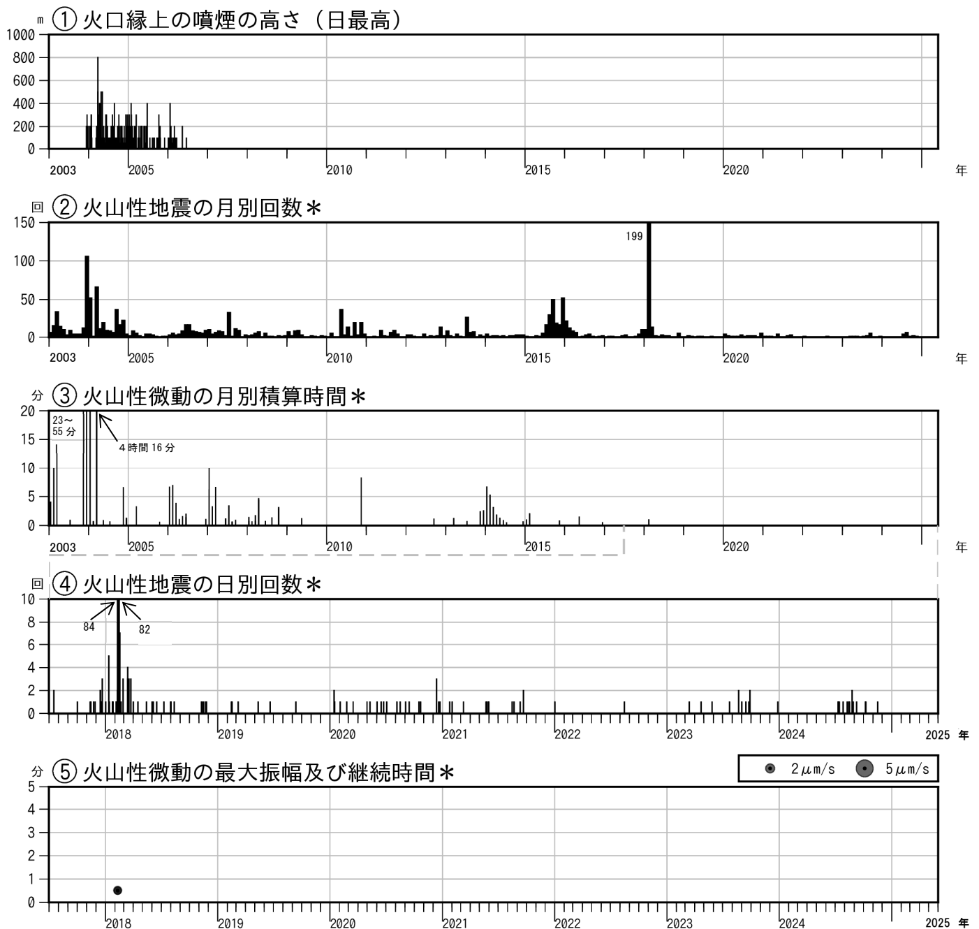
図3 霧島山（御鉢） 火山活動経過図（2003年1月～2025年5月）
