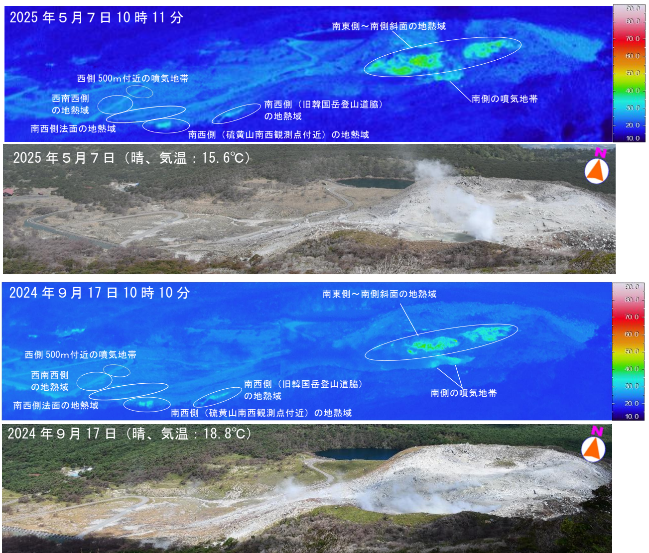
図3 霧島山（えびの高原（硫黄山）周辺） 硫黄山の火口及びその周辺の状況
