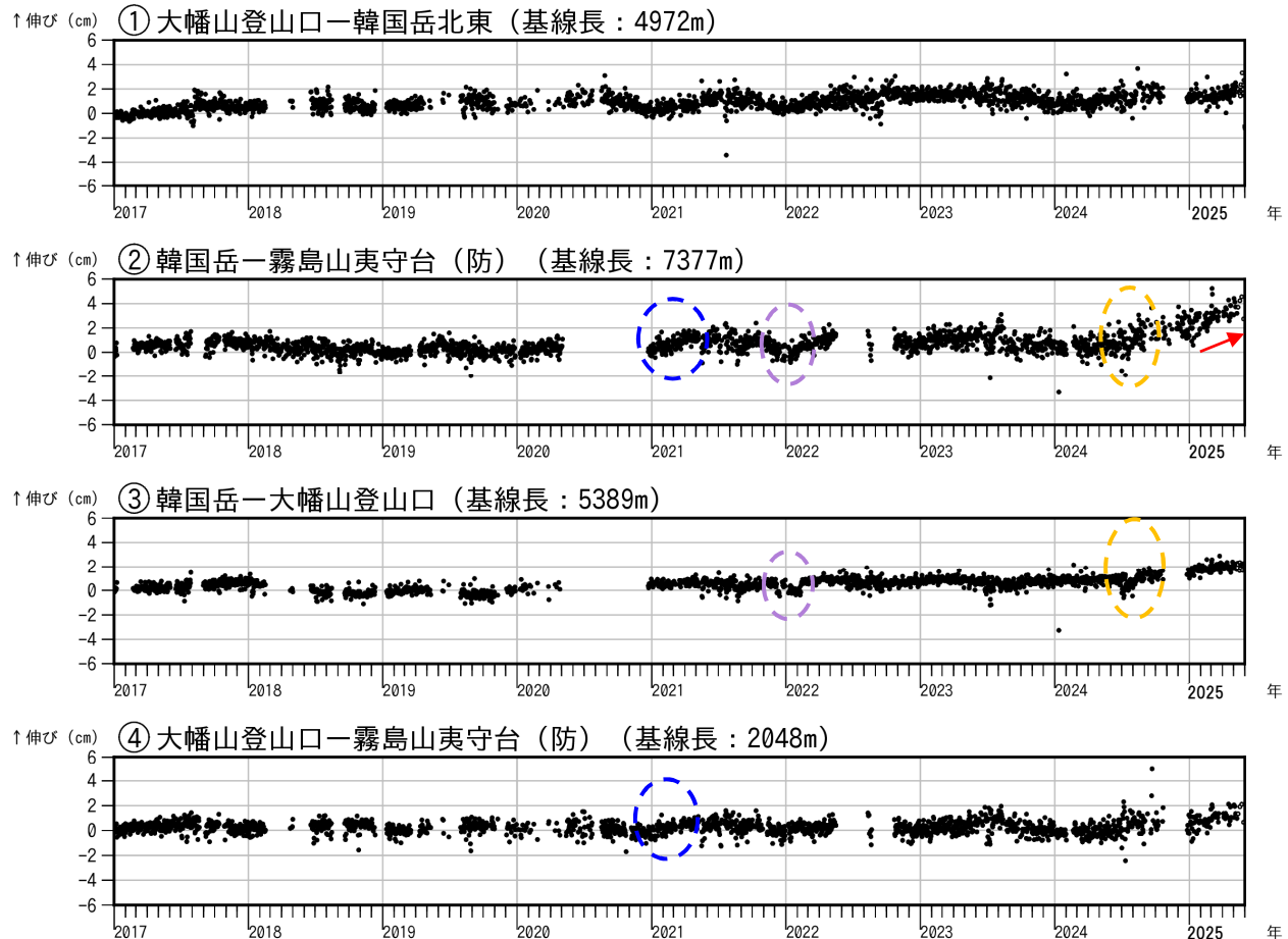
図4 霧島山（大幡池） GNSS 連続観測による基線長変化（2017年1月～2025年5月）
