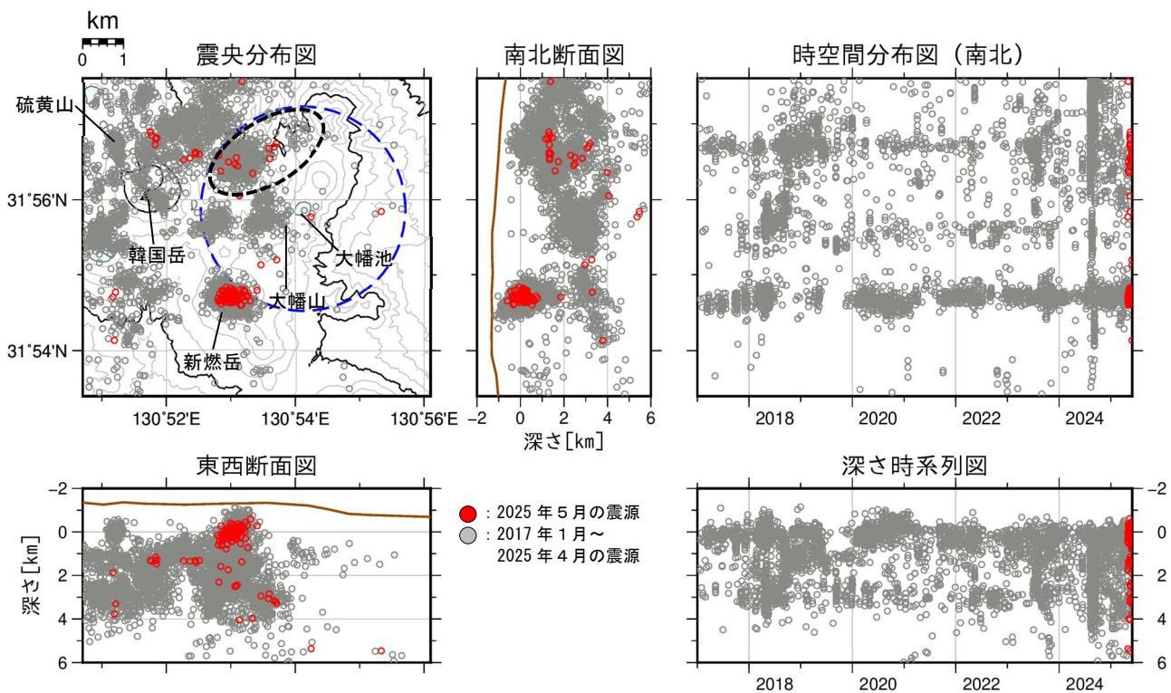
図 3 霧島山（大幡池） 震源分布図（2017 年 1 月～2025 年 5 月）
