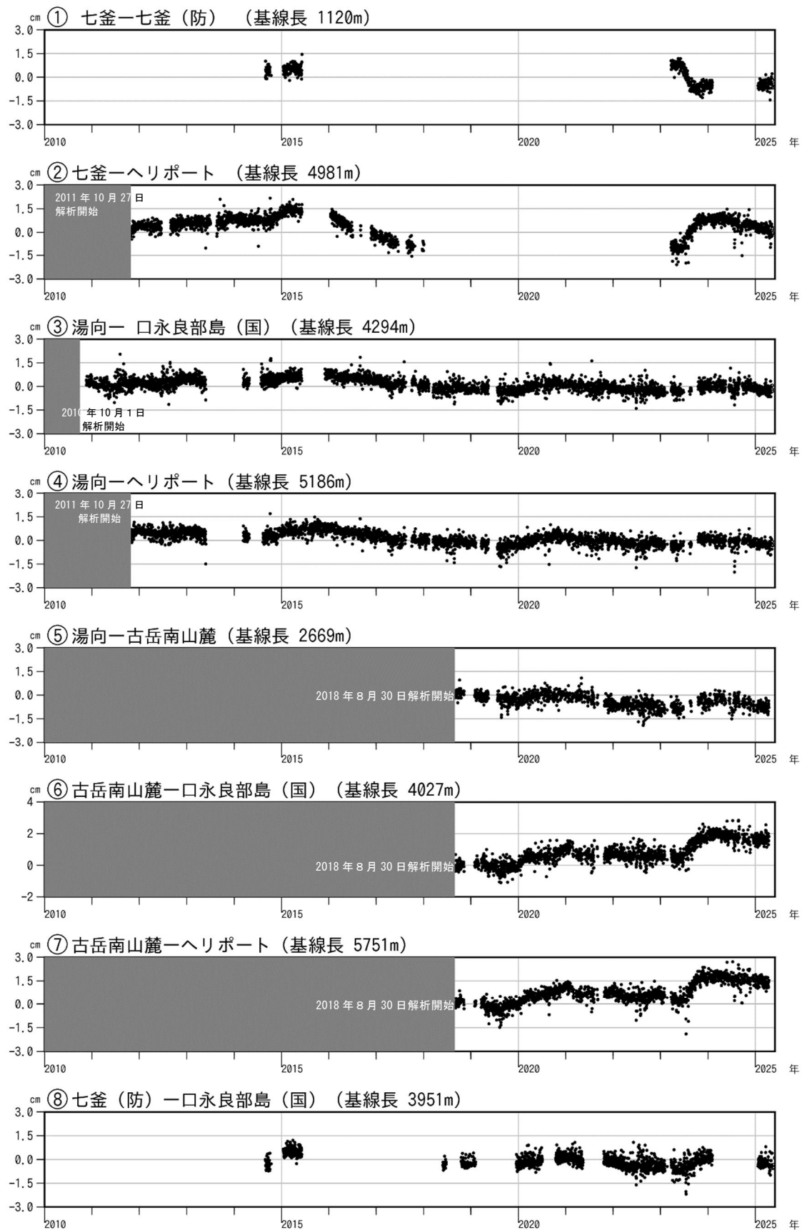
図 6-2 口永良部島 GNSS 連続観測による基線長変化（2010 年 1 月～2025 年 5 月）
