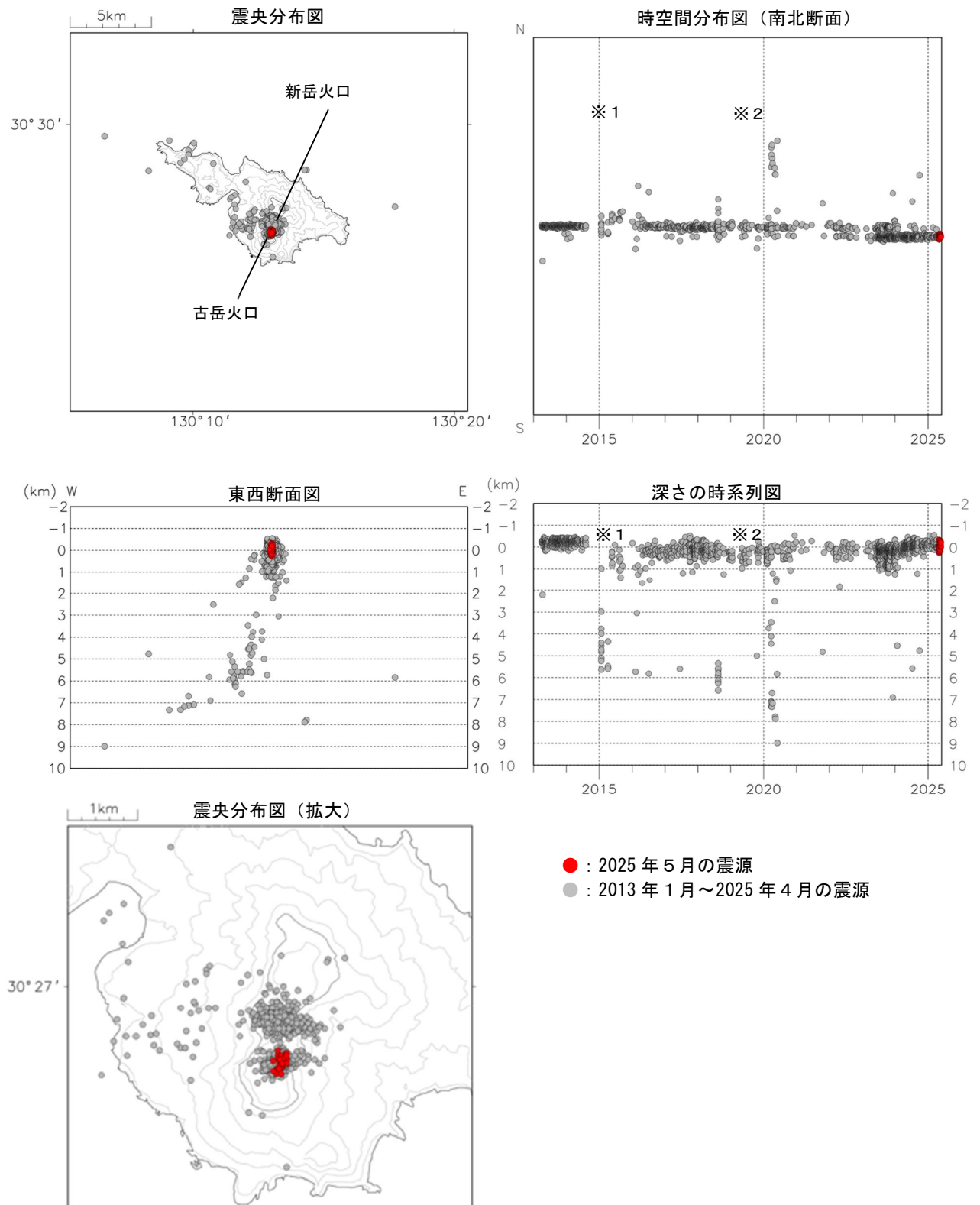
図5 口永良部島 震源分布図（2013年1月～2025年5月）
