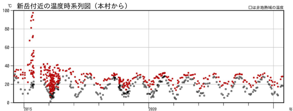
図 2-5 口永良部島 新岳火口西側割れ目付近の地熱域の温度時系列 (2014 年 9 月～2025 年 5 月、本村から観測)
