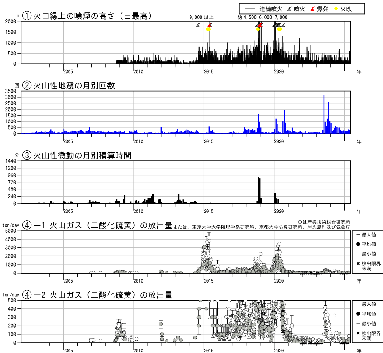
図3 口永良部島 火山活動経過図（2002年1月～2025年5月）
