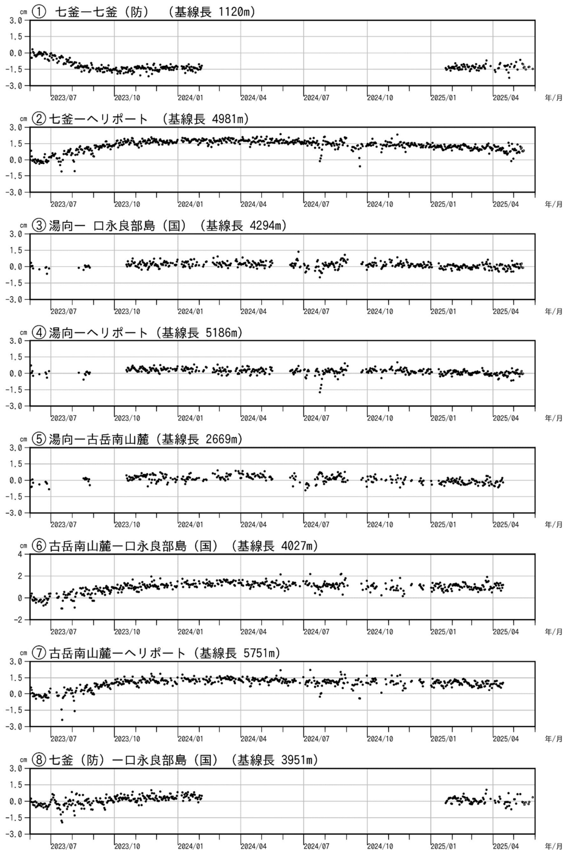
図 6-1 口永良部島 GNSS 連続観測による基線長変化（2023 年 6 月～2025 年 5 月）
