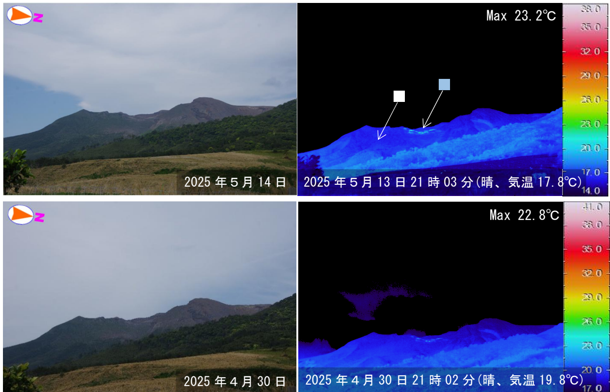
図 2-2 口永良部島 古岳周辺の地熱域の状況（湯向から観測）
