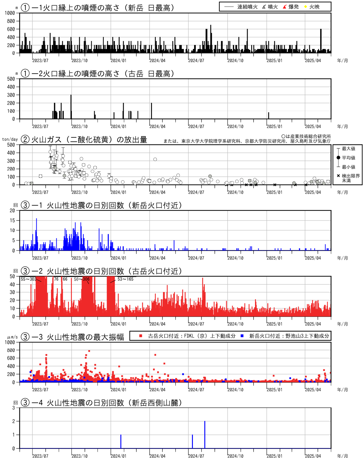
図4 ロ永良部島 最近の火山活動経過図（2023年6月～2025年5月）
