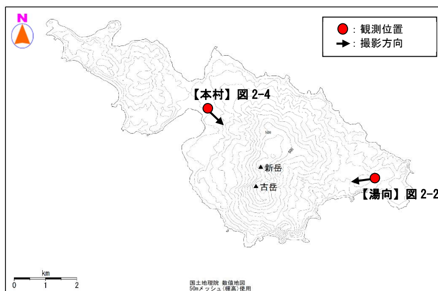
図2-1 口永良部島 観測位置及び撮影方向
