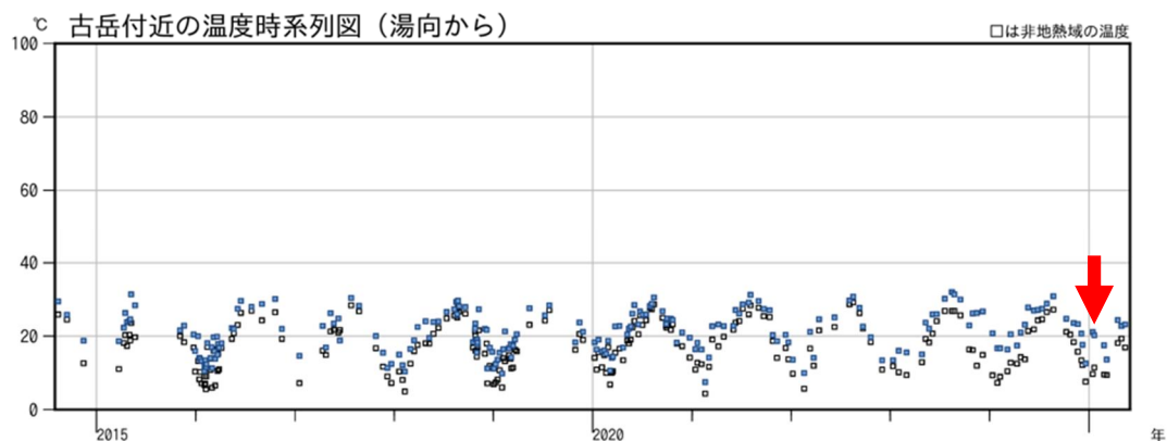
図 2-3 口永良部島 古岳火口付近の地熱域の温度時系列 （2014年9月～2025年5月、湯向から観測）
