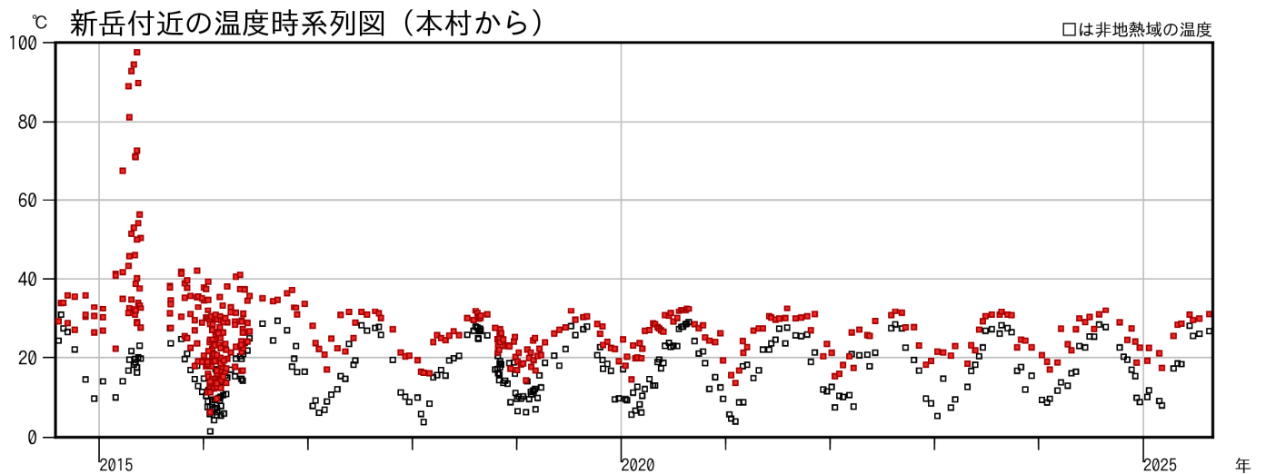
図 3-6 口永良部島 新岳火口西側割れ目付近の地熱域の温度時系列 (2014 年 9 月～2025 年 9 月 5 日（期間外）、本村から観測)
