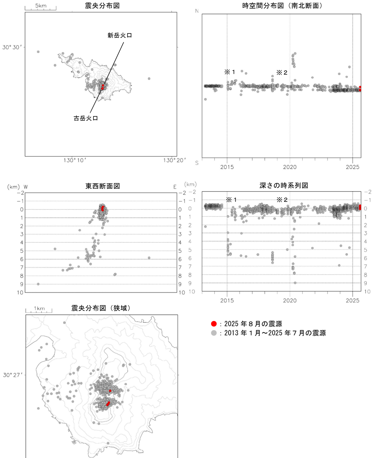
図6 口永良部島 震源分布図（2013年1月～2025年8月）
