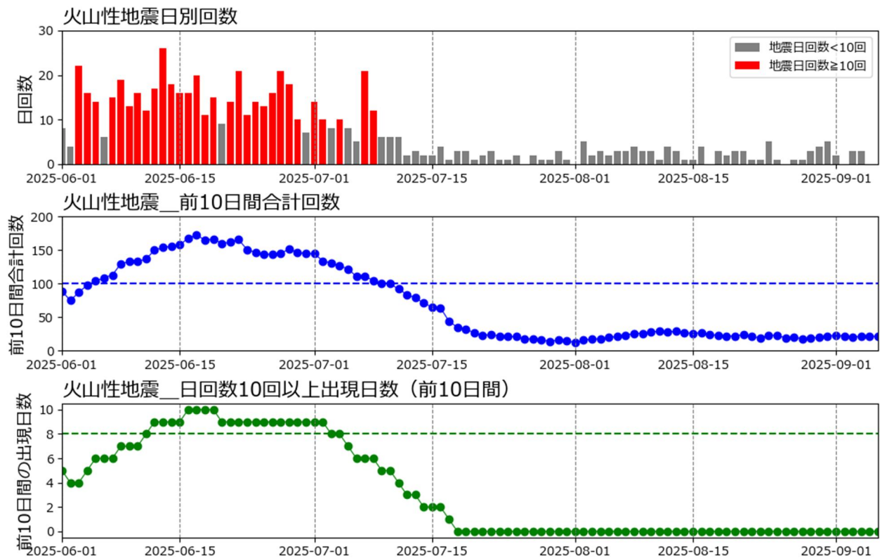
図1 口永良部島 【1段】火山性地震の日別回数、【2段】火山性地震の前10日間合計回数、【3段】火山性地震の日回数10回以上の出現日数（前10日間）（2025年6月1日～9月5日（期間外））
