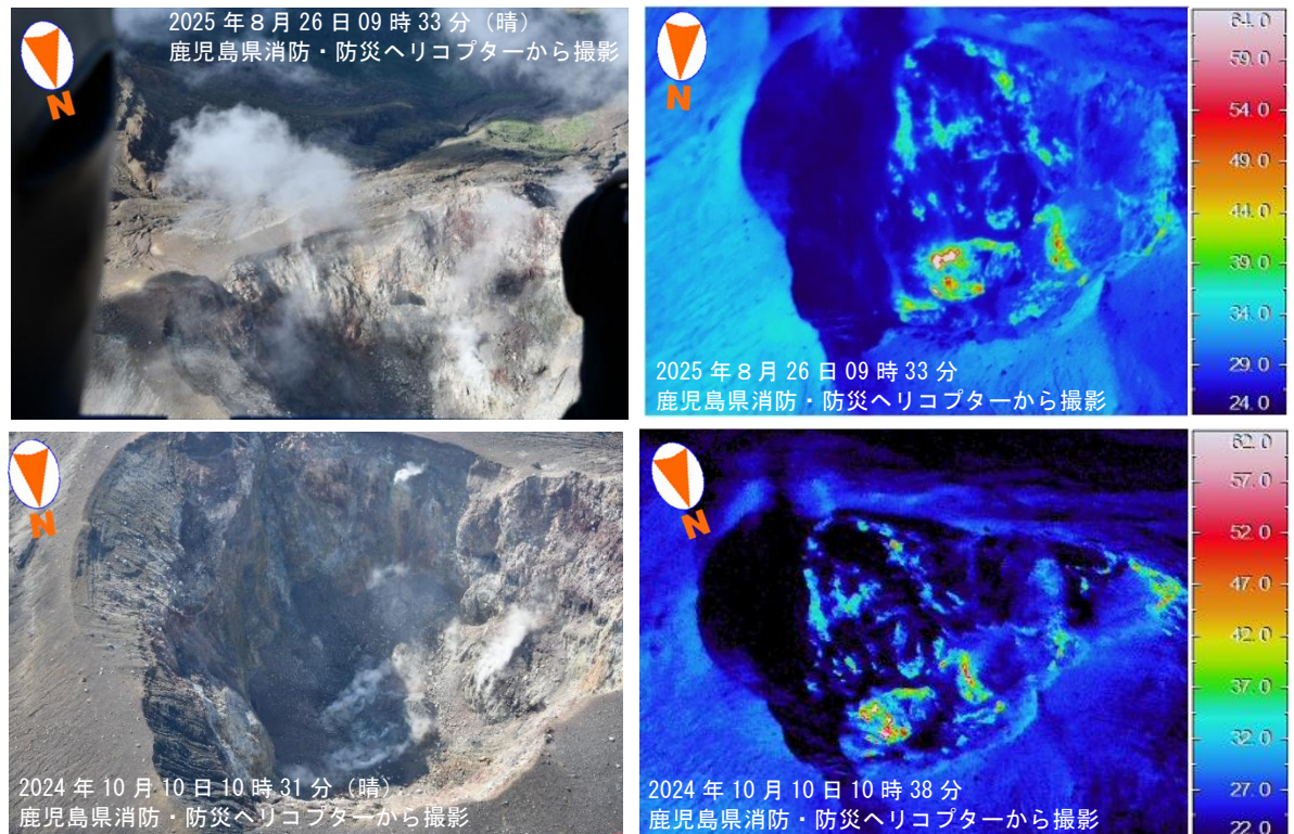
図 3-2 口永良部島 新岳火口内の状況（上空から観測）
