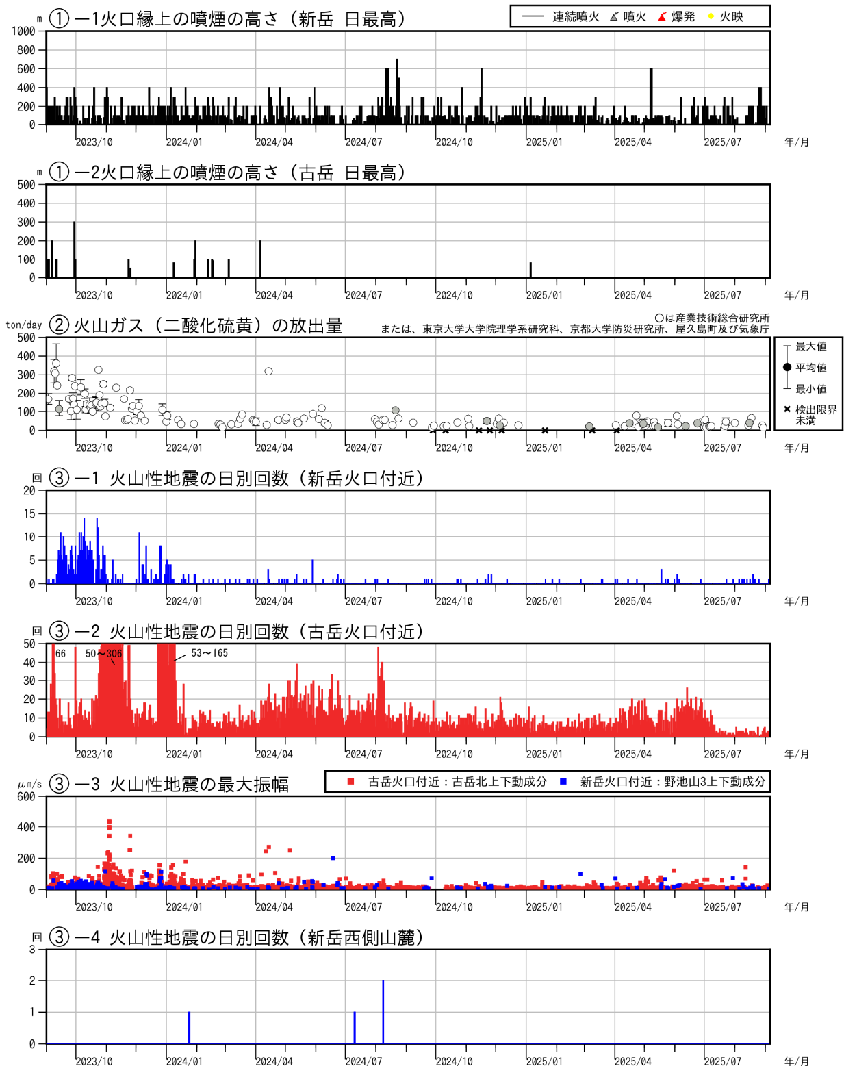
図5 口永良部島 最近の火山活動経過図（2023年9月～2025年9月5日（期間外））
