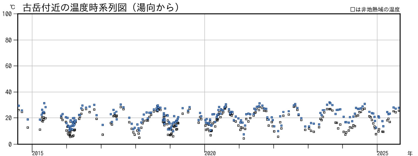
図 3-4 口永良部島 古岳火口付近の地熱域の温度時系列 （2014年9月～2025年9月5日（期間外）、湯向から観測）
