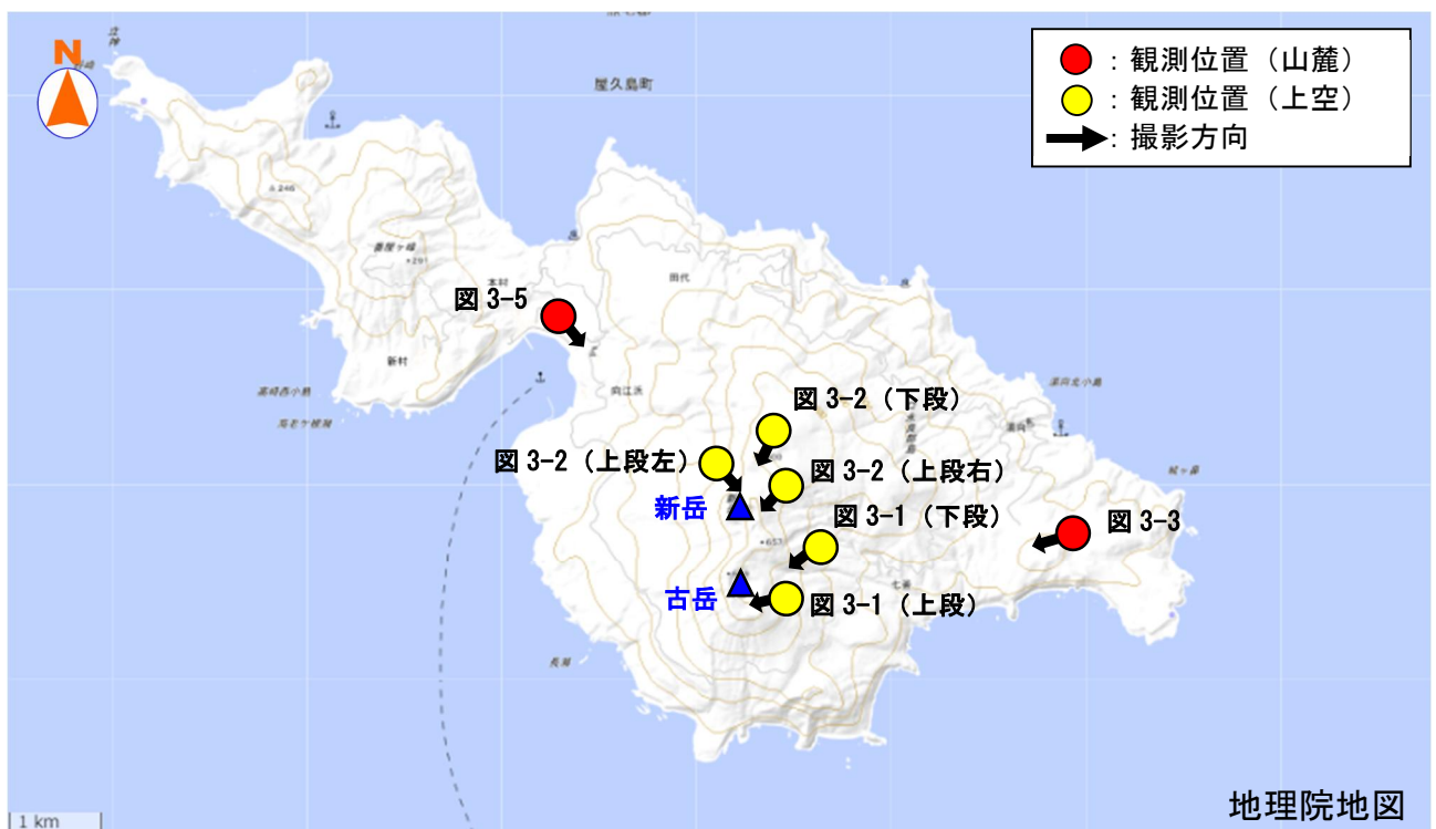
図2 口永良部島 観測位置及び撮影方向
