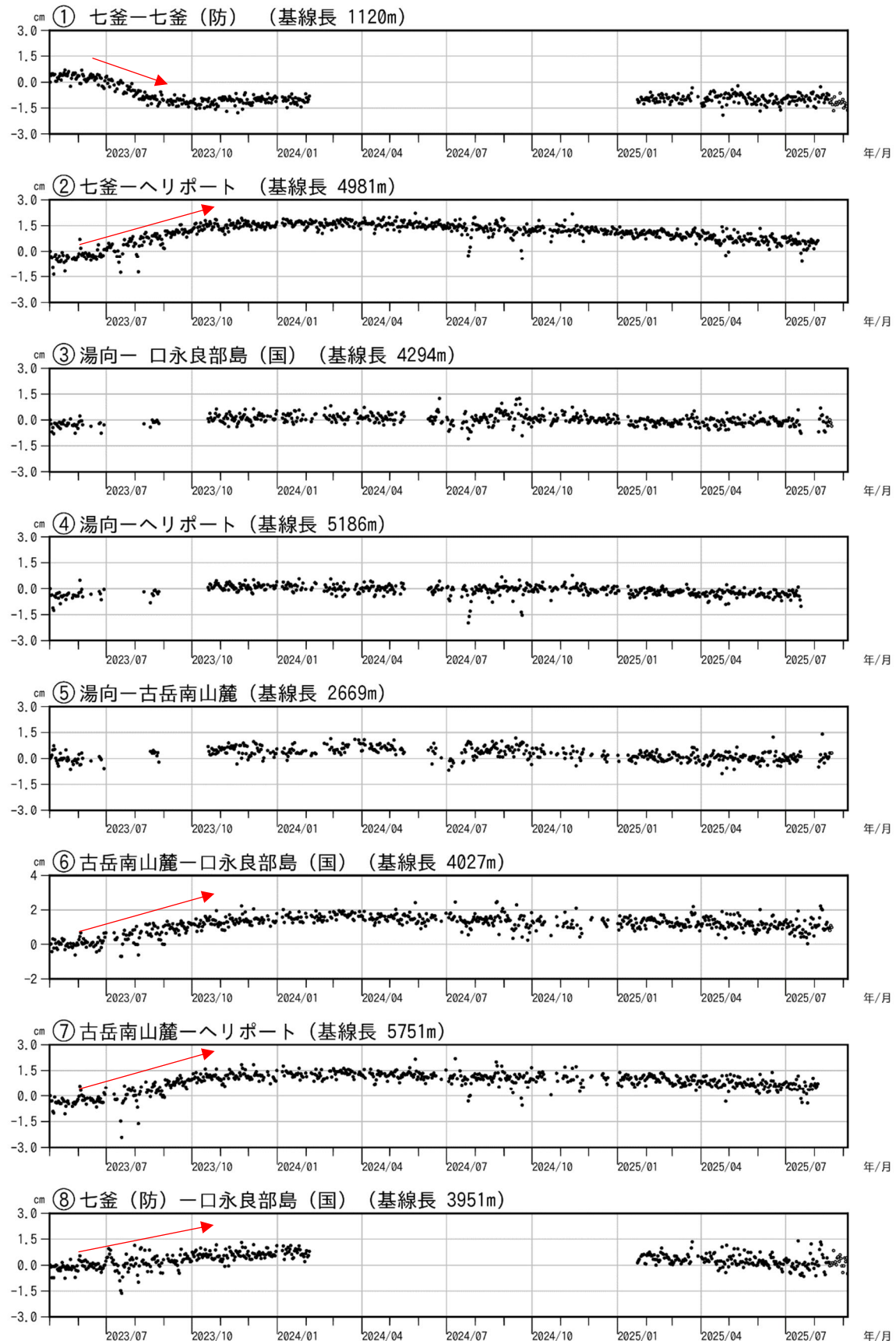
図 7-1 口永良部島 GNSS 連続観測による基線長変化（2023 年 5 月～2025 年 9 月 5 日（期間外））
