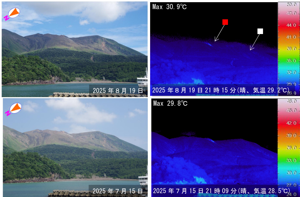
図 3-5 口永良部島 新岳火口及び新岳火口西側割れ目付近の状況（本村から観測）
