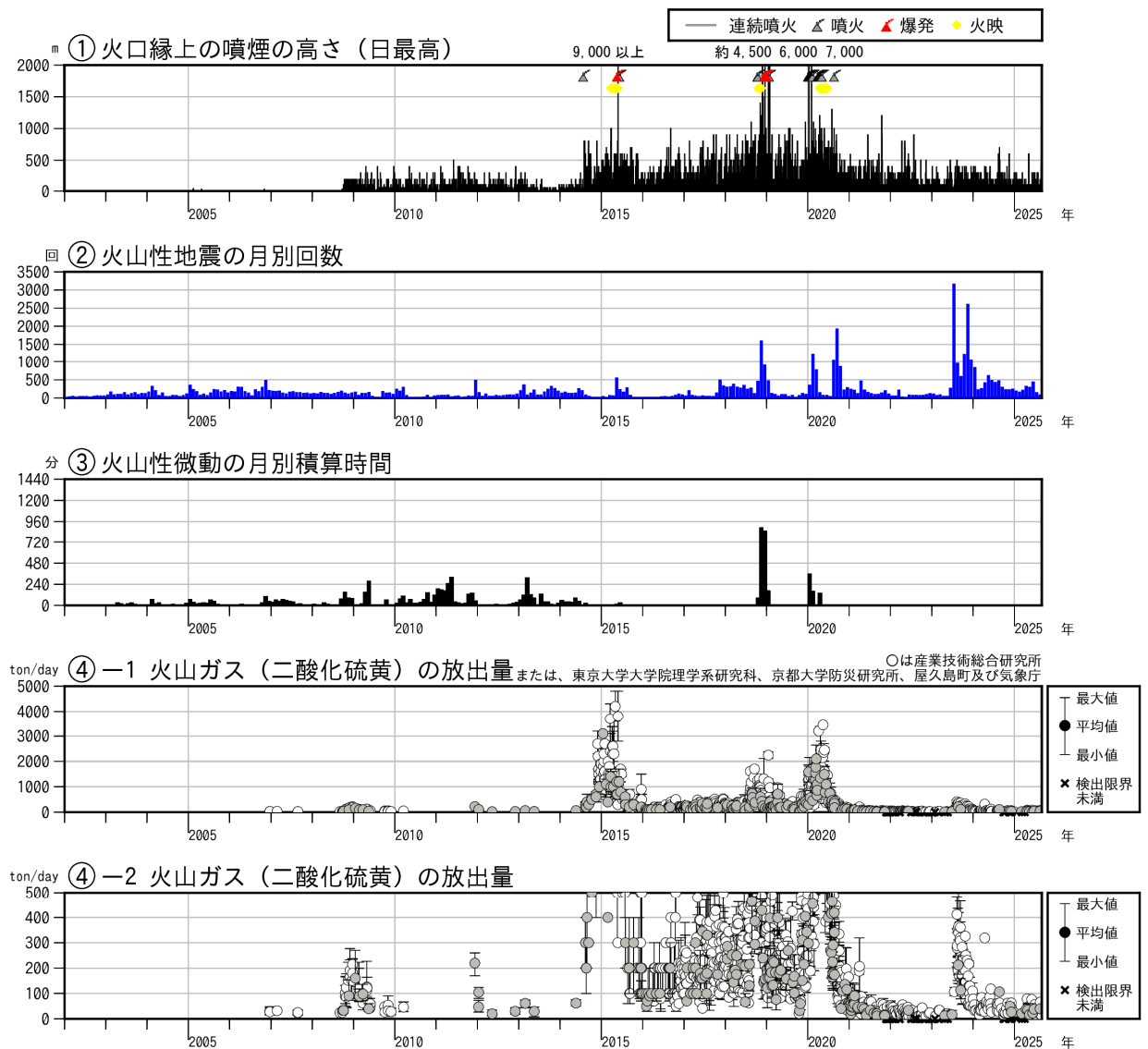
図4 口永良部島 火山活動経過図（2002年1月～2025年8月）
