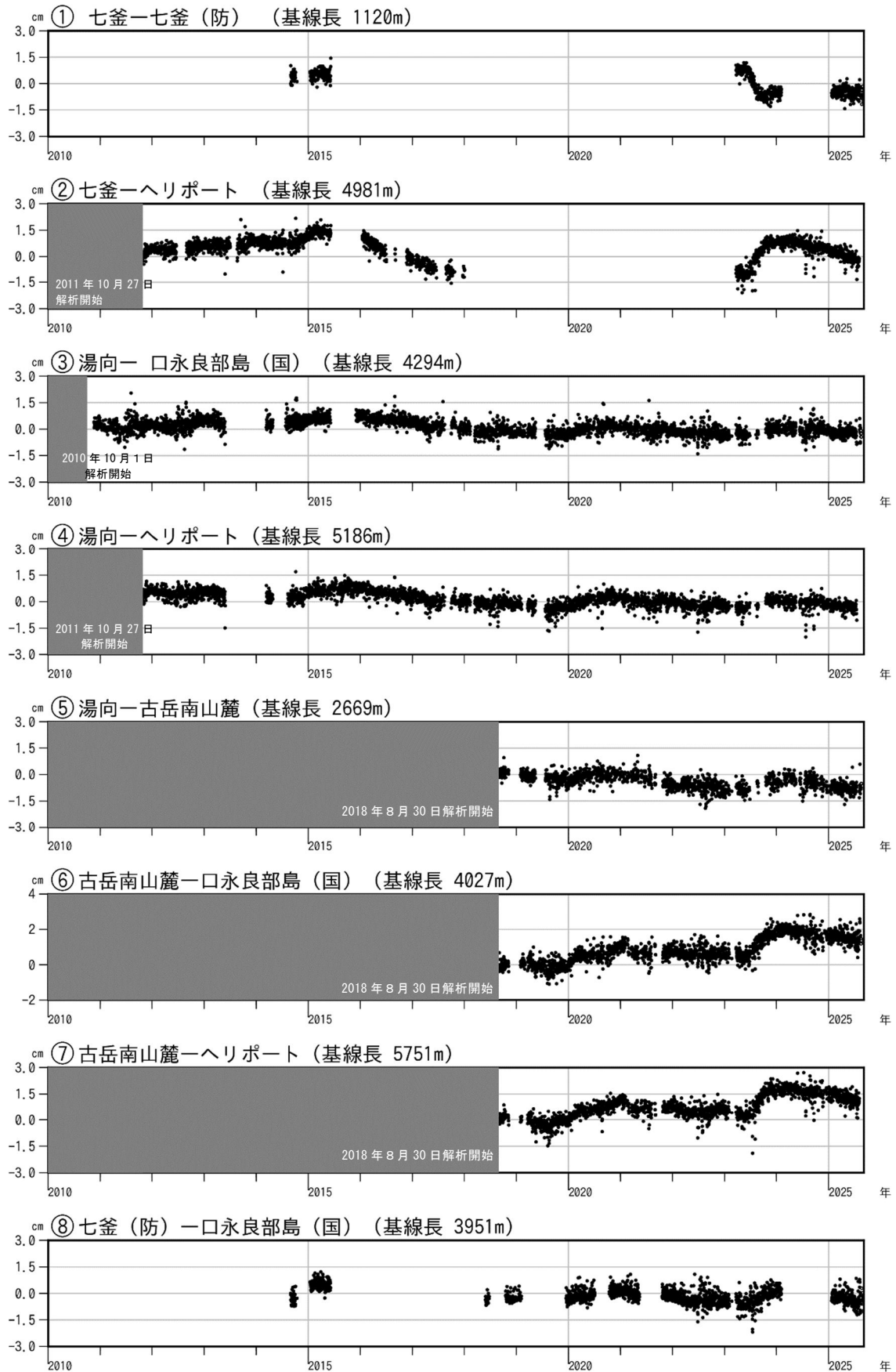
図 7-2 口永良部島 GNSS 連続観測による基線長変化（2010 年 1 月～2025 年 9 月 5 日（期間外））
