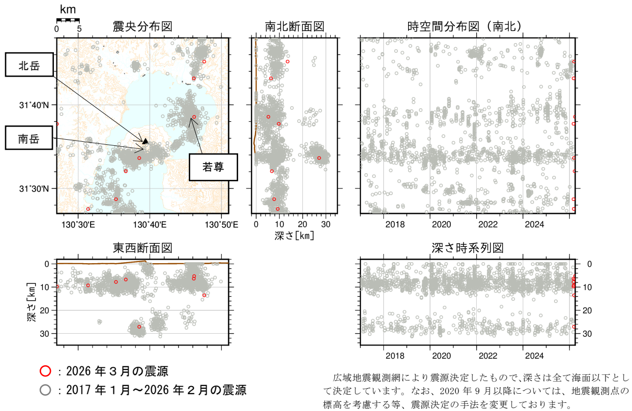
図 4-1 桜島 始良カルデラ周辺の震源分布図（2017 年 1 月～2026 年 3 月）
