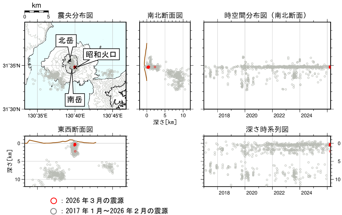
図 4-2 桜島 桜島付近の震源分布図（2017 年 1 月～2026 年 3 月）
