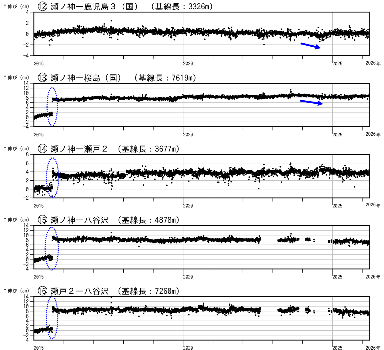
図 9-3 桜島 GNSS 連続観測による基線長変化（2015 年 1 月～2026 年 3 月）
