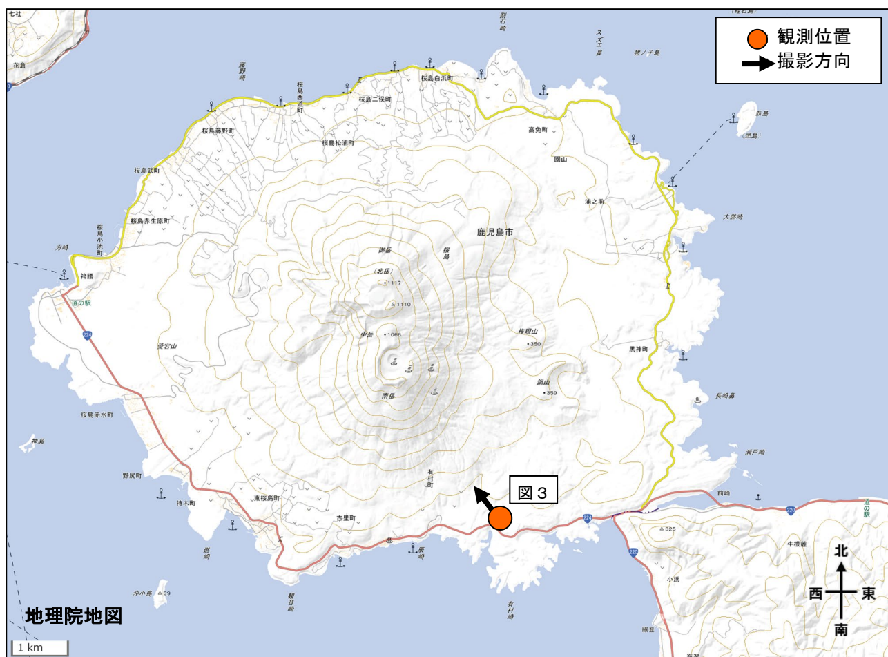
図2 桜島 現地調査観測位置及び撮影方向
