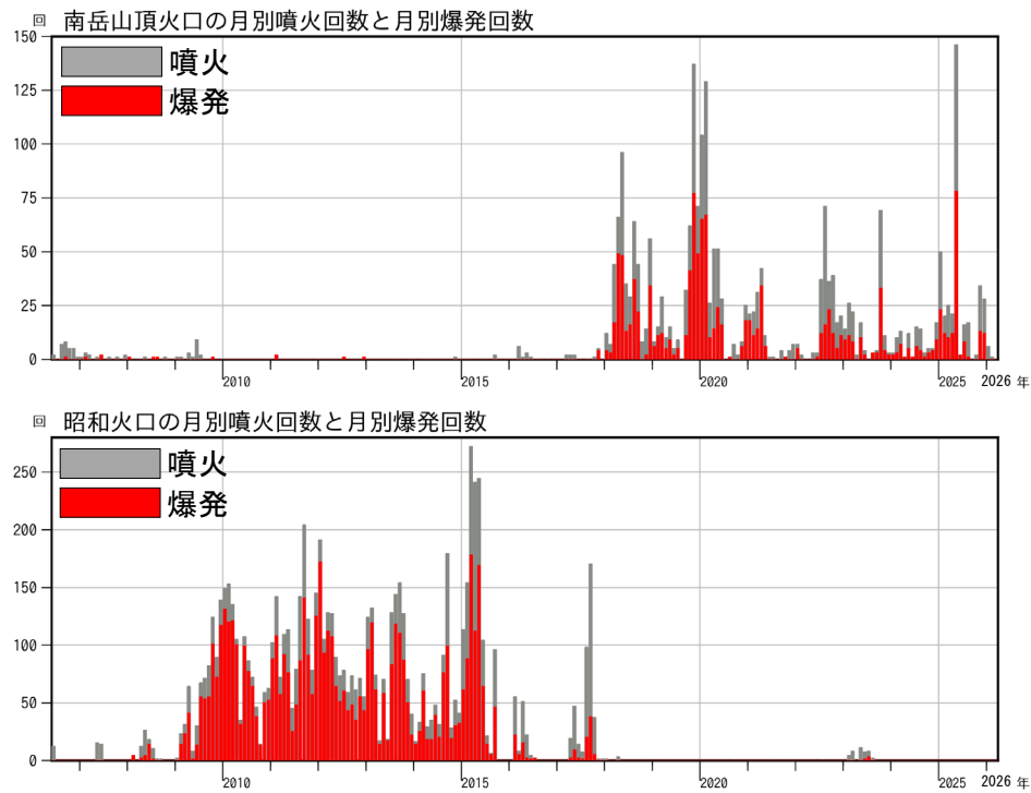
図5 桜島 南岳山頂火口（上図）と昭和火口（下図）の月別噴火回数と月別爆発回数 （2006年6月～2026年3月）
