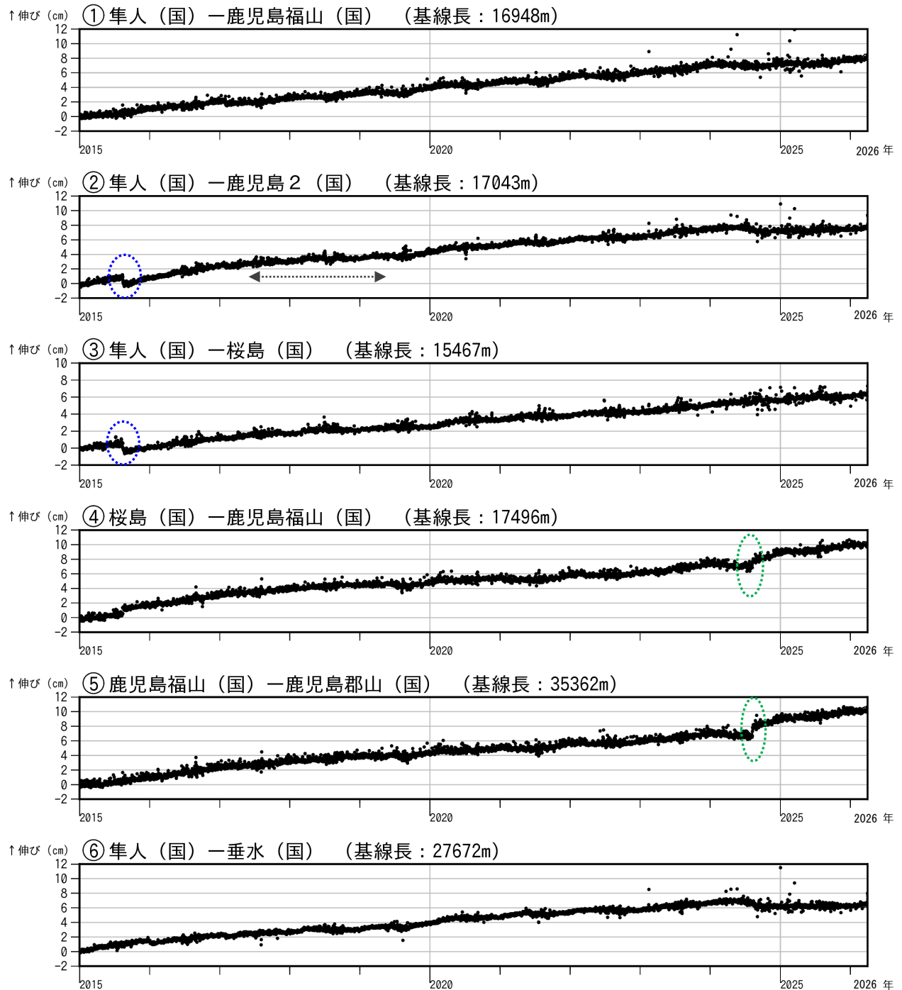
図 9-1 桜島 GNSS 連続観測による基線長変化 (2015 年 1 月～2026 年 3 月)
