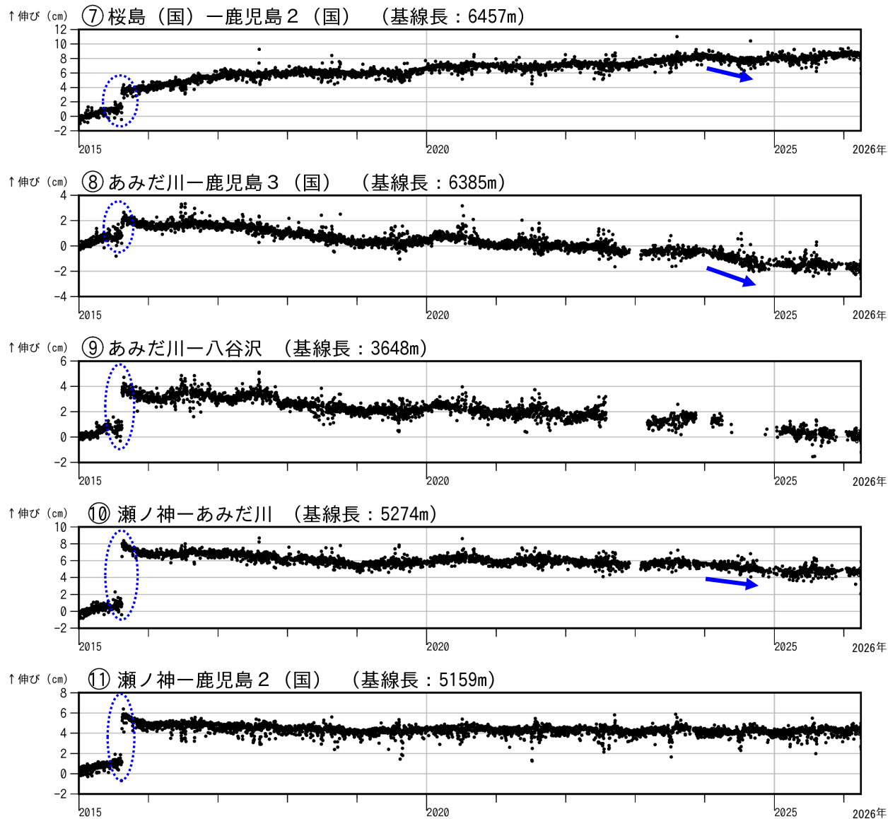
図9-2 桜島 GNSS 連続観測による基線長変化（2015年1月～2026年3月）
