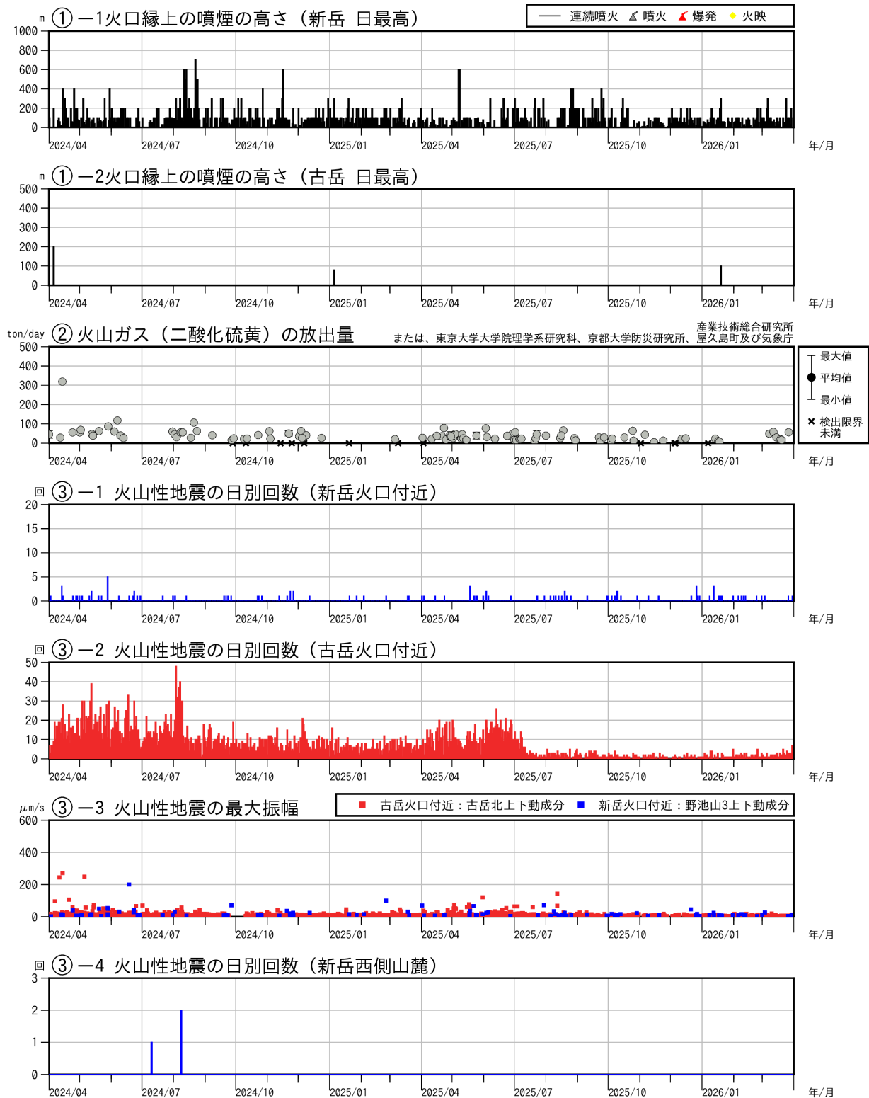
図4 口永良部島 最近の火山活動経過図（2024年4月～2026年3月）
