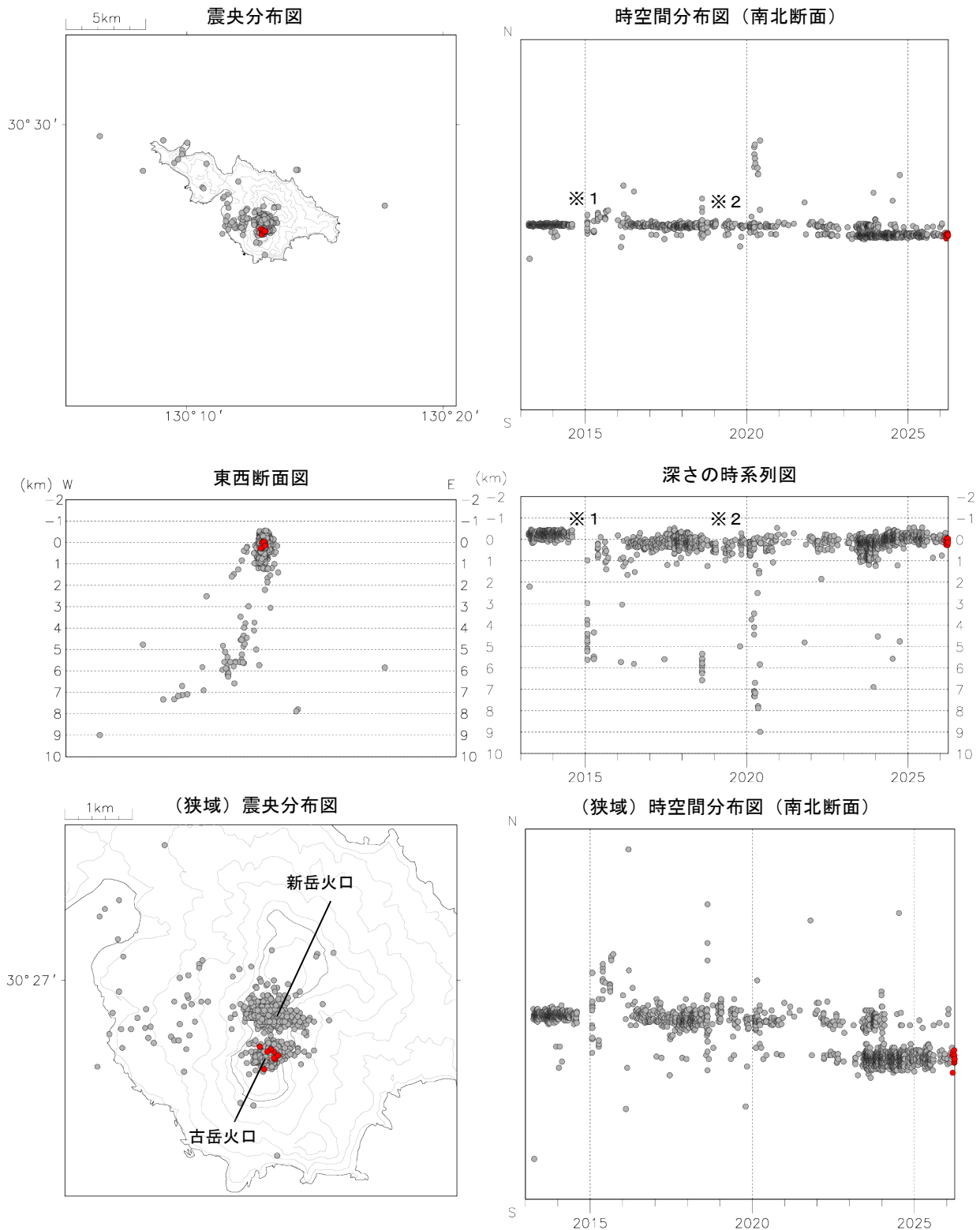
図5 口永良部島 震源分布図（2013年1月～2026年3月）
