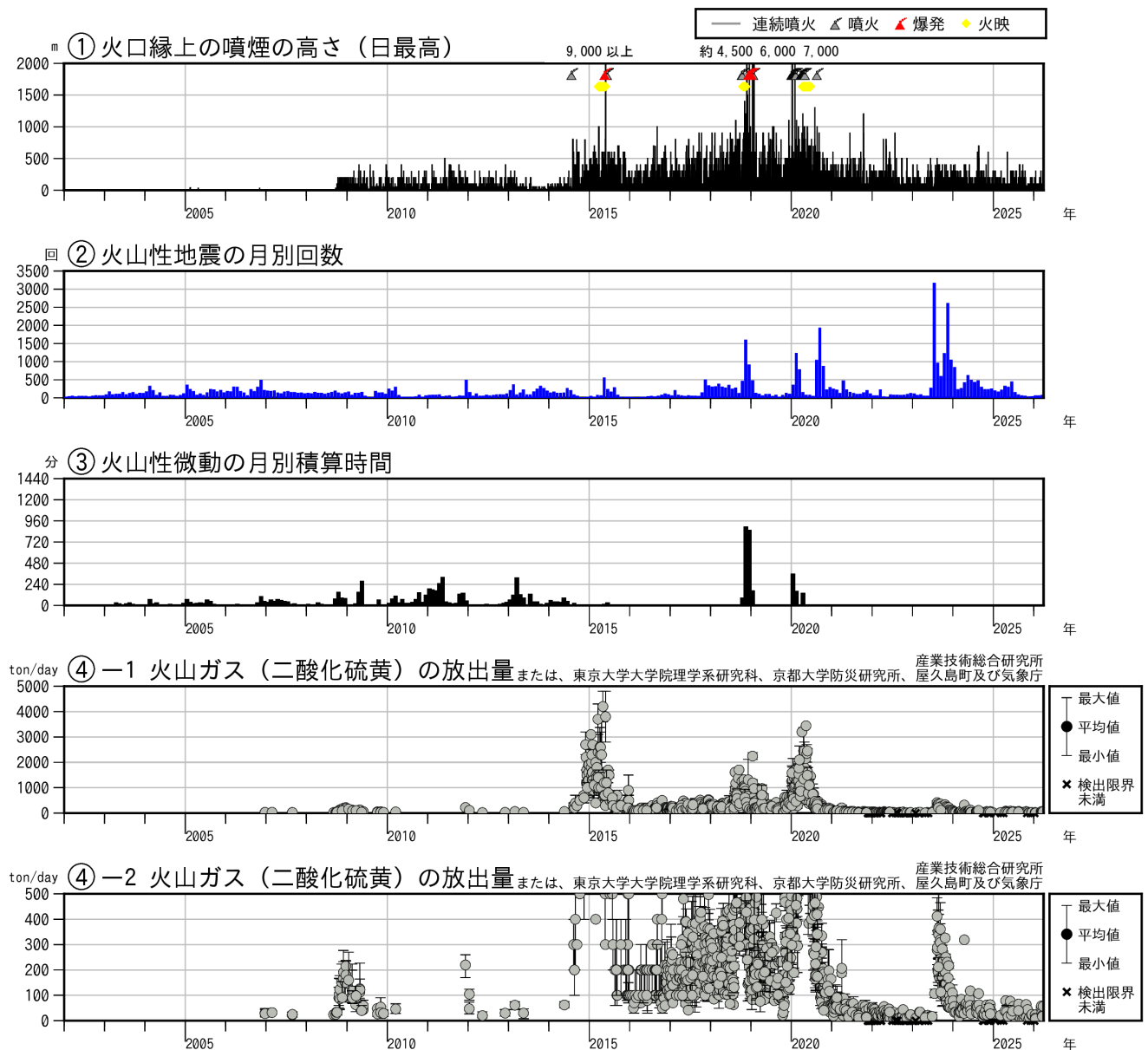
図3 口永良部島 火山活動経過図（2002年1月～2026年3月）
