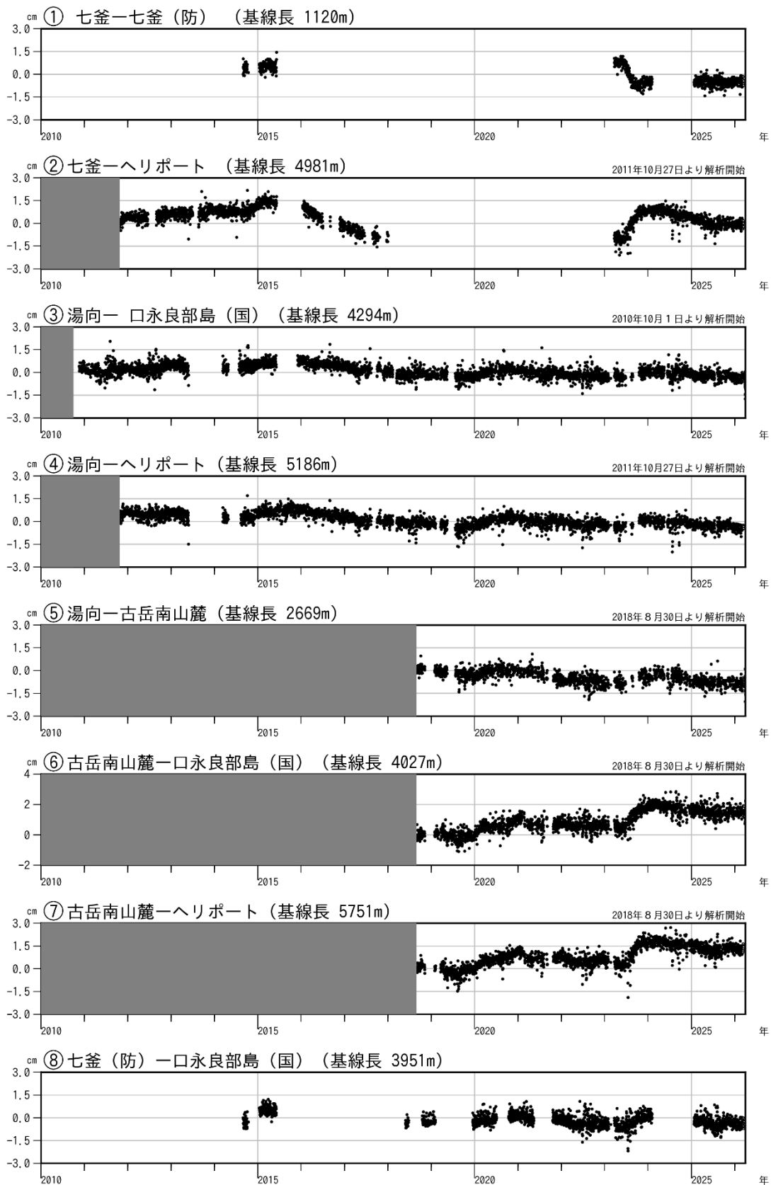
図6 口永良部島 GNSS 連続観測による基線長変化（2010年1月～2026年3月）
