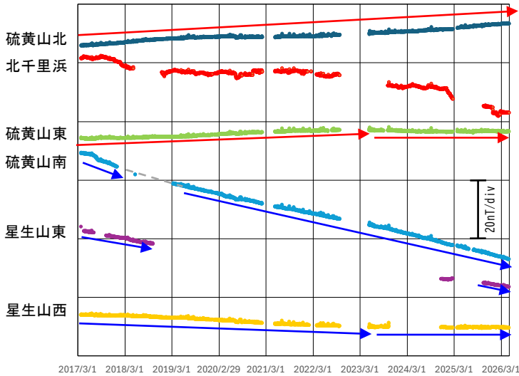
図 4-1 九重山 連続観測による全磁力の変化 (2017 年 3 月～2026 年 4 月)
