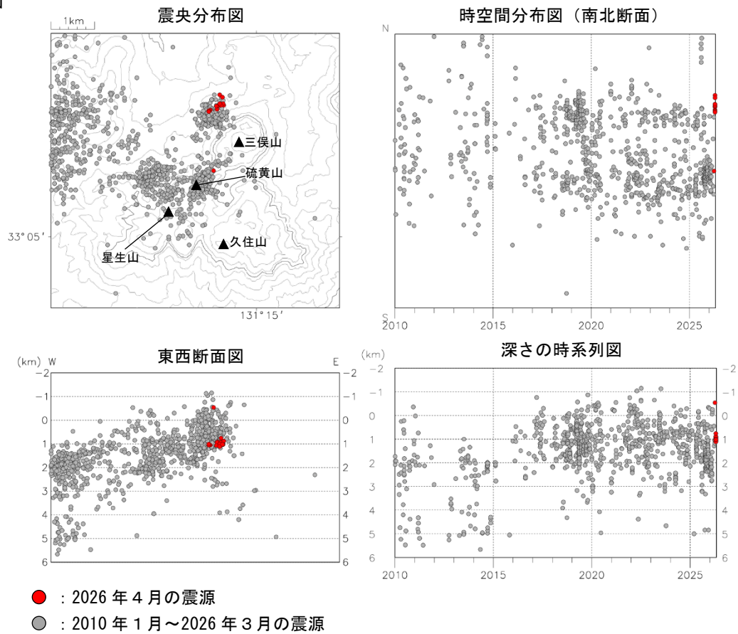
図3 九重山 震源分布図 ①広域図 ②狭域図（2010年1月～2026年4月）
