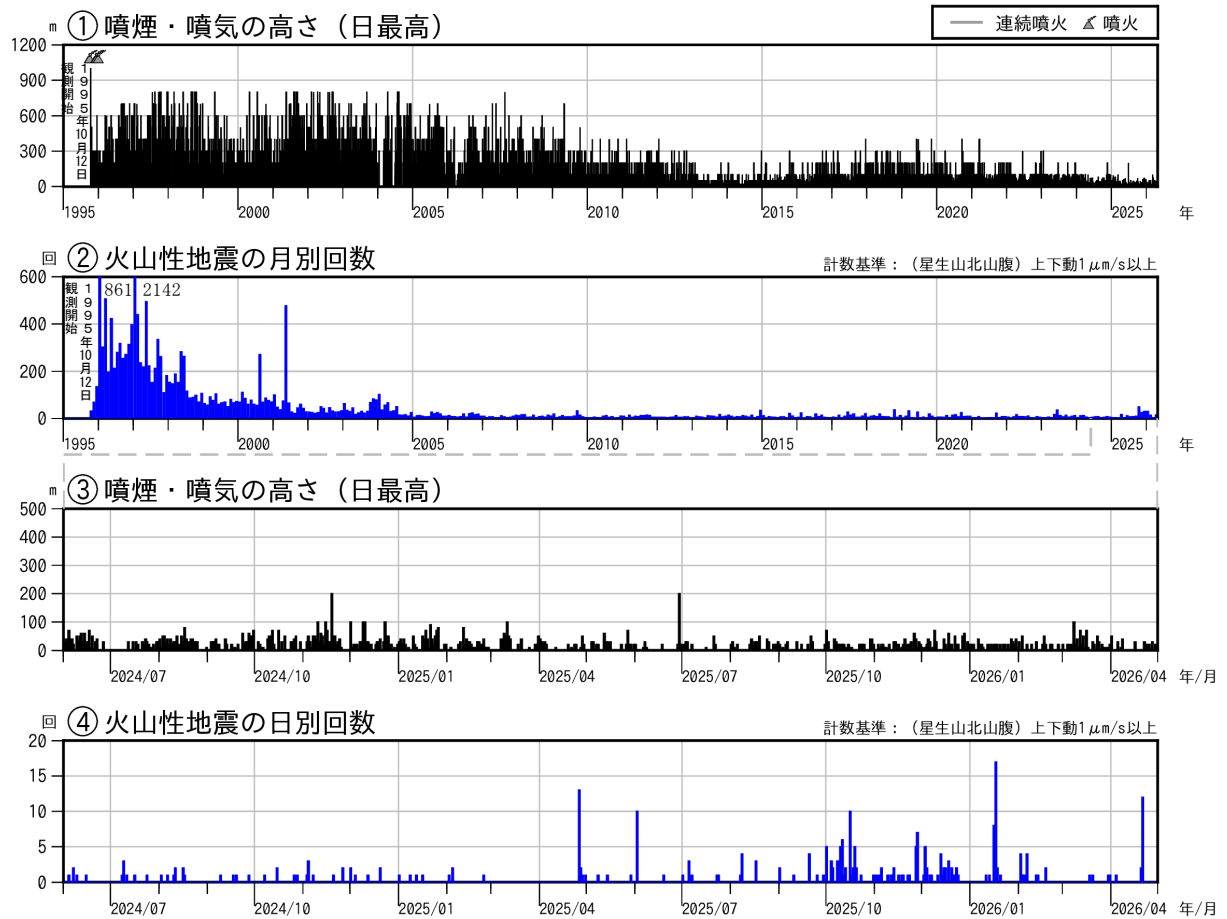
図2 九重山 火山活動経過図（1995年1月～2026年4月）
