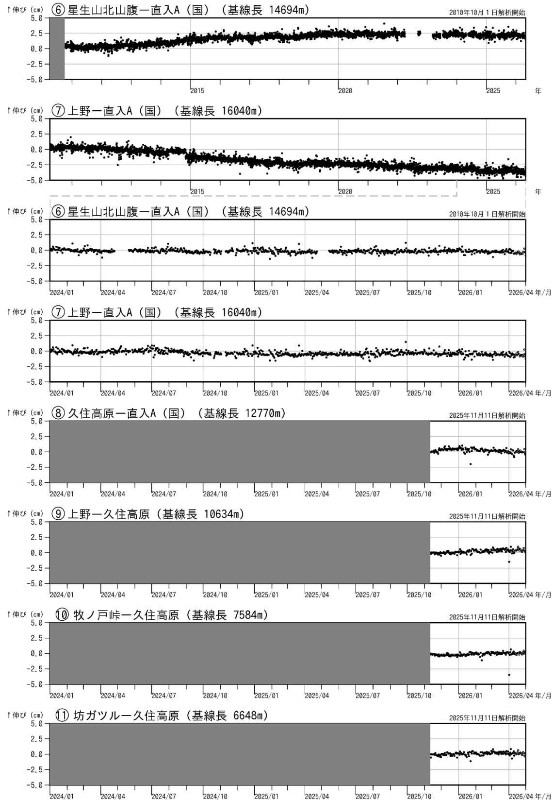
図 5-2 九重山 GNSS 連続観測による基線長変化（2010 年 1 月～2026 年 4 月）
