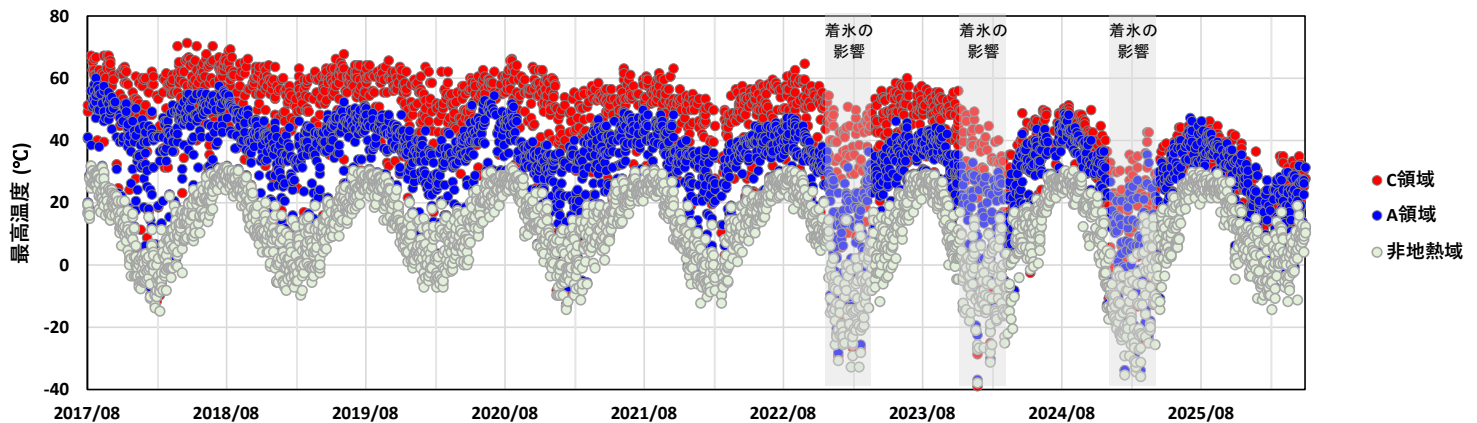
図 1-2 九重山 星生山北尾根の赤外熱映像装置による日別最高温度（2017年8月～2026年4月）
