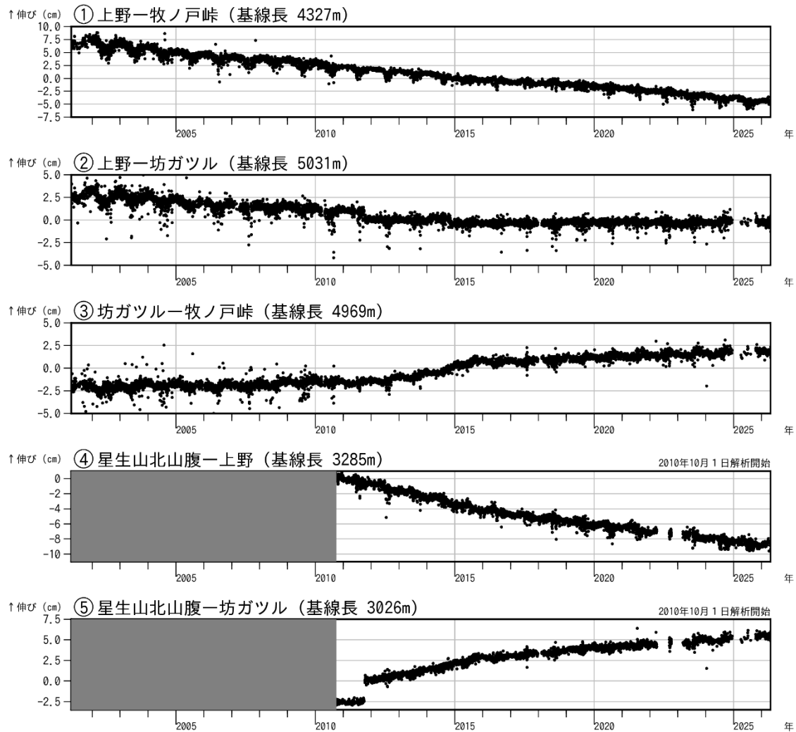
図 5-1 九重山 GNSS 連続観測による基線長変化（2001 年 4 月～2026 年 4 月）
