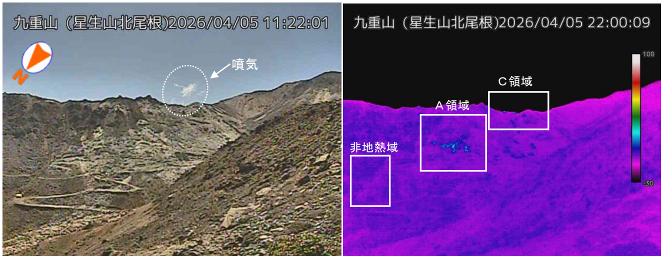
図 1-1 九重山 硫黄山の噴気及び地熱域の状況（4月5日 星生山北尾根監視カメラ）
