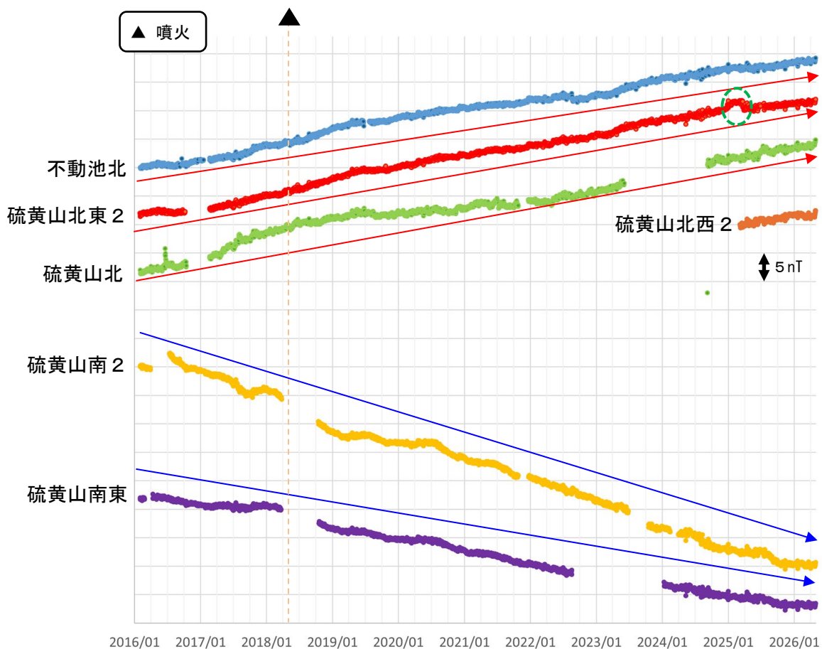
図 6-2 霧島山（えびの高原（硫黄山）周辺） 全磁力観測点で観測された全磁力変動 （2016年1月～2026年4月）
