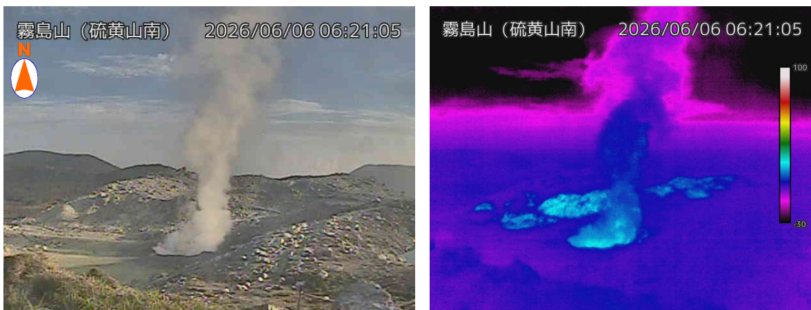
図1-2 霧島山（えびの高原（硫黄山）周辺） 硫黄山南側の状況 （6月6日、硫黄山南監視カメラ）
