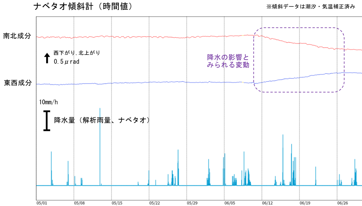
図5 諏訪之瀬島 ナベタオ観測点の傾斜変動（2026年5月～6月）
