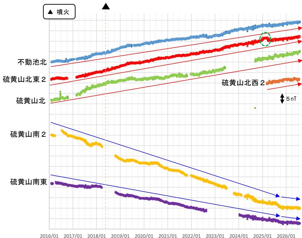
図 9-2 霧島山（えびの高原（硫黄山）周辺） 全磁力観測点で観測された全磁力変動 （2016年1月～2026年7月）
