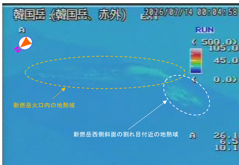
図1 霧島山（新燃岳） 噴煙及び地熱域の状況
