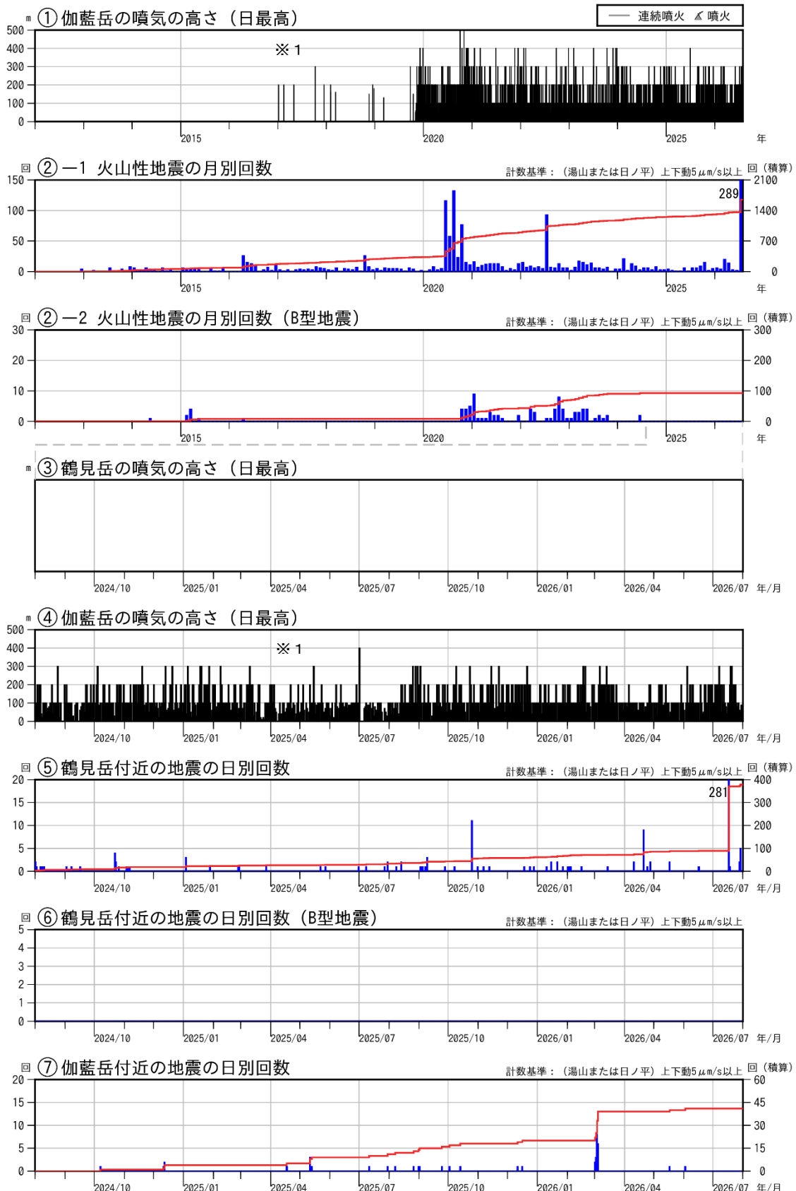
図2 鶴見岳・伽藍岳 火山活動経過図（2012年1月～2026年7月）
