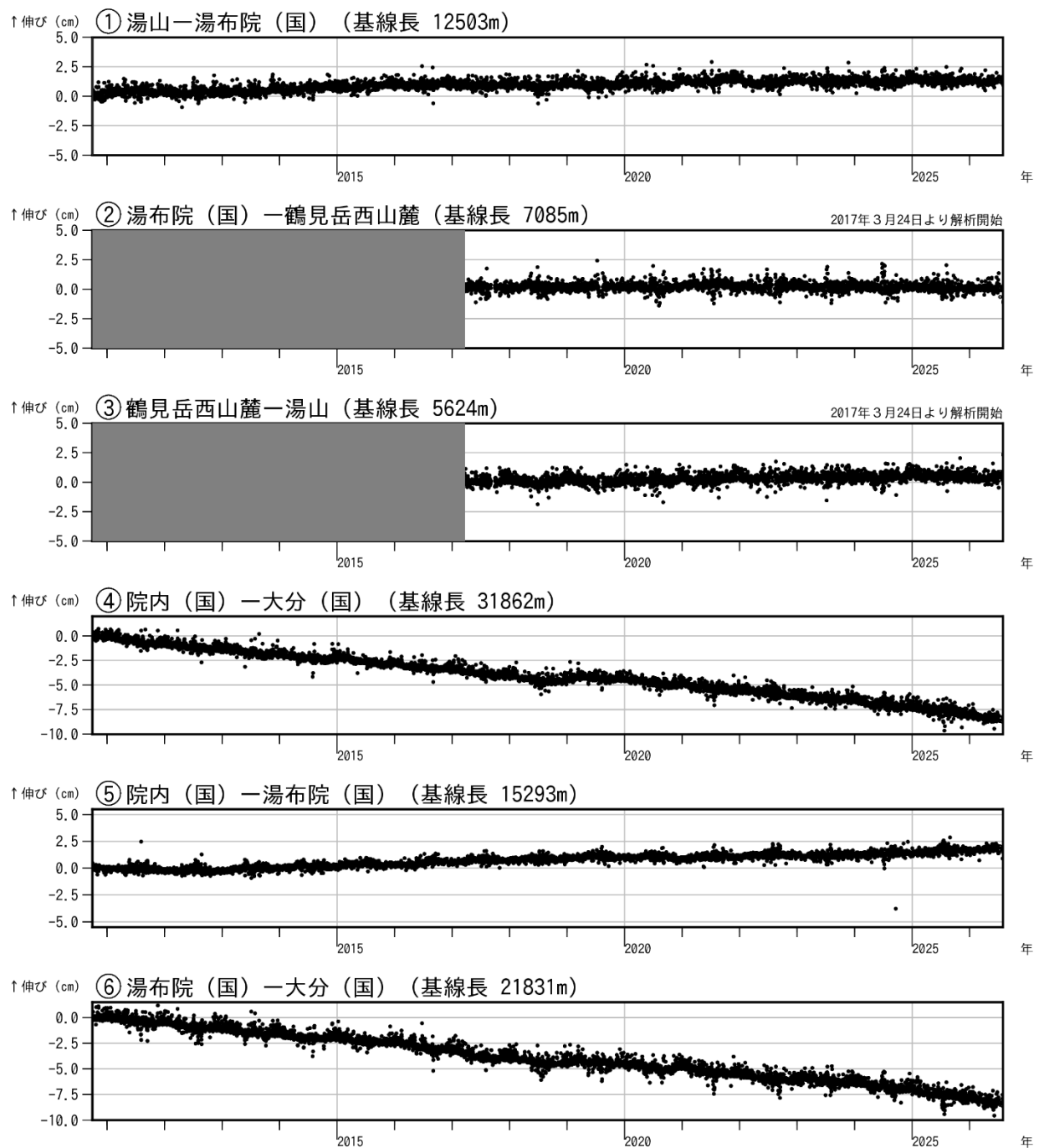
図5 鶴見岳・伽藍岳 GNSS連続観測による基線長変化（2010年10月～2026年7月）
