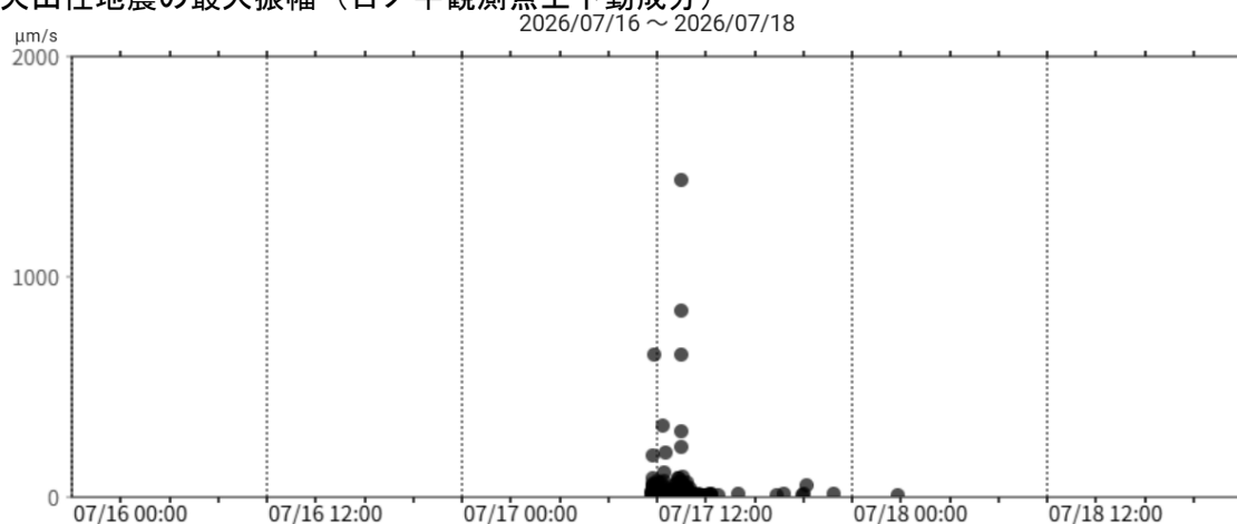
図3 鶴見岳・伽藍岳 火山性地震の発生状況（2026年7月17日11時30分～14時00分、日ノ平観測点上下動成分）、及び時間別地震回数と最大振幅（2026年7月16日～18日）
