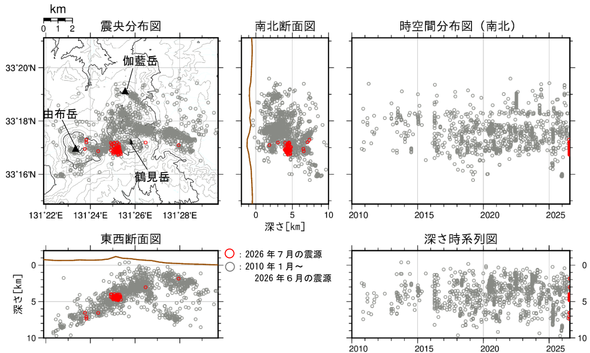
図4 鶴見岳・伽藍岳 震源分布図（2010年1月～2026年7月）
