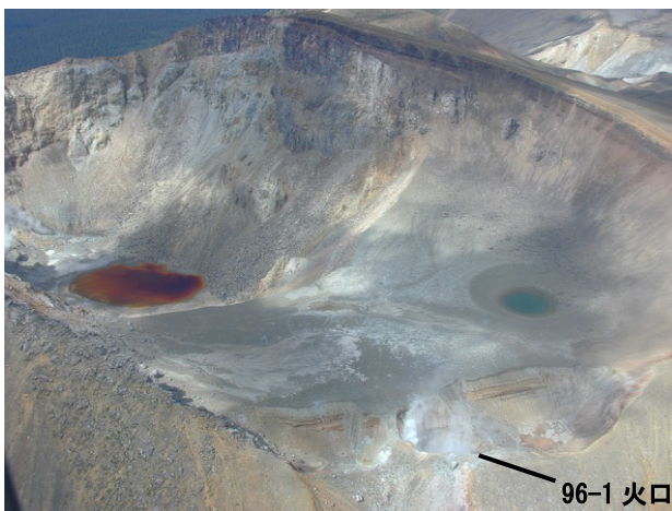
図 5 雌阿寒岳 ポンマチネシリ火口の状況 （8 月 20 日 図 4 ②方向から撮影）
