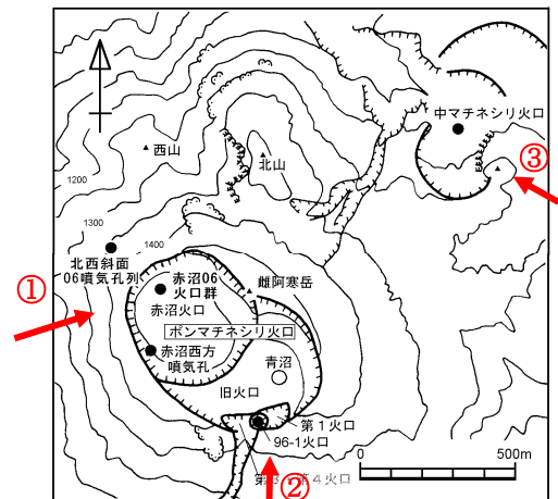
図 4 雌阿寒岳 火口周辺図
