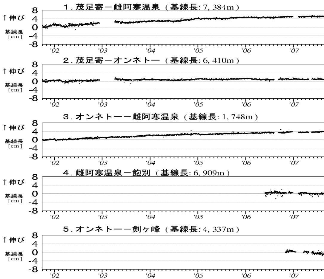
図 8 雌阿寒岳 GPS 連続観測による基線長変化 (2001 年 10 月～2007 年 8 月) グラフの空白部分は欠測 図 8 の 1～5 は、図 9 の GPS 基線①～⑤に対応しています。
