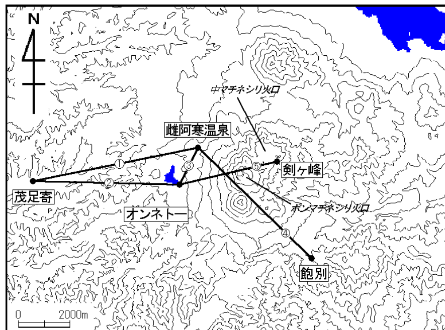
図 9 雌阿寒岳 GPS 連続観測点配置図
