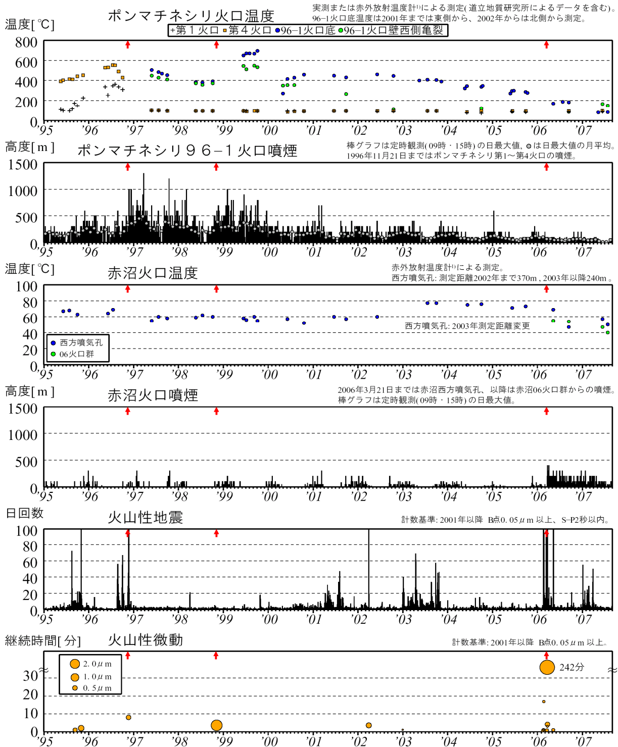
図 2※ 雌阿寒岳 最近の火山活動経過図（1995 年 1 月～2007 年 8 月） ↑印は噴火
