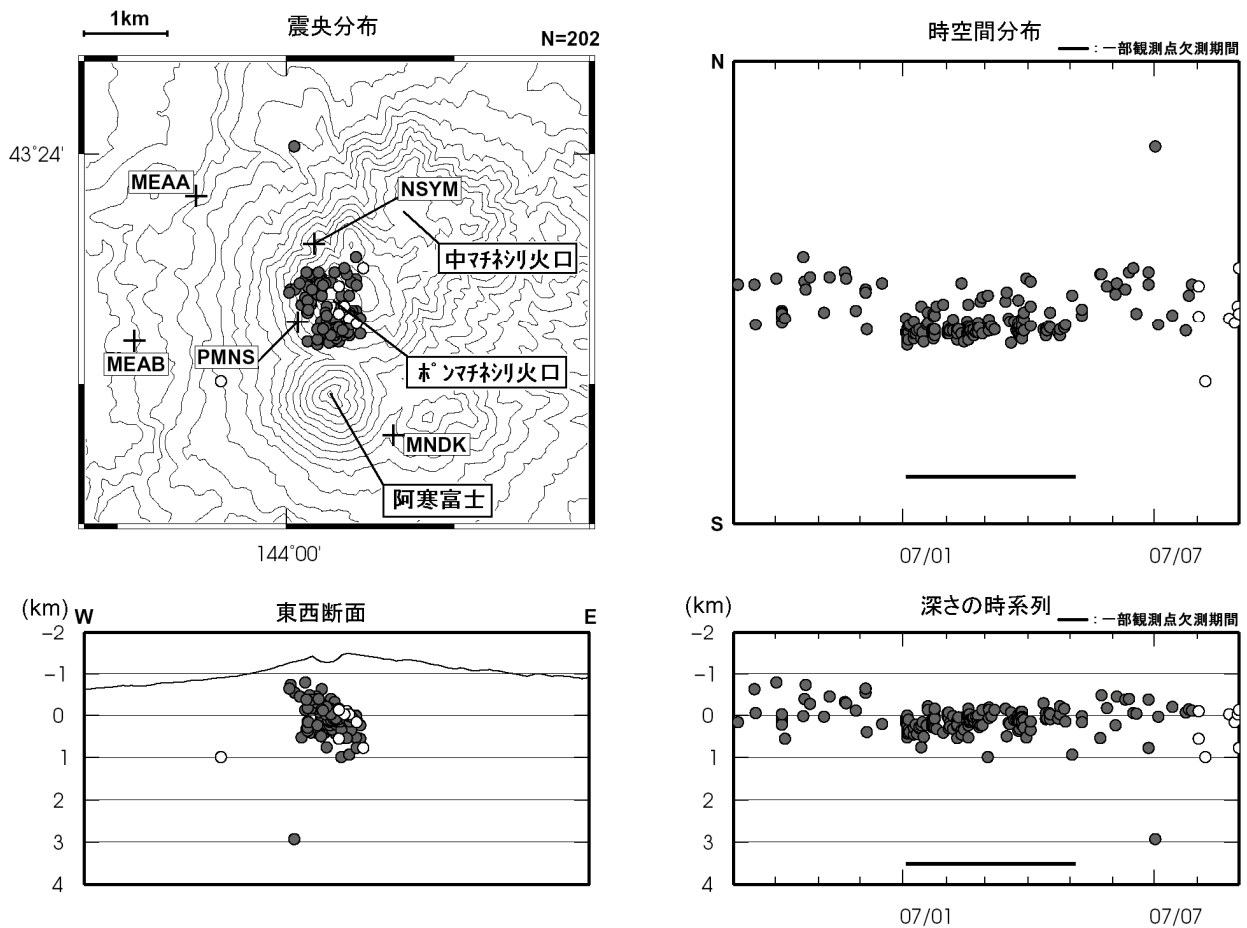
図 7 雌阿寒岳 震源分布図(2006 年 9 月～2007 年 8 月、+は地震観測点)
