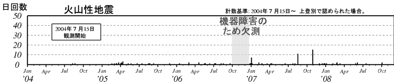
図 2 倶多楽 日別地震回数（2004 年 7 月～2008 年 11 月）
