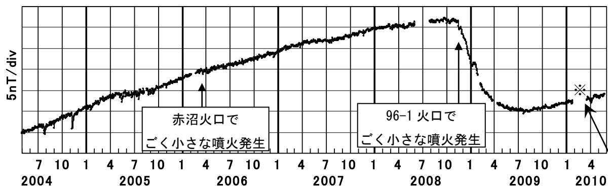
図 4 雌阿寒岳 全磁力連続観測結果（2004 年 5 月 1 日～2010 年 5 月 27 日） MEA と地磁気観測所女満別出張所の全磁力単純差（日平均値） 図 5 の MEA（◎）にて測定 ※ソーラーパネルへの着雪によりバッテリー電圧が低下し、欠測。
