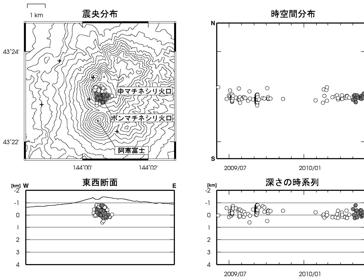
図 6 雌阿寒岳 震源分布図(2009 年 6 月～2010 年 5 月) +は地震観測点
