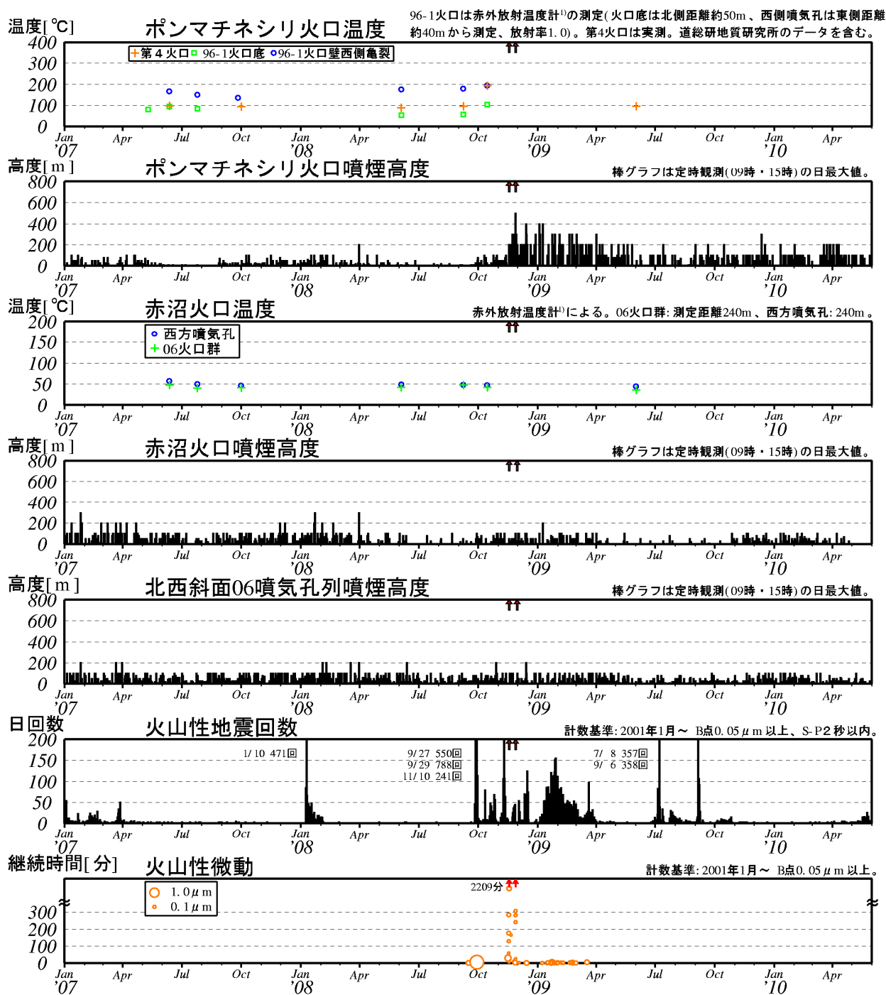
図3※ 雌阿寒岳 最近の火山活動経過図（2007年1月～2010年5月） ↑印は噴火
