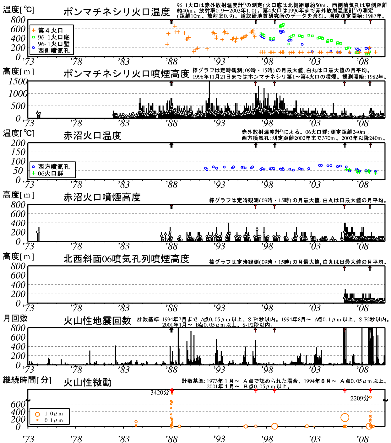
図 2 ※ 雌阿寒岳 長期の火山活動経過図 (1973 年 1 月～2010 年 5 月) ↑印は噴火
