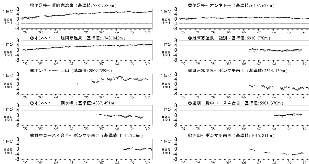
図 7 ※ 雌阿寒岳 GPS 連続観測による基線長変化（2001 年 10 月～2010 年 5 月）
