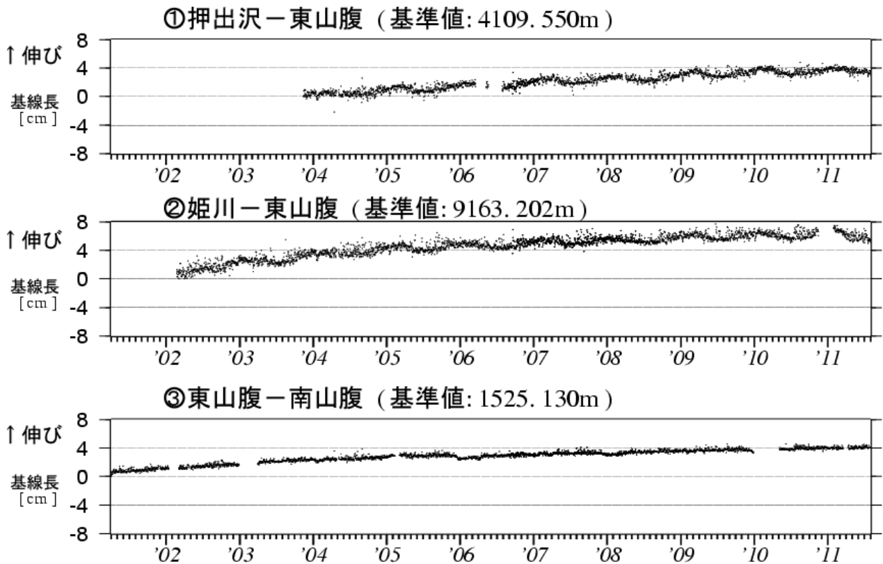
図 4 北海道駒ヶ岳 GPS 連続観測による基線長変化（2001 年 4 月～2011 年 7 月）
