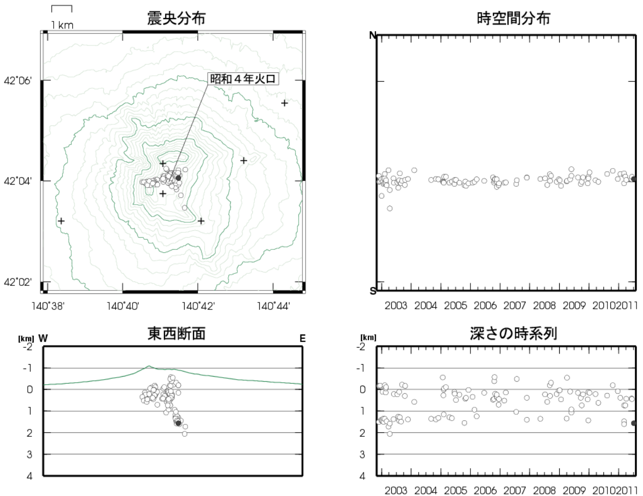
図 3※ 北海道駒ヶ岳 火山性地震の震源分布(2002 年 11 月～2011 年 7 月)
