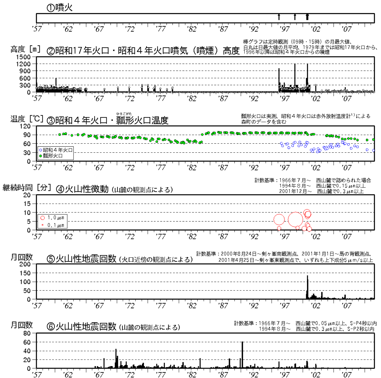
図 1 ※ 北海道駒ヶ岳 火山活動経過図（1957 年 1 月～2011 年 7 月）
