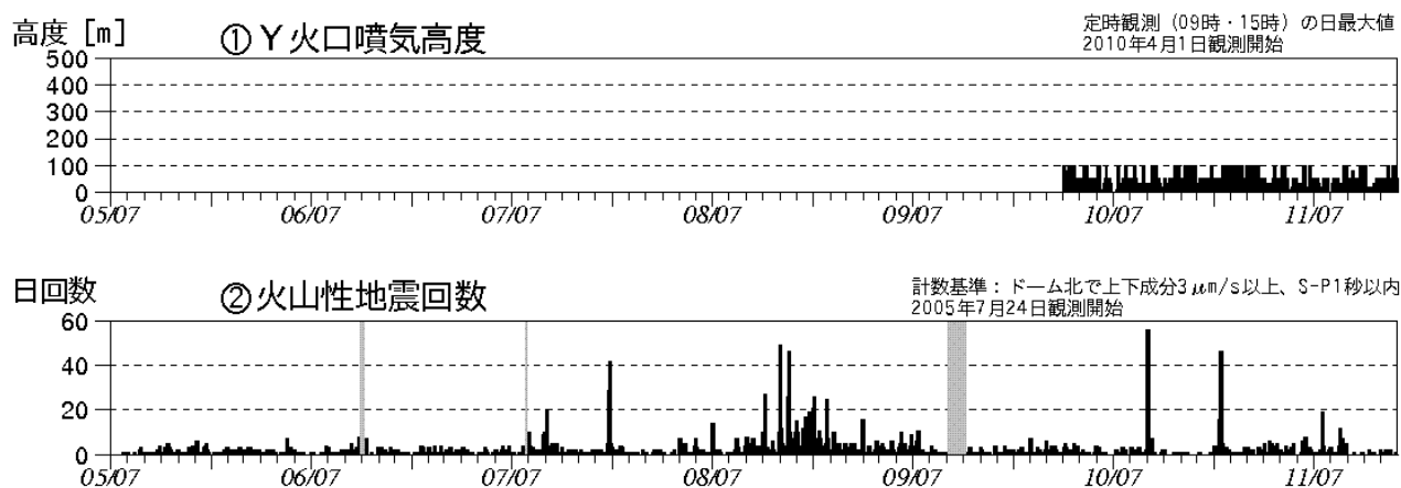
図 1 恵山 火山活動経過図（2005 年 7 月～2011 年 11 月）
