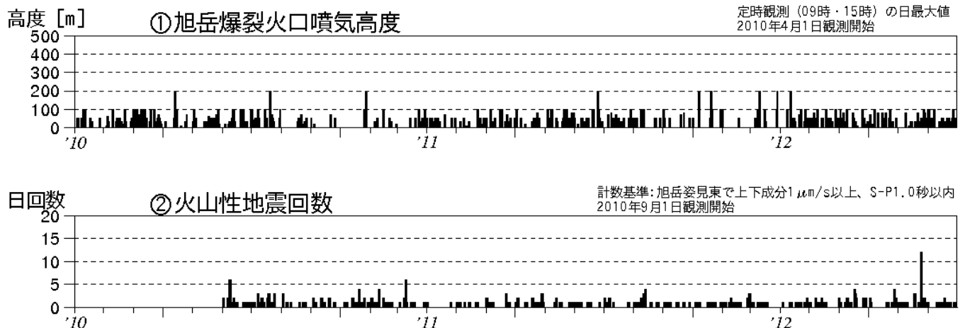
図1 大雪山 火山活動経過図（2010年4月～2012年9月）
