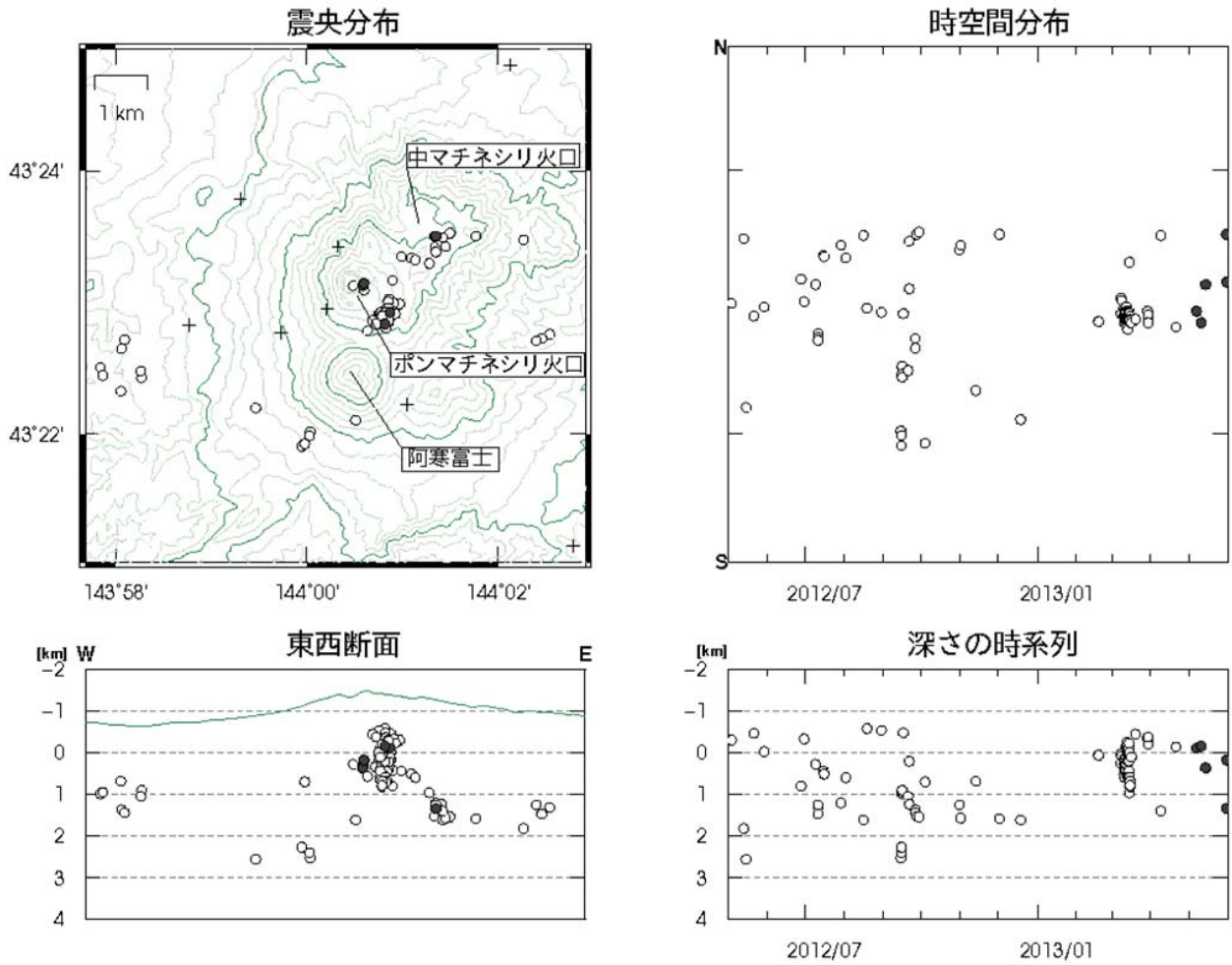
図 4 雌阿寒岳 火山性地震の震源分布（2012年5月～2013年5月）
