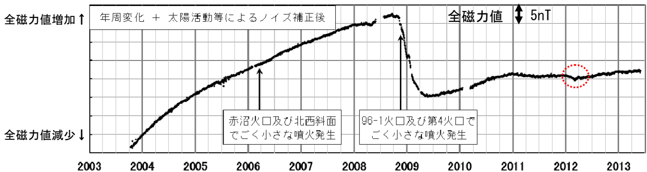
図3 雌阿寒岳 全磁力連続観測 1) による連続観測点MEA（上図中◎）の全磁力値変化（2003年10月16日～2013年5月28日）
