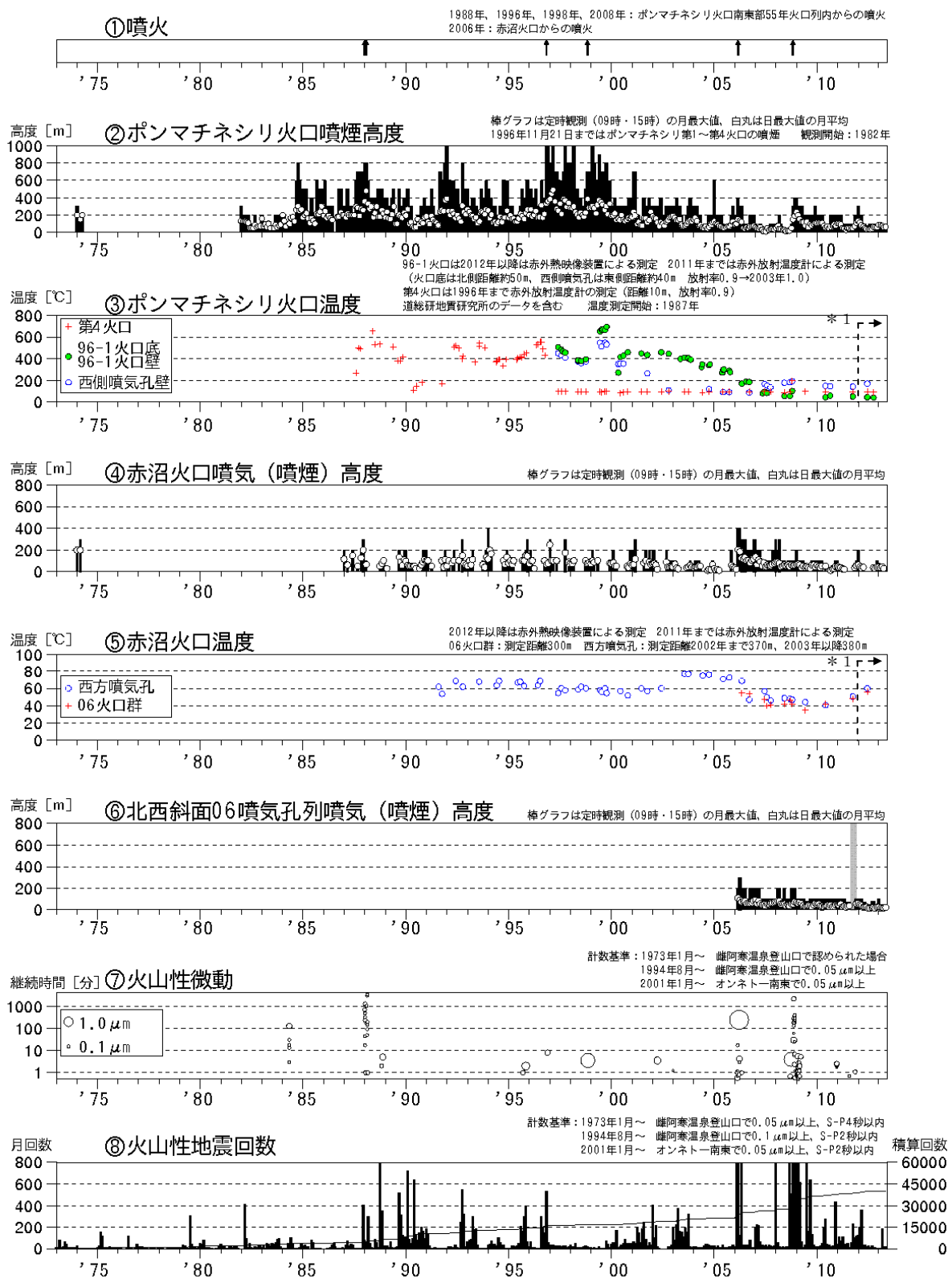
図 1 雌阿寒岳 火山活動経過図（1973年1月～2013年5月）
