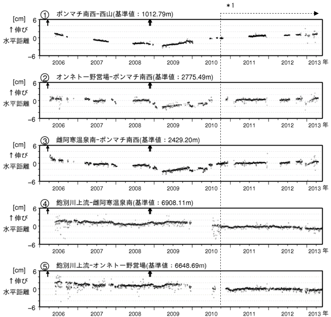
図5 雌阿寒岳 GPS連続観測による水平距離変化（2006年5月～2013年5月） ・グラフの空白部分は欠測を示し、GPS基線①～⑤は図6の①～⑤に対応しています ＊ 1：2010年10月以降のデータについては、解析方法を改良して精度を向上させています
