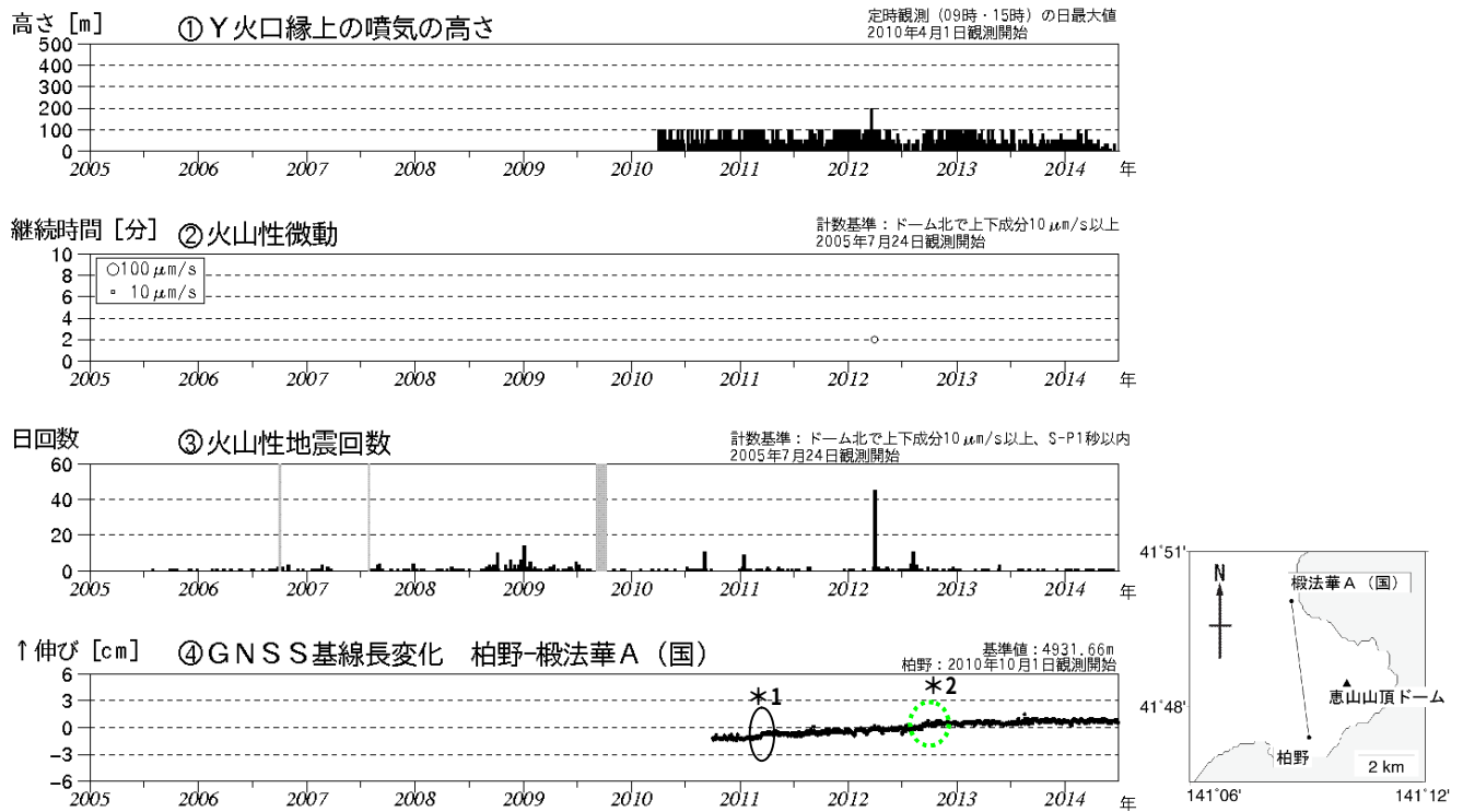
図1 恵山 火山活動経過図（2005年7月～2014年6月）、GNSS連続観測点配置図
