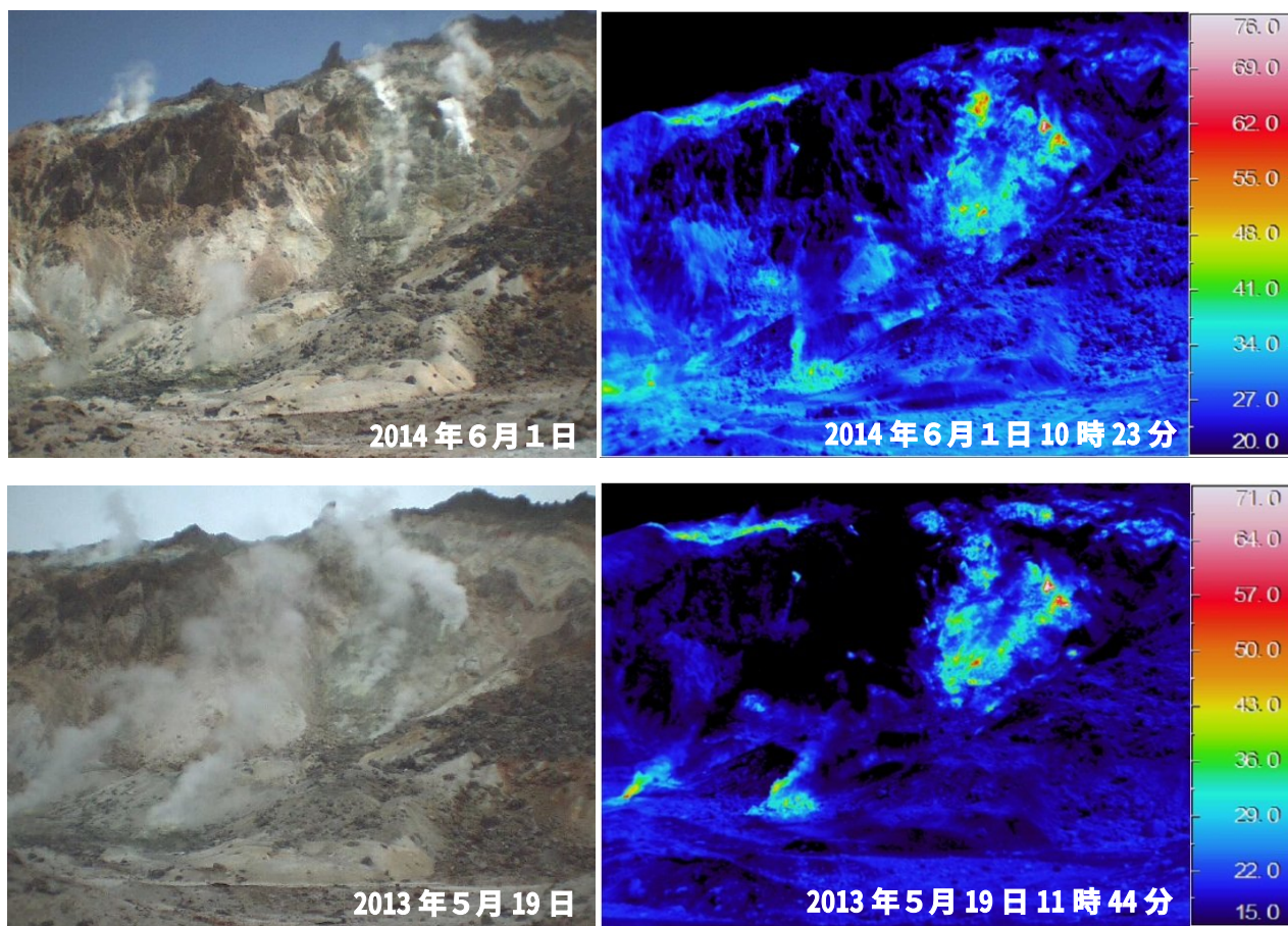
図 6 恵山 Y 火口内の地表面温度分布（図 3 - ③から撮影）
