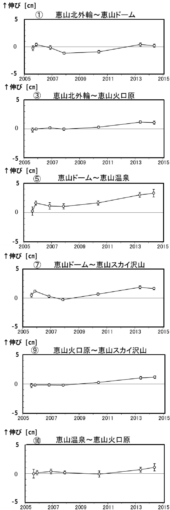
図 7 恵山 GNSS繰り返し観測による基線長変化（2005 年 8 月～2014 年 6 月）
