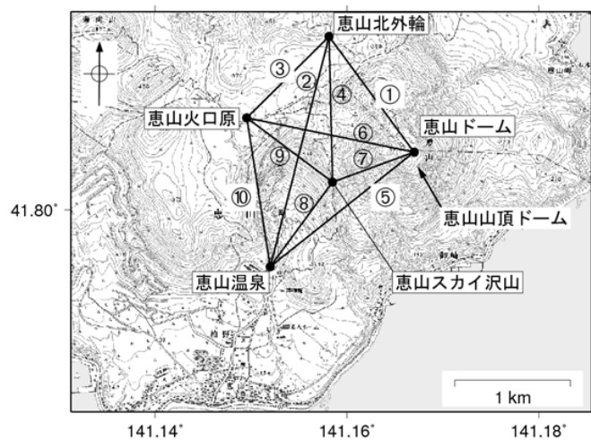
図 7 恵山 GNSS繰り返し観測による基線長変化（2005 年 8 月～2014 年 6 月）
