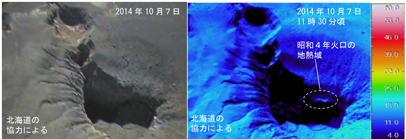
図6 北海道駒ヶ岳 赤外熱映像装置 1) による昭和4年火口内の地表面温度分布 北側上空（図3の①の矢印方向）から撮影
