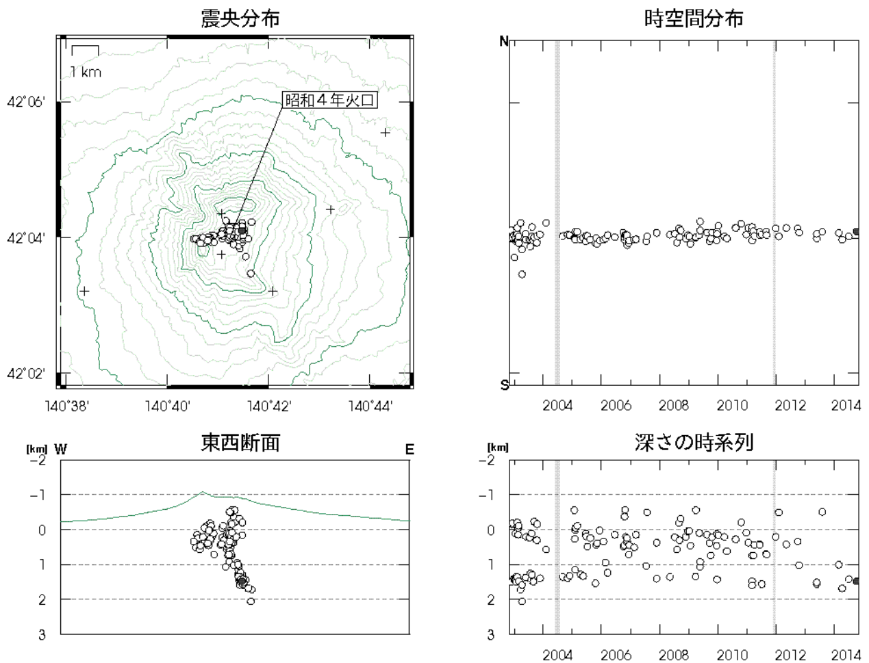
図7 北海道駒ヶ岳 火山性地震の震源分布（2002年12月～2014年10月） 灰色の期間は一部観測点欠測のため震源の決定数減少や精度低下が見られます ○印：2002年11月から2014年9月の震源 ●印：2014年10月の震源 ＋印：地震観測点
