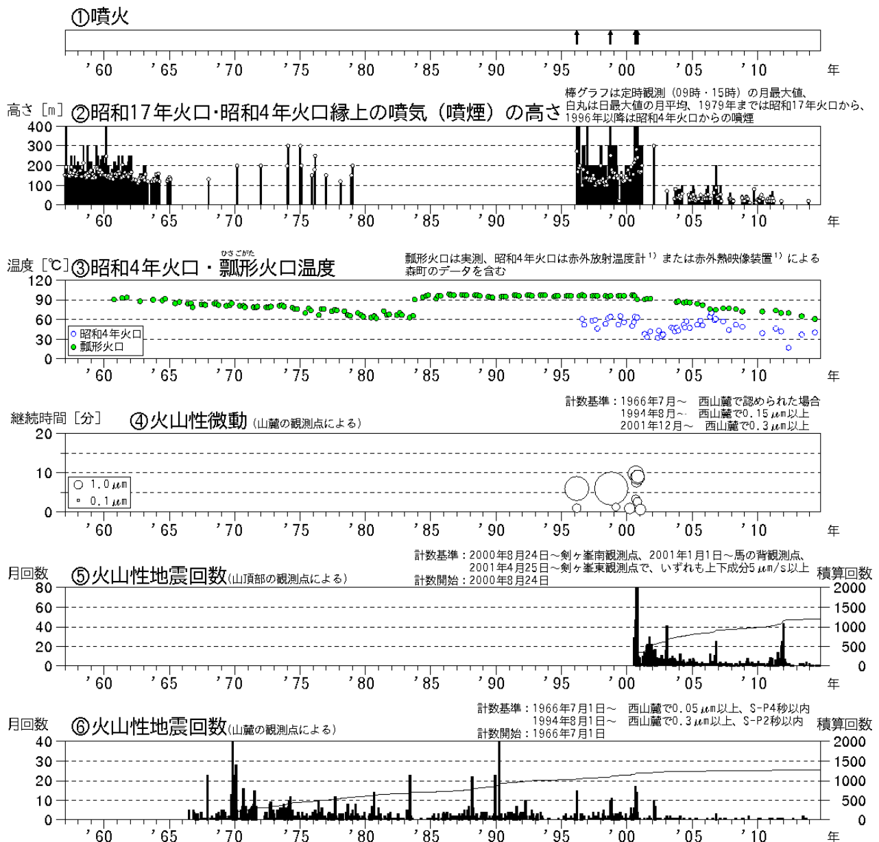
図 1 北海道駒ヶ岳 火山活動経過図（1957年 1 月～2014年10月）
