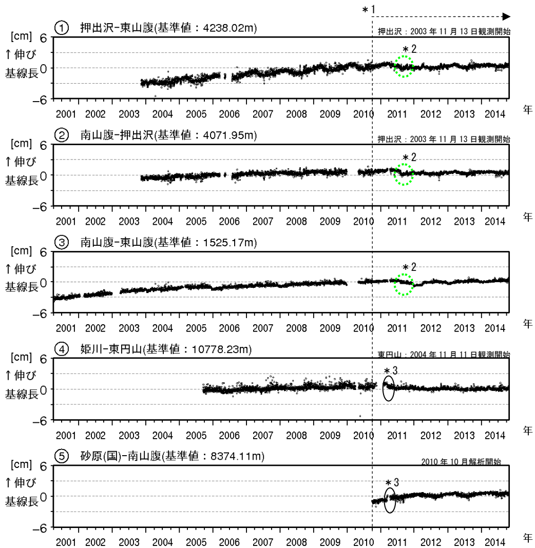
図 8 北海道駒ヶ岳 GNSS連続観測による基線長変化 (2001年4月～2014年10月)
