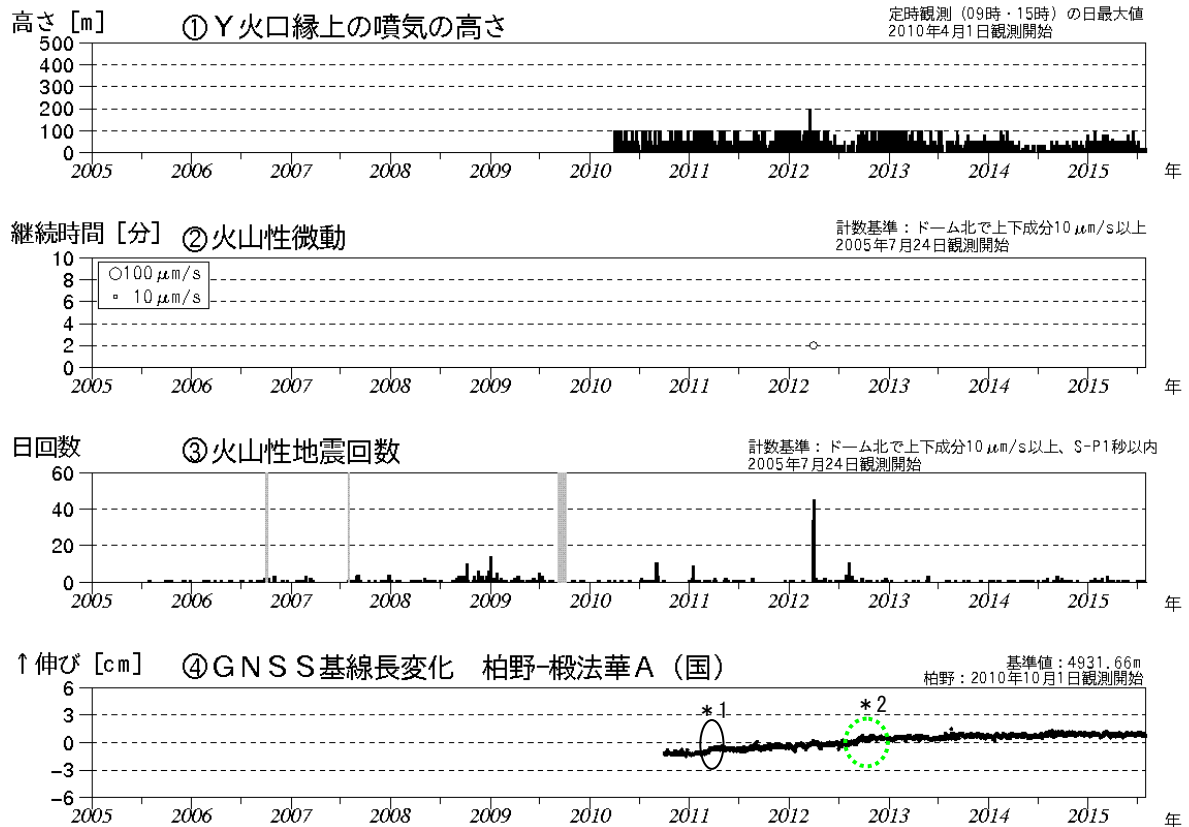
図2 恵山 火山活動経過図（2005年7月～2015年7月）
