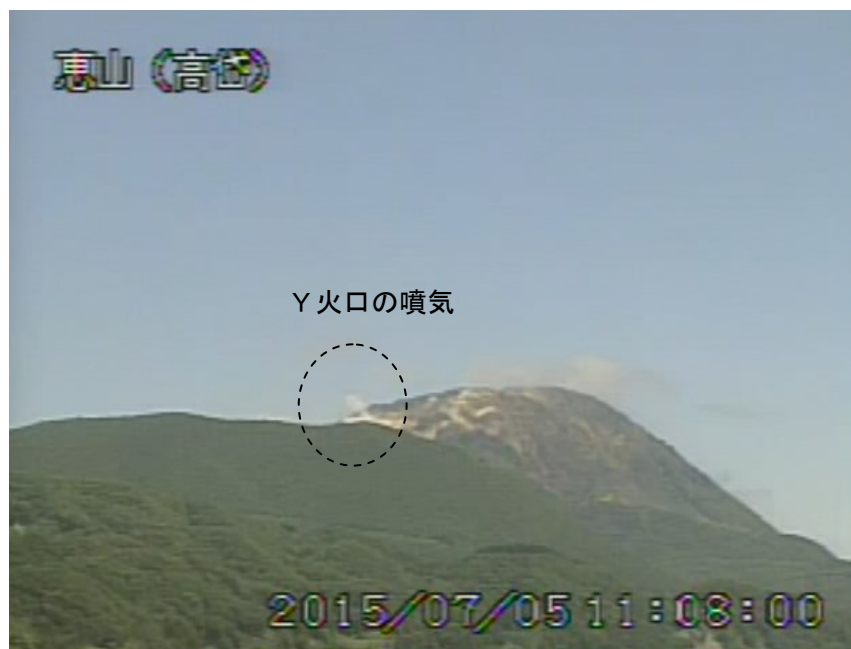
図1 恵山 西南西側から見た山頂部の状況（7月5日、 ただい 高岱遠望カメラによる）
