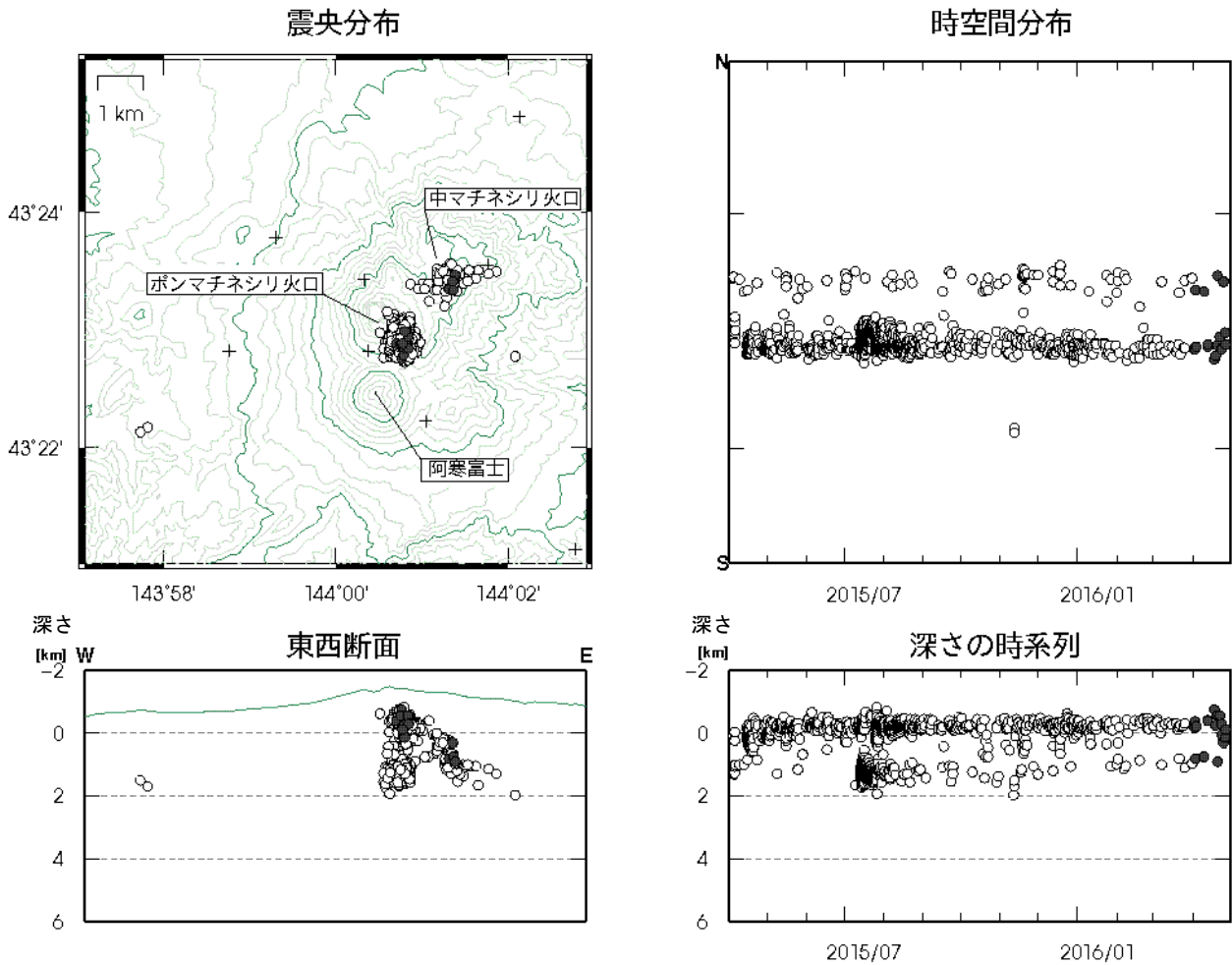
図 6 雌阿寒岳 火山性地震の震源分布（2015年4月～2016年4月）
