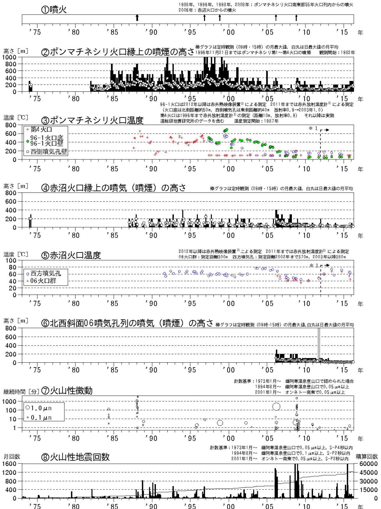
図1 雌阿寒岳 火山活動経過図（1973年1月～2016年4月）
