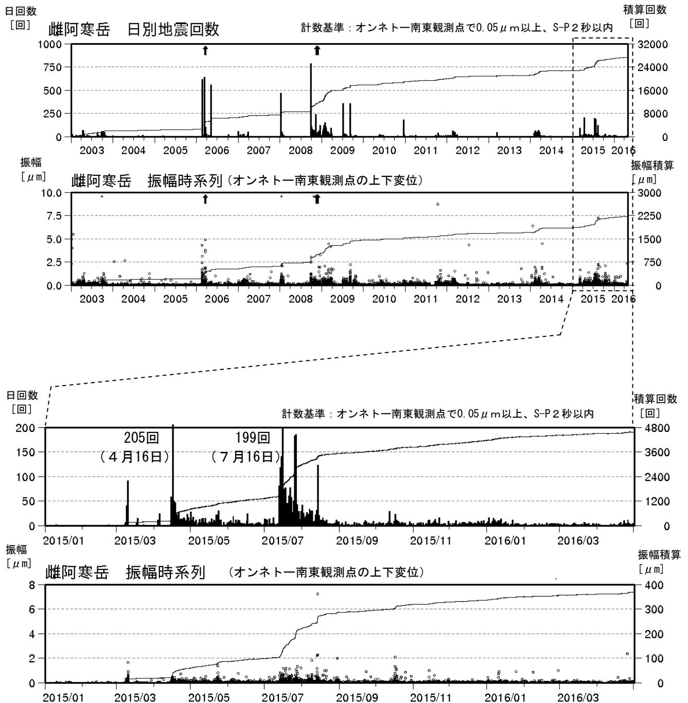
図5 雌阿寒岳 日別地震回数及び振幅時系列 上図：2003年1月1日～2016年4月30日 下図：2015年1月1日～2016年4月30日
