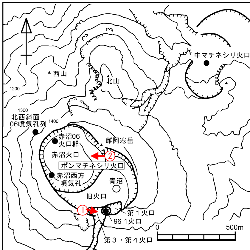
図2 雌阿寒岳 写真及び赤外熱映像の撮影方向
