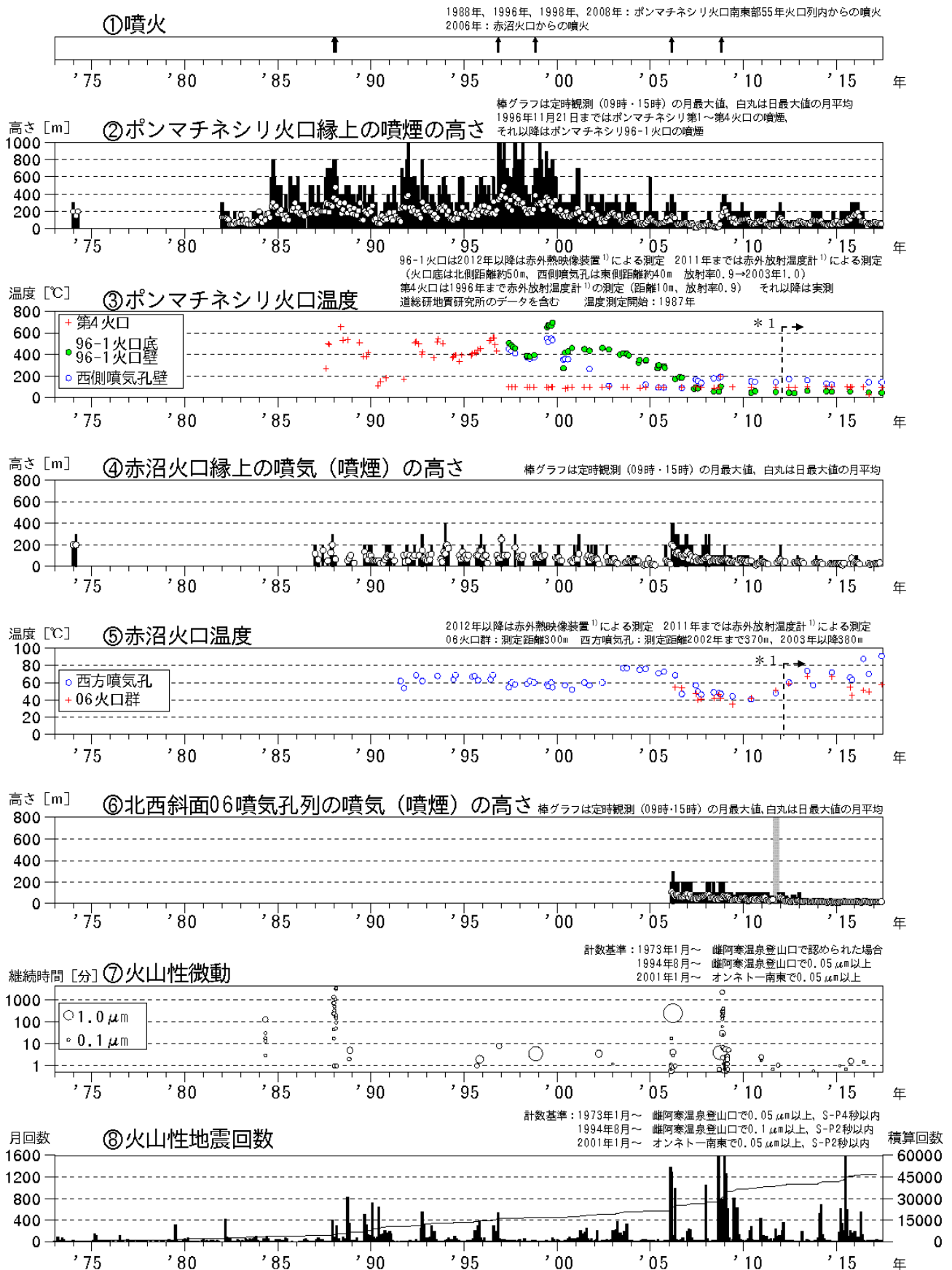
図1 雌阿寒岳 火山活動経過図（1973年1月～2017年6月）
