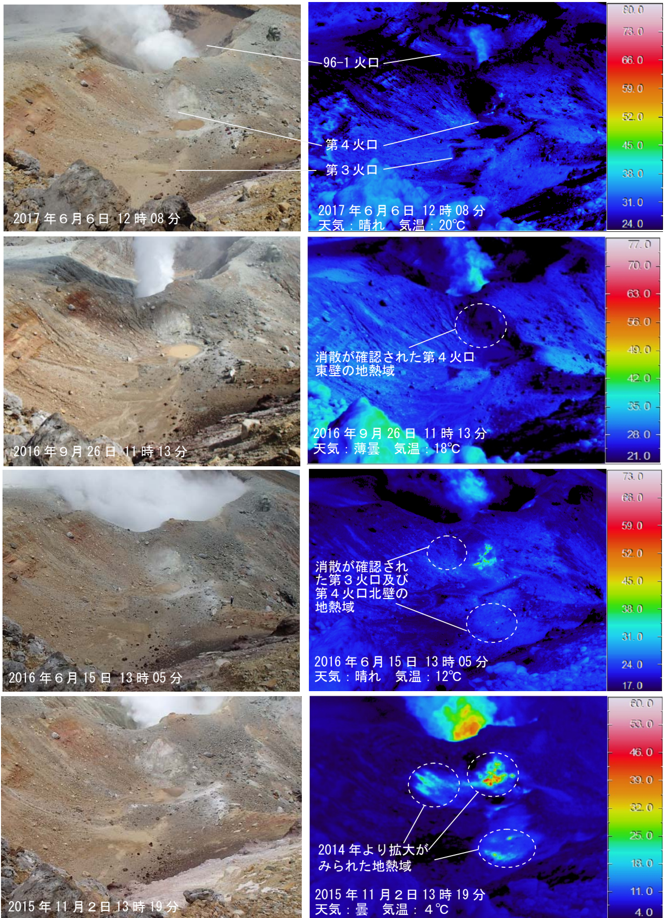
図4 雌阿寒岳 赤外熱映像装置によるポンマチネシリ第3火口及び第4火口の地表面温度分布及び96-1火口の噴煙（図2中の①から撮影）
