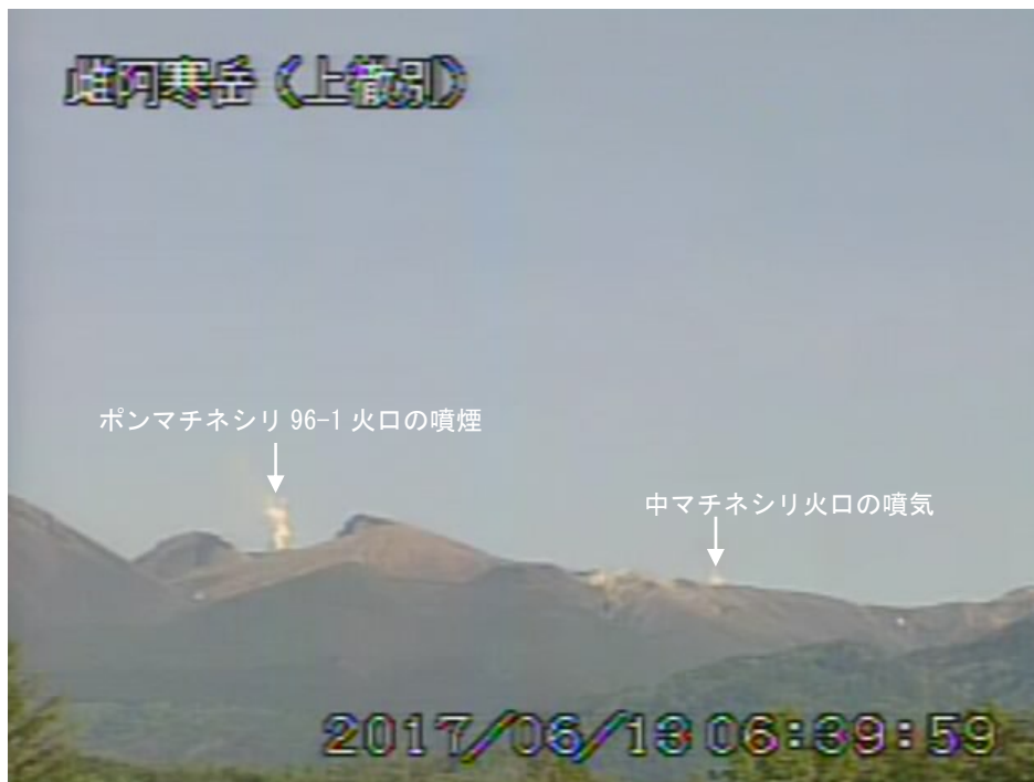
図3 雌阿寒岳 南東側から見た山体の状況 (6月13日、上徹別監視カメラによる)
