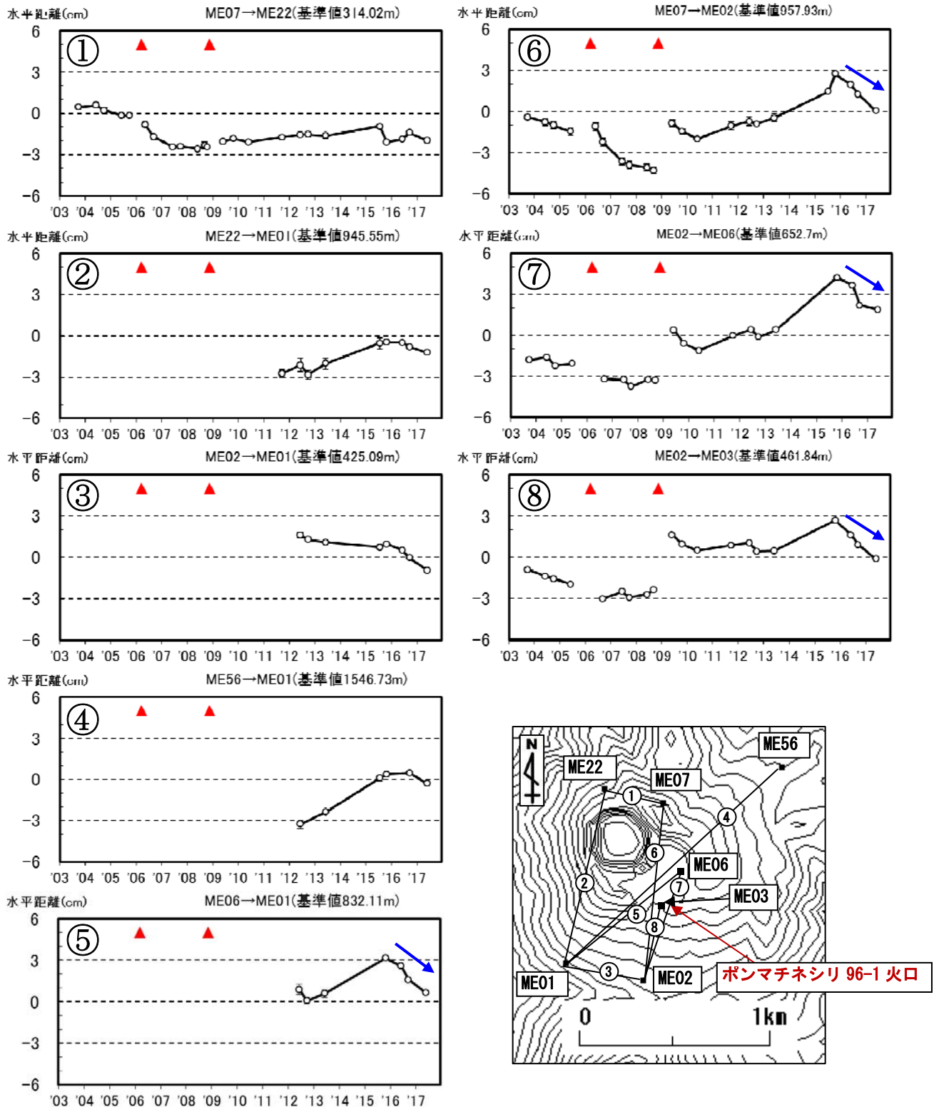
図 10 雌阿寒岳 GNSS 繰り返し観測によるポンマチネシリ火口付近の基線長変化 (2003 年 7 月～2017 年 6 月)
