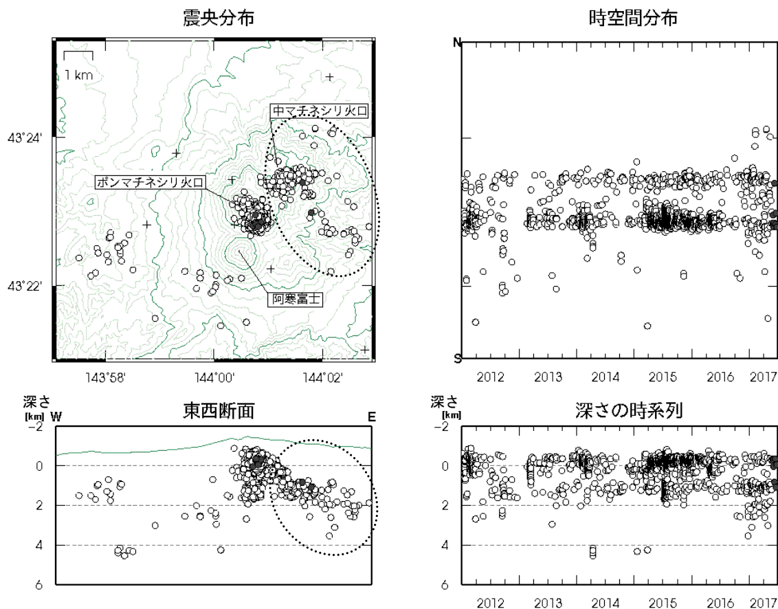
図 8 雌阿寒岳 火山性地震の震源分布（2012年1月～2017年6月）
