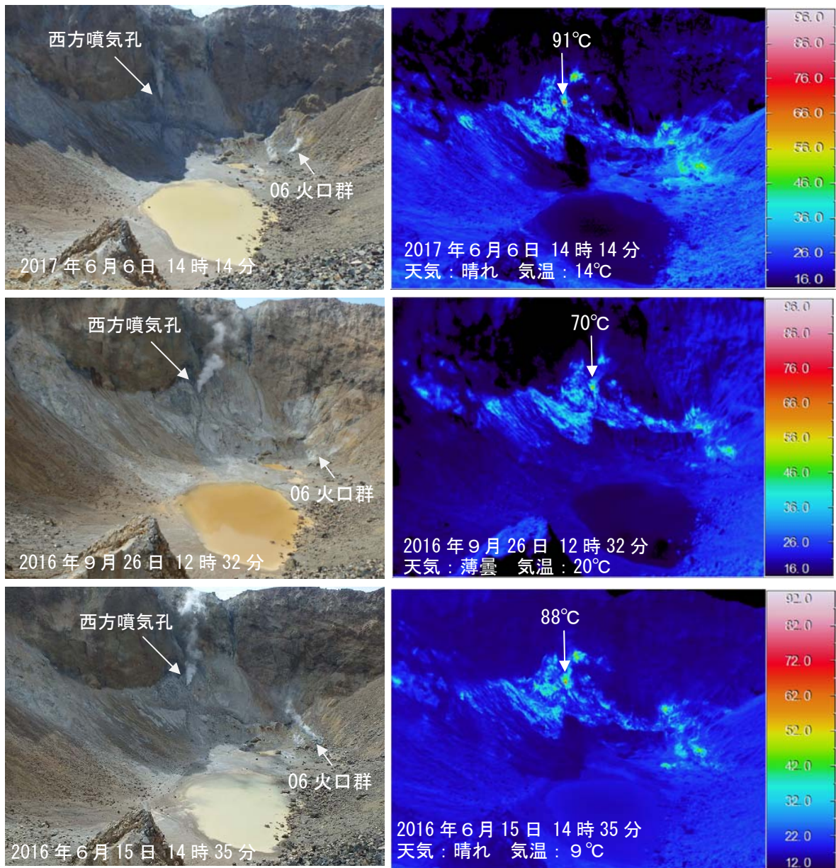
図5 雌阿寒岳 赤外熱映像装置によるポンマチネシリ赤沼火口の地表面温度分布 (図2中の②から撮影)
