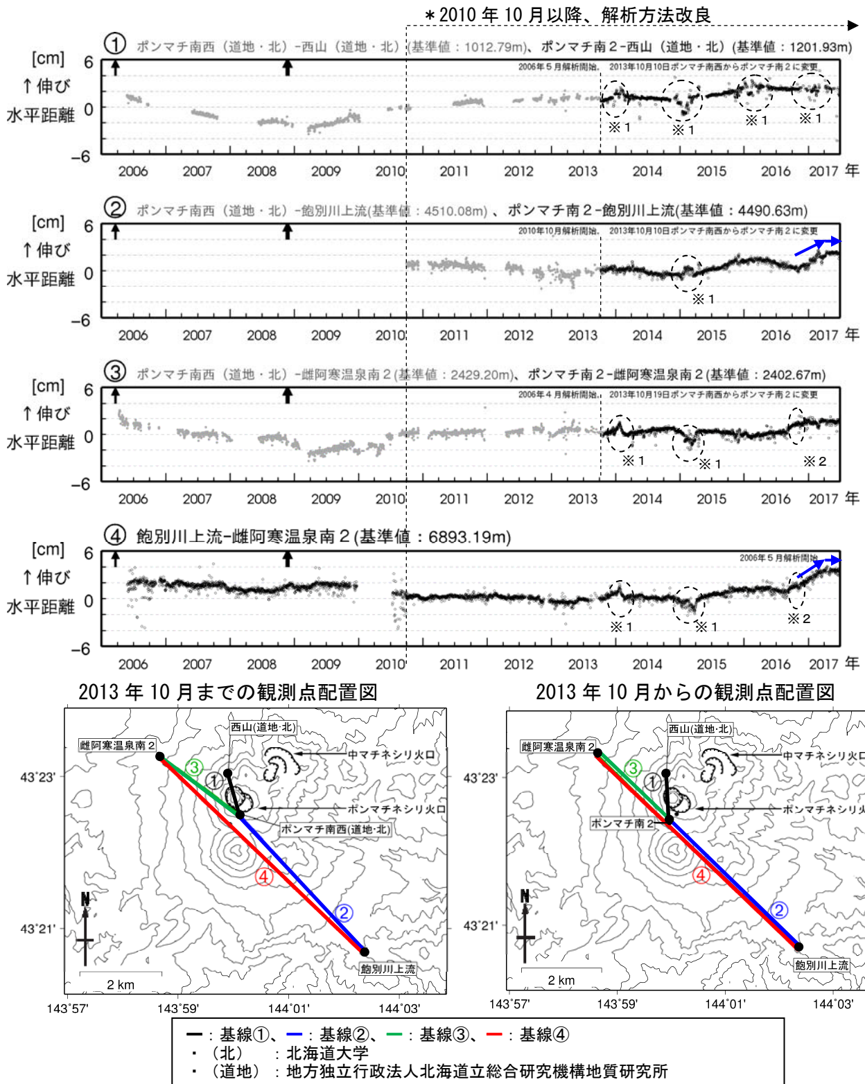
図 9 雌阿寒岳 GNSS連続観測による水平距離変化（2006年4月～2017年6月）及び観測点配置図
