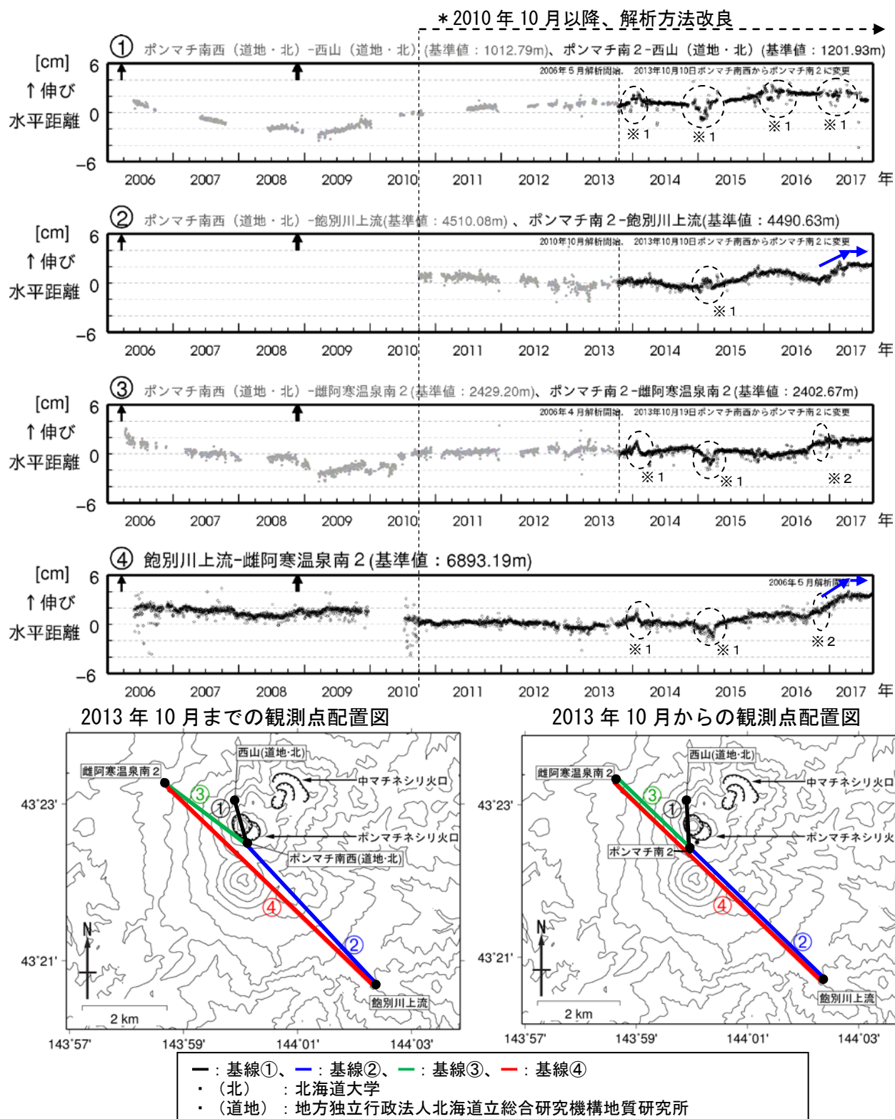
図 7 雌阿寒岳 GNSS連続観測による水平距離変化（2006年4月～2017年8月）及び観測点配置図
