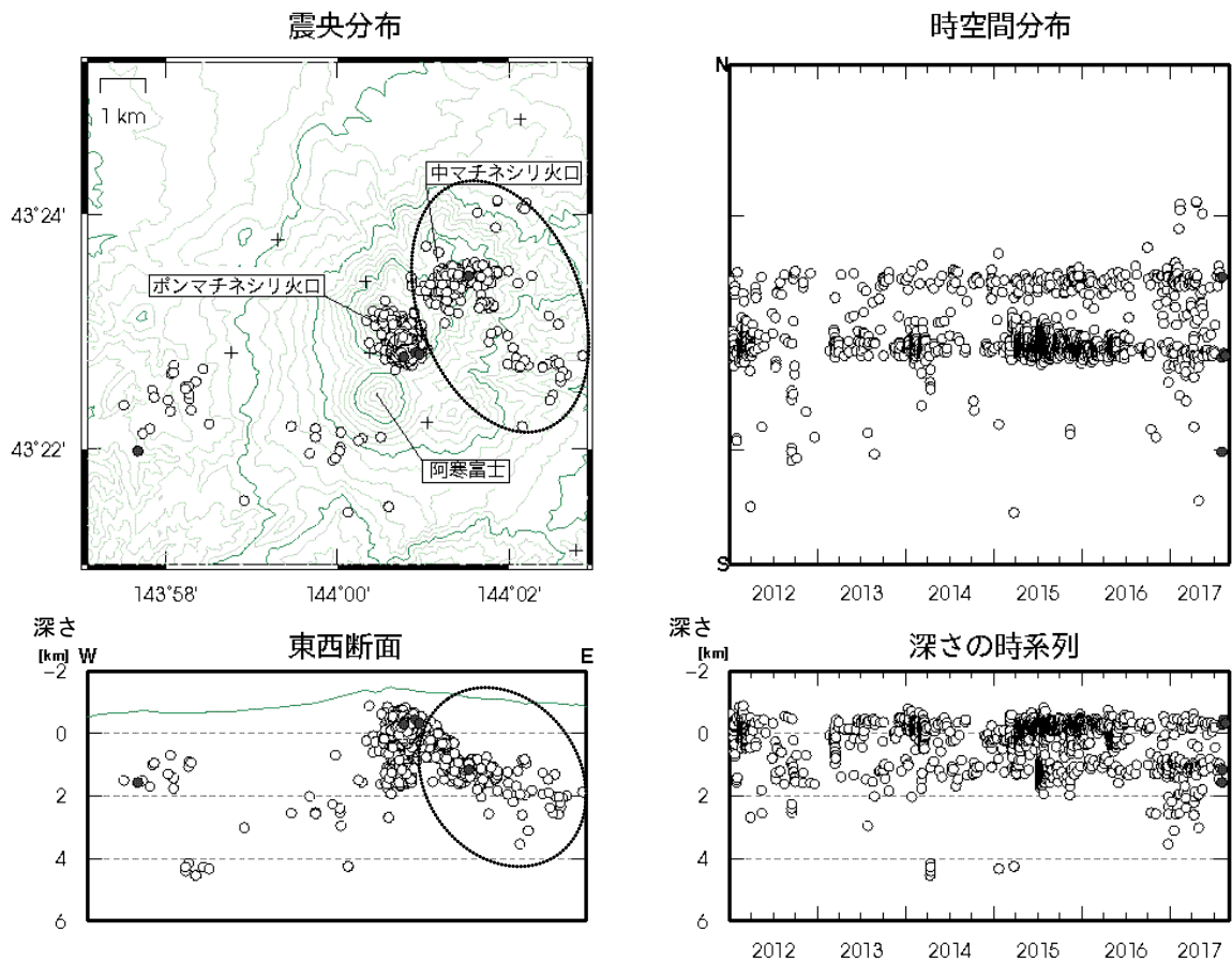
図6 雌阿寒岳 火山性地震の震源分布（2012年1月～2017年8月）
