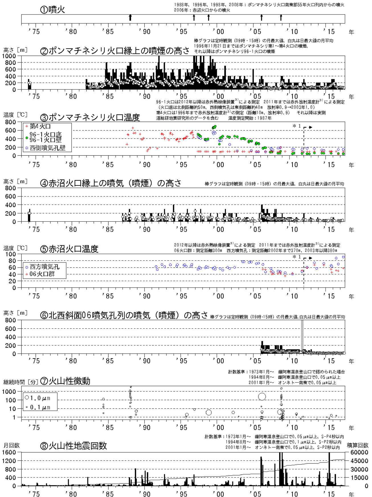
図1 雌阿寒岳 火山活動経過図（1973年1月～2017年8月）
