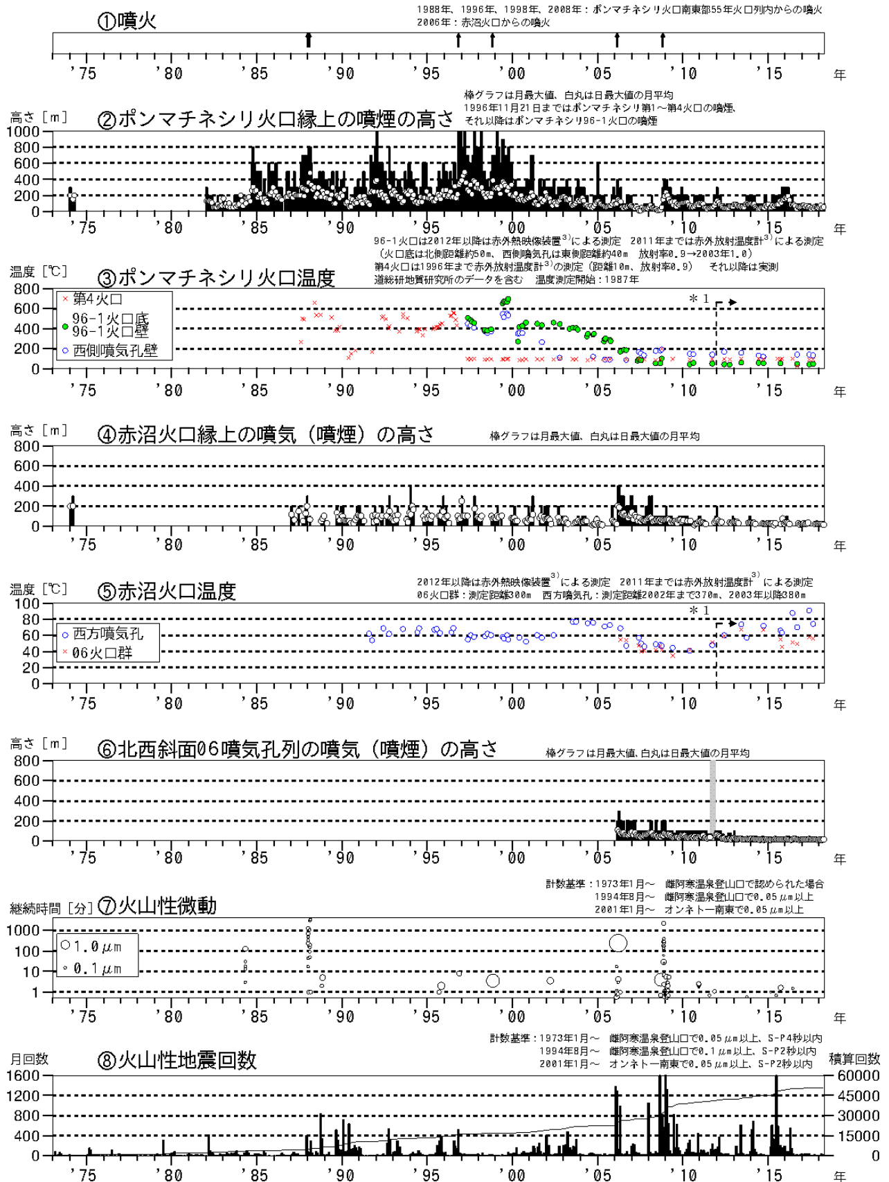
図1 雌阿寒岳 火山活動経過図（1973年1月～2018年4月）
