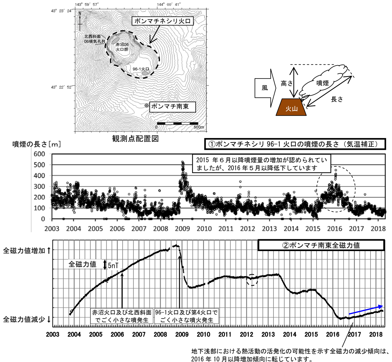
図 4 雌阿寒岳 噴煙の長さと全磁力の比較及び全磁力観測点配置図
