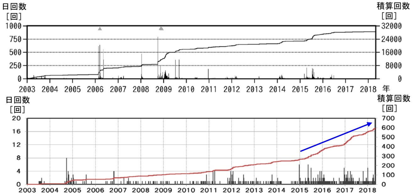
図5 雌阿寒岳 火山性地震の日回数及び積算回数推移（2003年1月～2018年4月）
