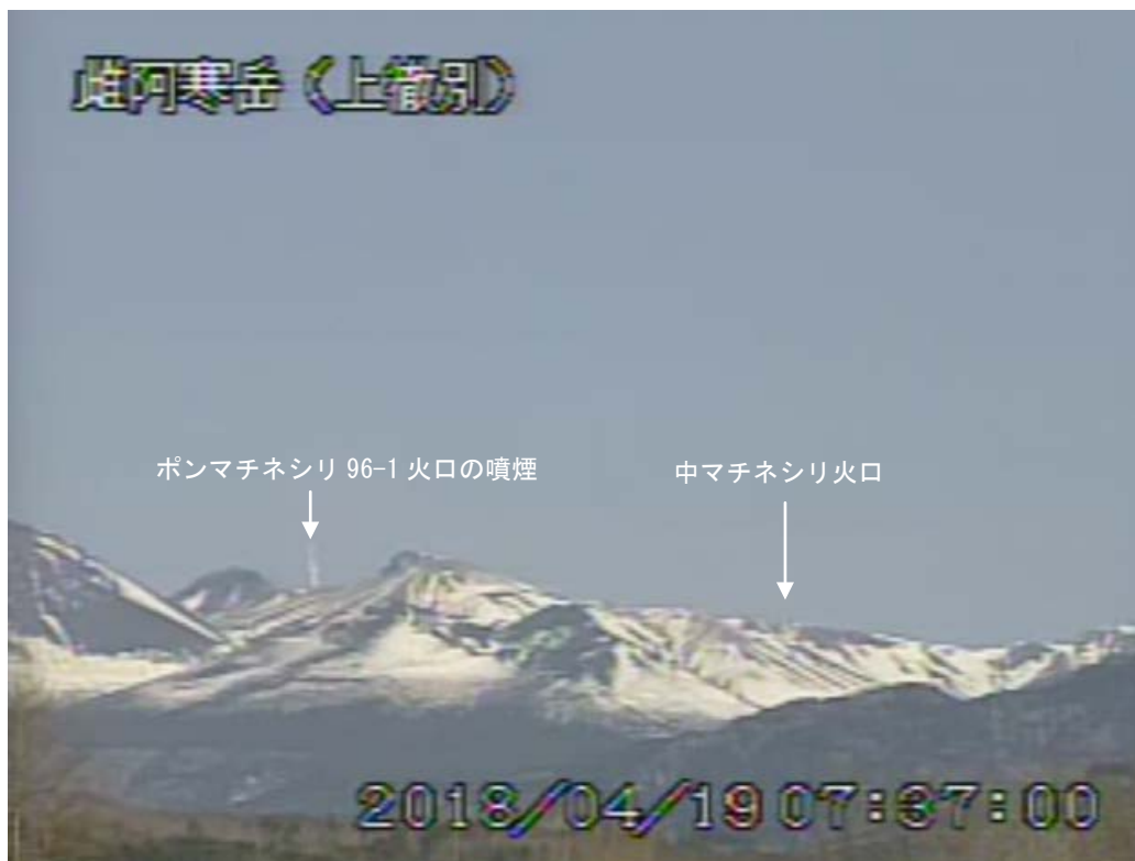
図3 雌阿寒岳 南東側から見た山体の状況 （4月19日、上徹別監視カメラによる）
