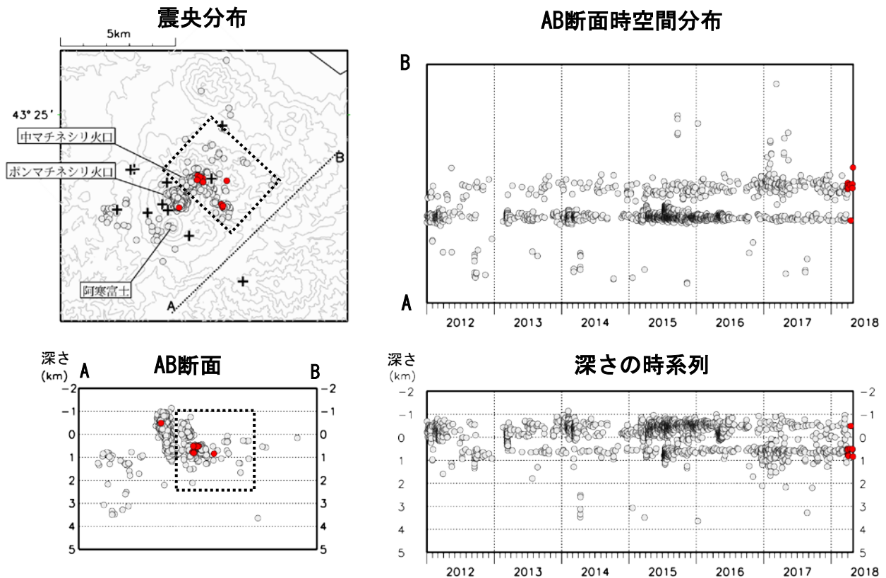
図6 雌阿寒岳 火山性地震の震源分布（2012年1月～2018年4月）
