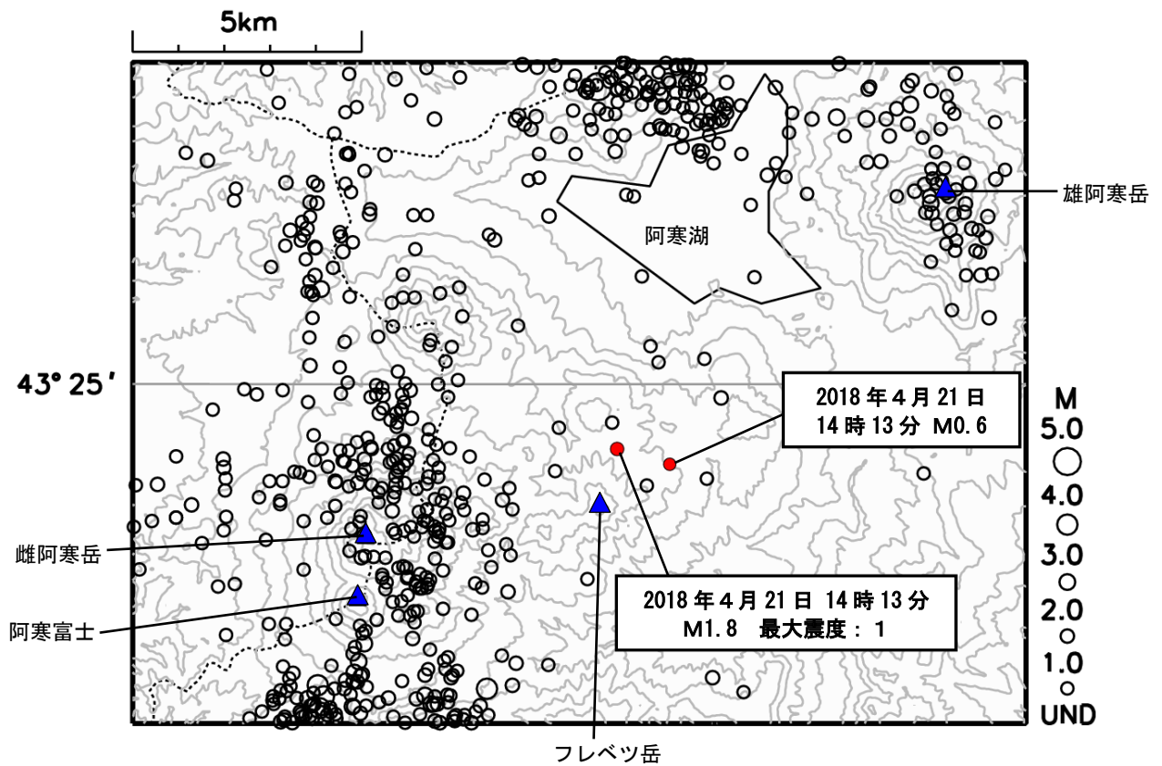
図 7 雌阿寒岳 広域地震観測網による山体周辺の地震活動 (1997年10月1日～2018年4月30日、マグニチュード0以上、深さ10km以浅) ・21日に阿寒湖温泉で震度1を観測した地震は、雌阿寒岳の東方約5kmで発生しました。
