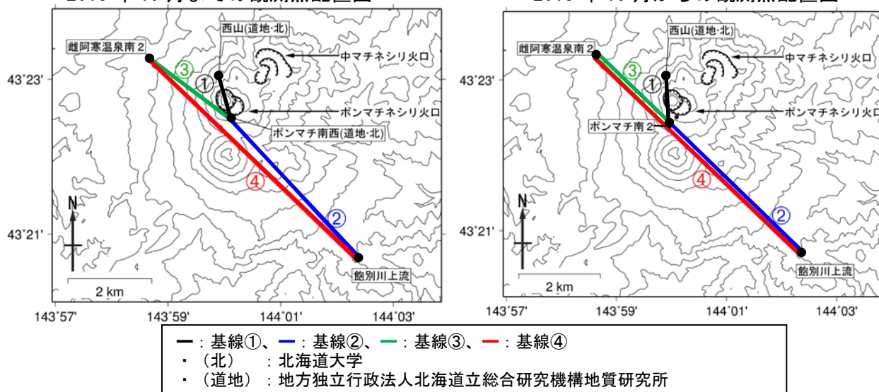
図 8 雌阿寒岳 GNSS連続観測による基線長変化（2006年 4 月～2018年 4 月）及び観測点配置図
