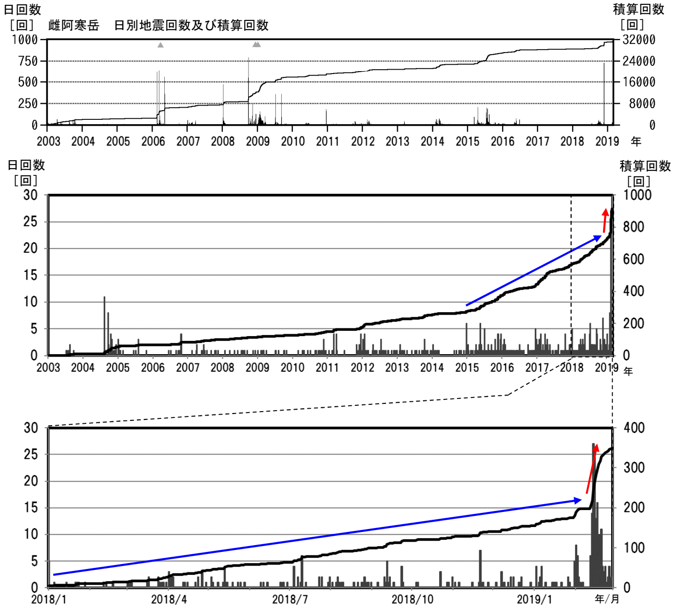
図5 雌阿寒岳 火山性地震の日別回数及び積算回数（2003年1月～2019年2月）
