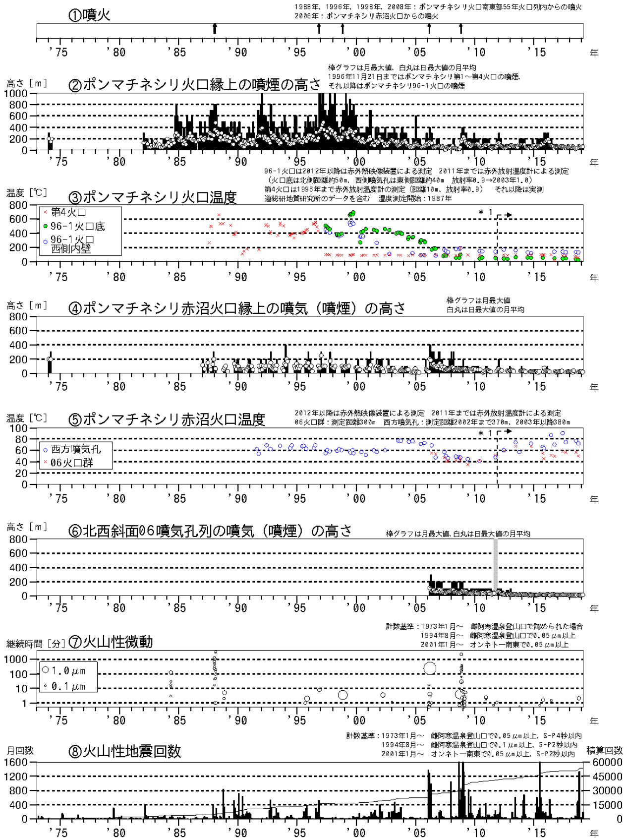
図 1 雌阿寒岳 火山活動経過図（1973年 1 月～2019年 2 月）
