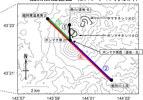
観測点配置図（2013年10月以降）
