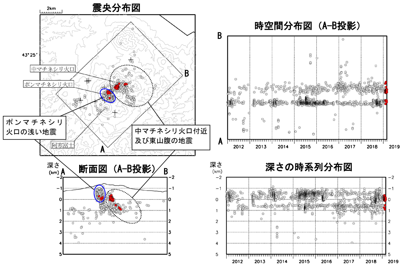
図6 雌阿寒岳 火山性地震の震源分布（2012年1月～2019年2月）
