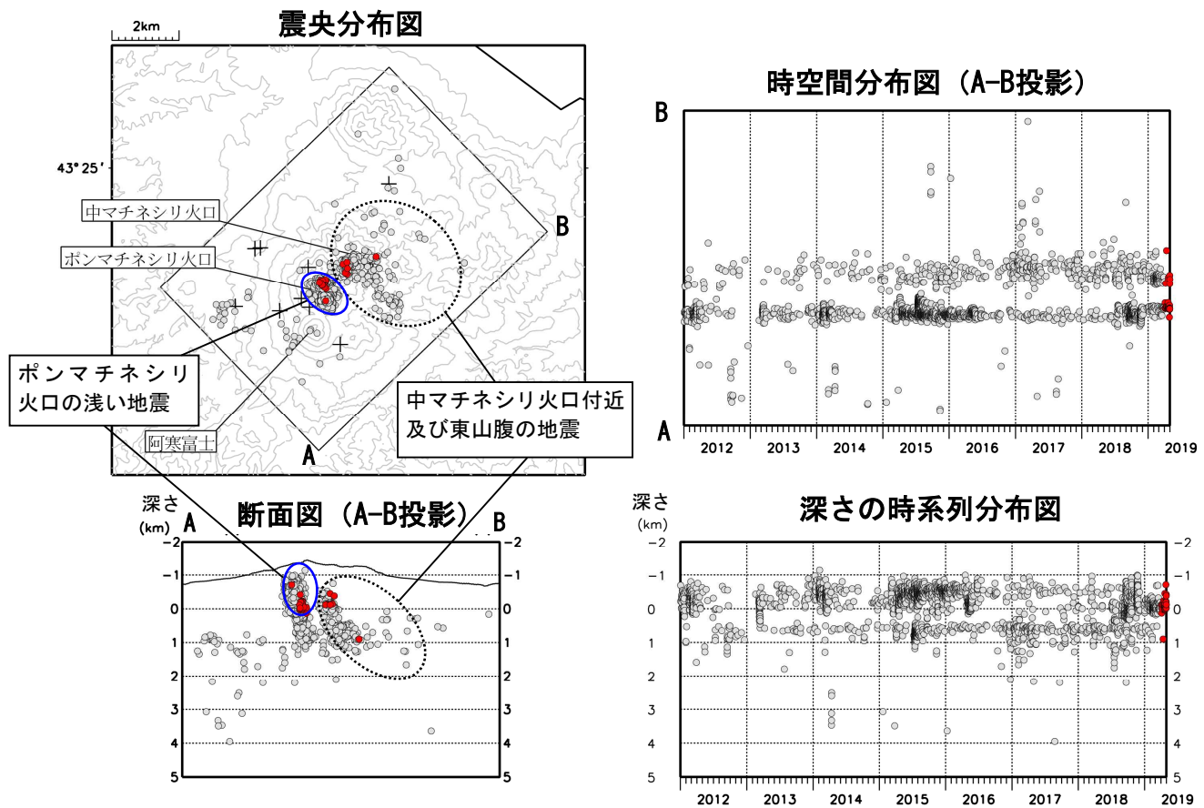
図 6 雌阿寒岳 火山性地震の震源分布（2012年1月～2019年4月）
