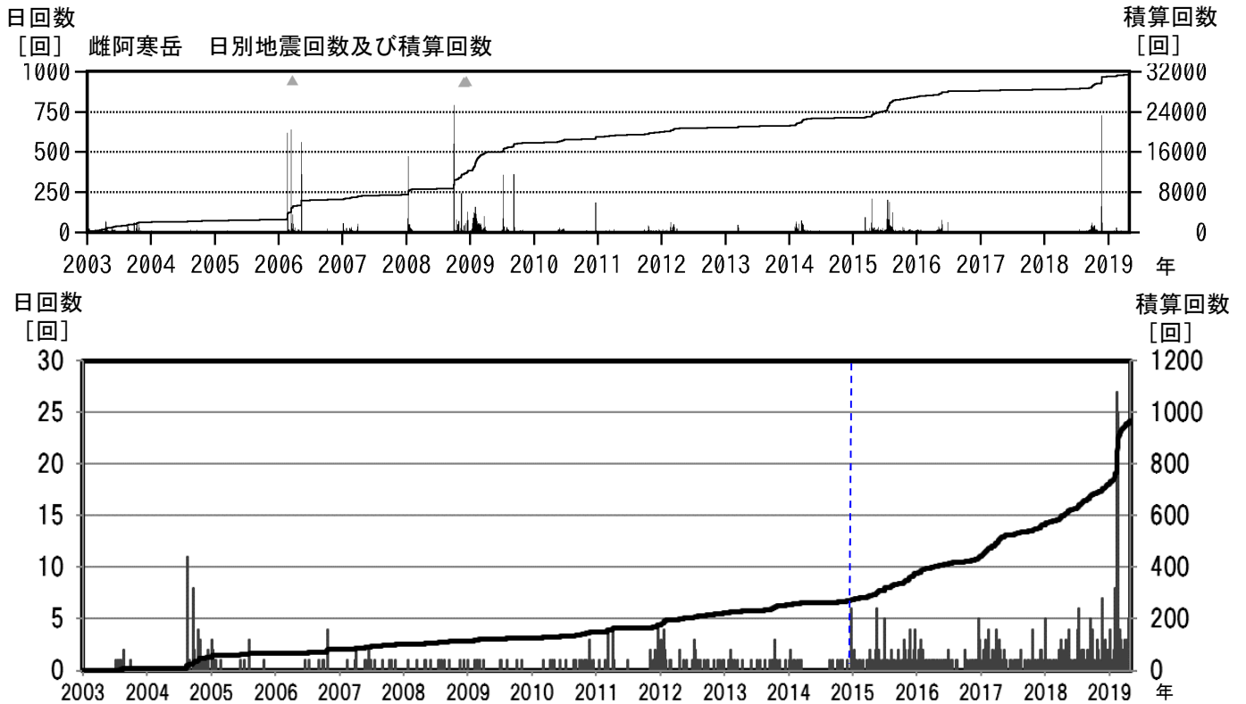
図5 雌阿寒岳 火山性地震の日別回数及び積算回数（2003年1月～2019年4月）
