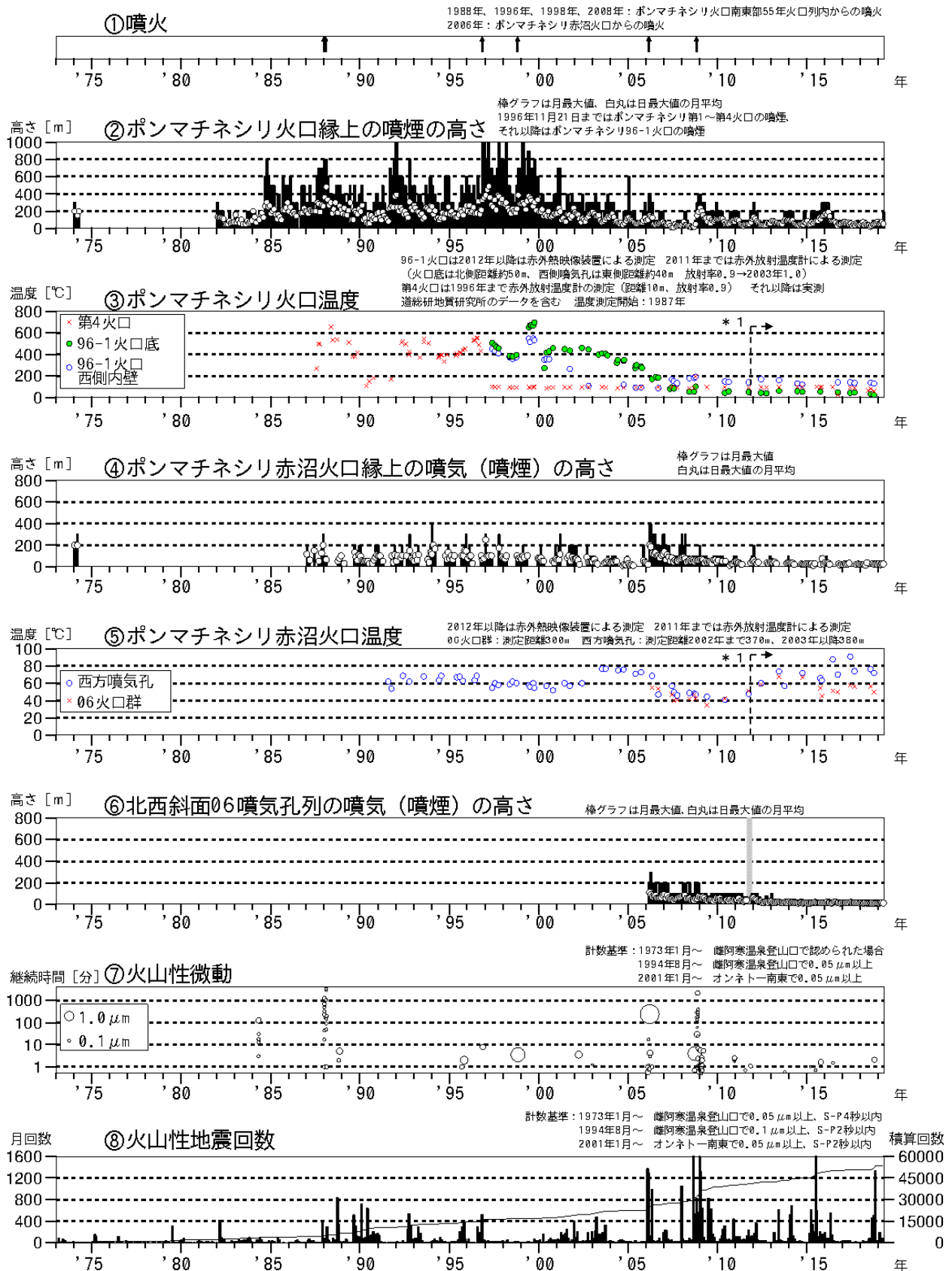
図 1 雌阿寒岳 火山活動経過図（1973年 1 月～2019年 4 月）
