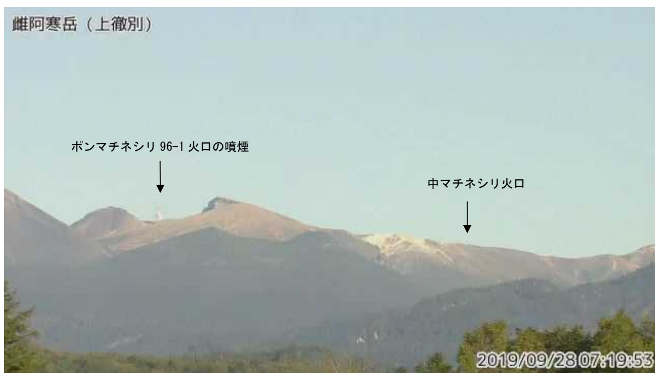
図3 雌阿寒岳 南東側から見た山体の状況 （9月28日、上徹別監視カメラによる）
