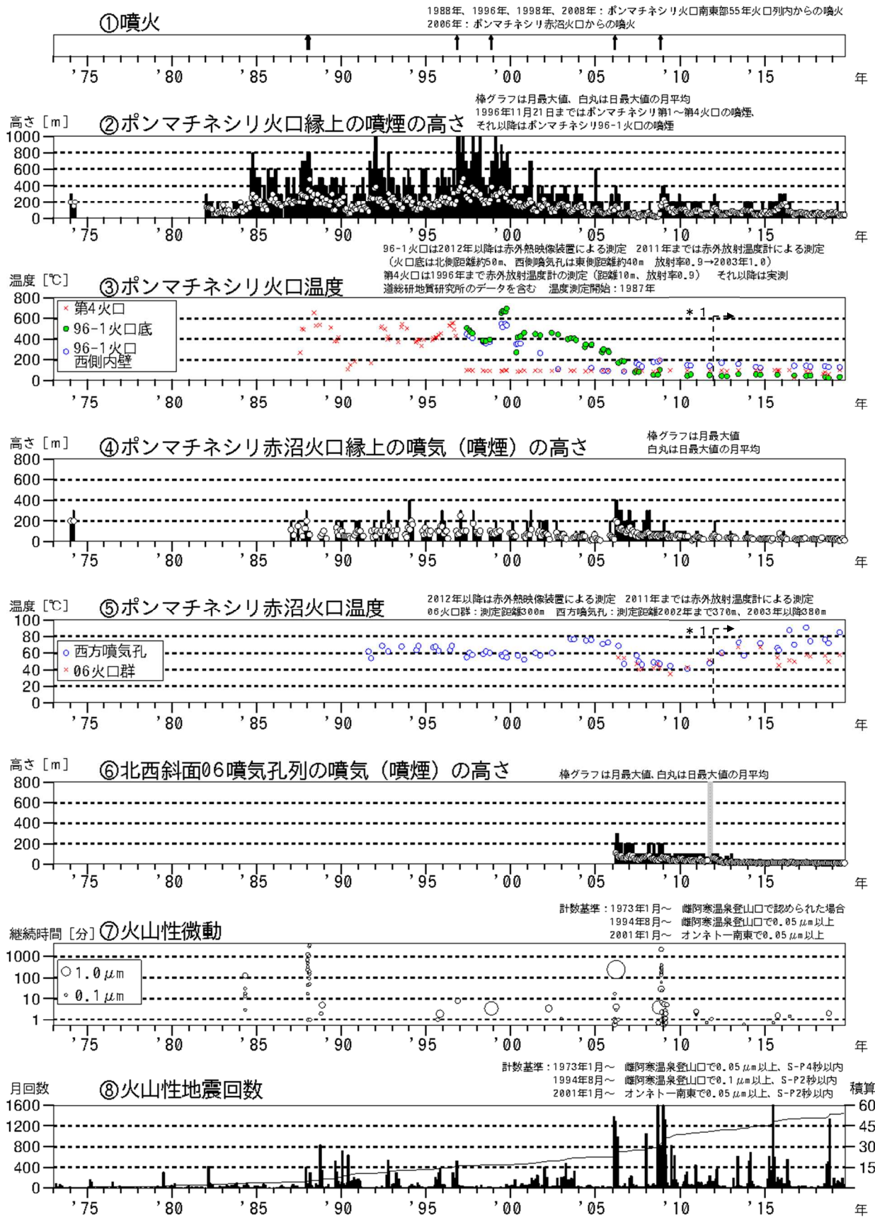
図1 雌阿寒岳 火山活動経過図（1973年1月～2019年9月）
