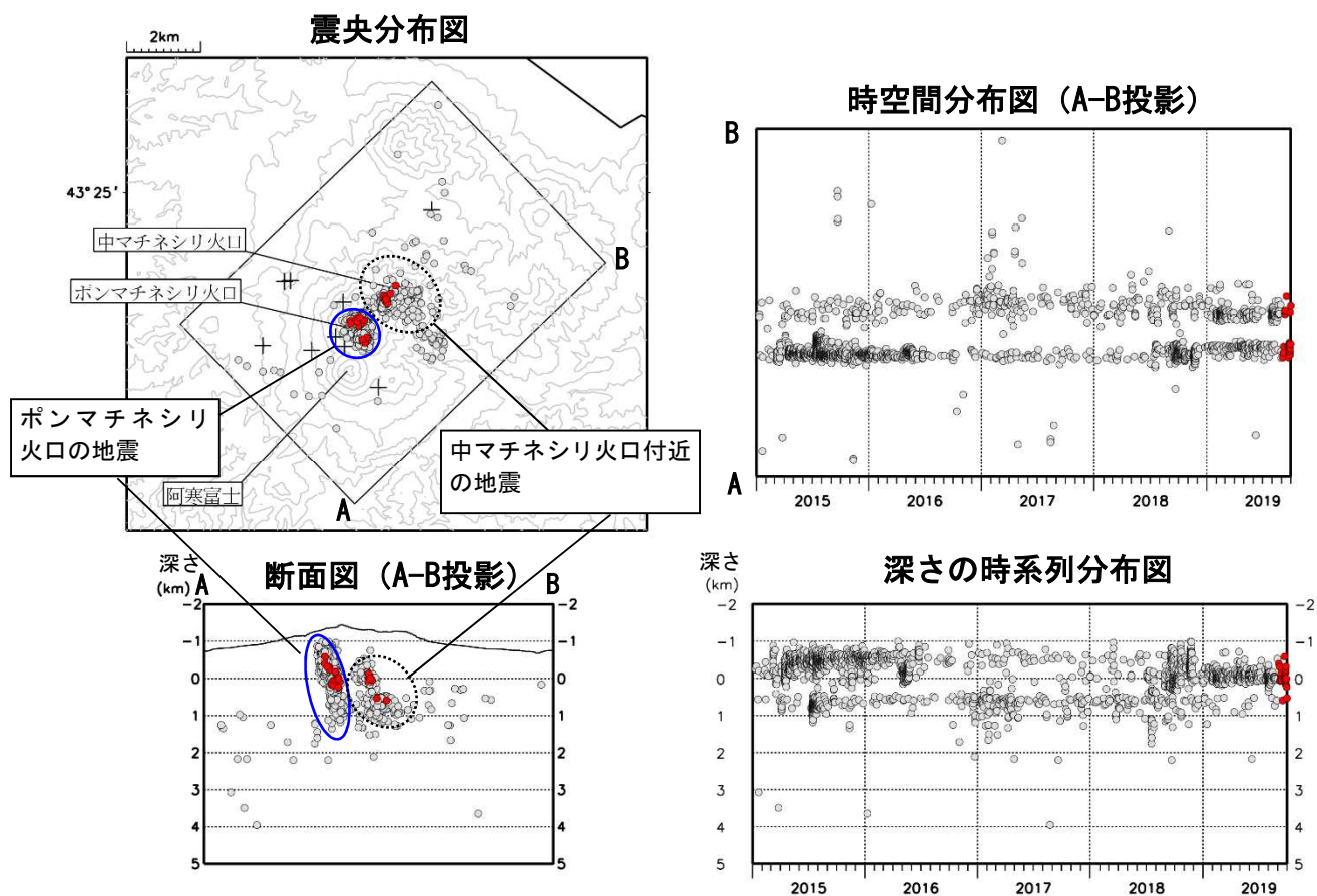
図6 雌阿寒岳 火山性地震の震源分布（2015年1月～2019年9月）
