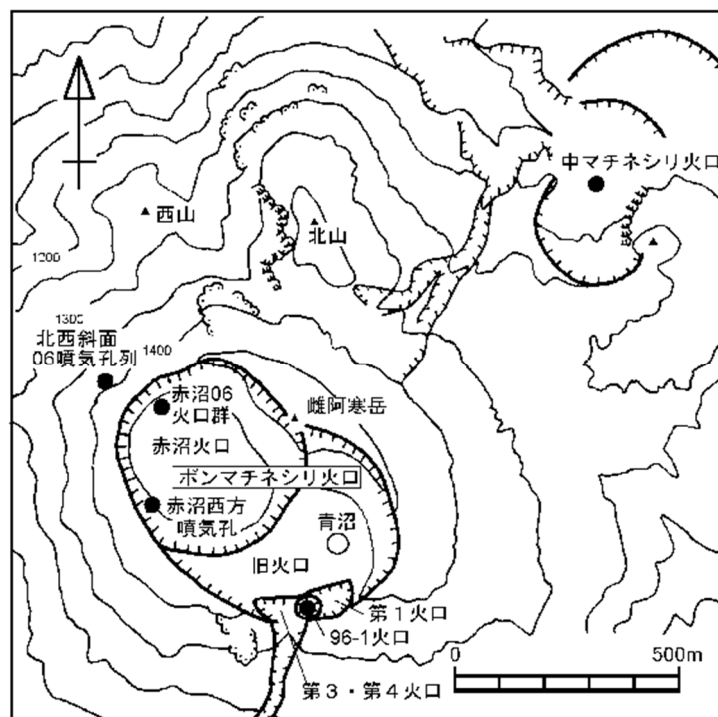
図2 雌阿寒岳 火口周辺図
