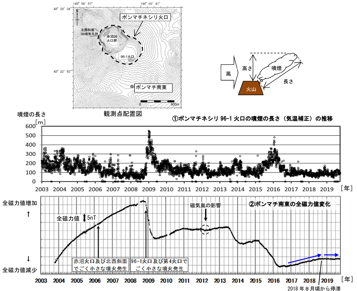
図4 雌阿寒岳 ポンマチネシリ96-1火口の噴煙の長さ と全磁力の比較及び全磁力観測点配置図
