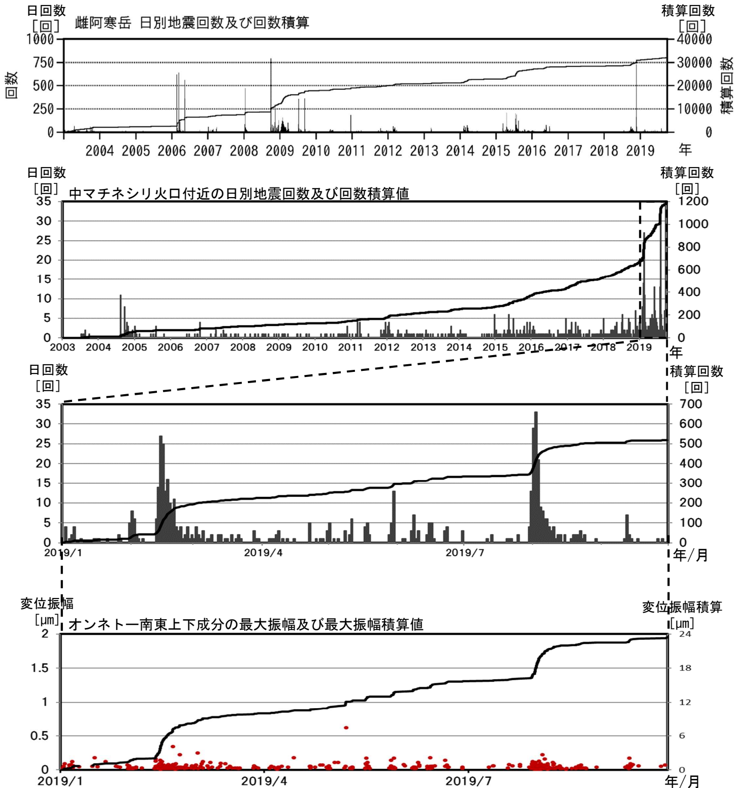
図5 雌阿寒岳 中マチネシリ火口付近の地震の日回数及び最大振幅（2003年1月～2019年9月）
