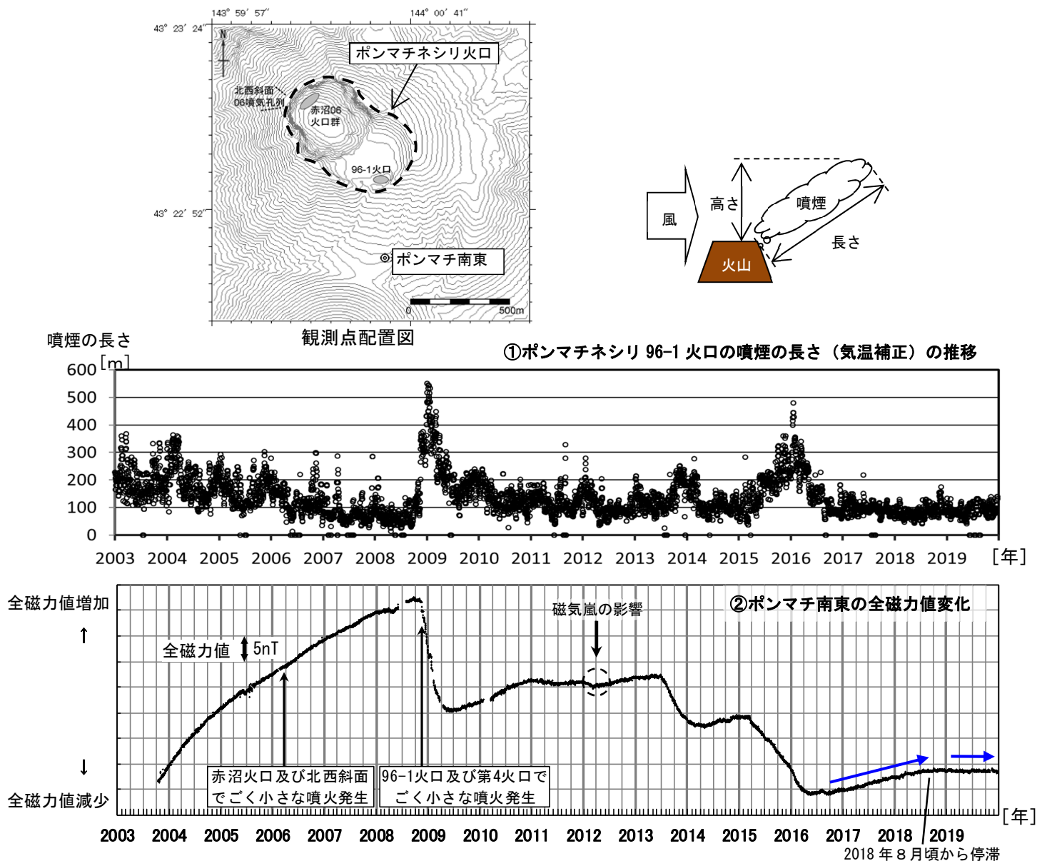
図4 雌阿寒岳 ポンマチネシリ96-1火口の噴煙の長さ（気温補正）と全磁力の比較及び全磁力観測点配置図
