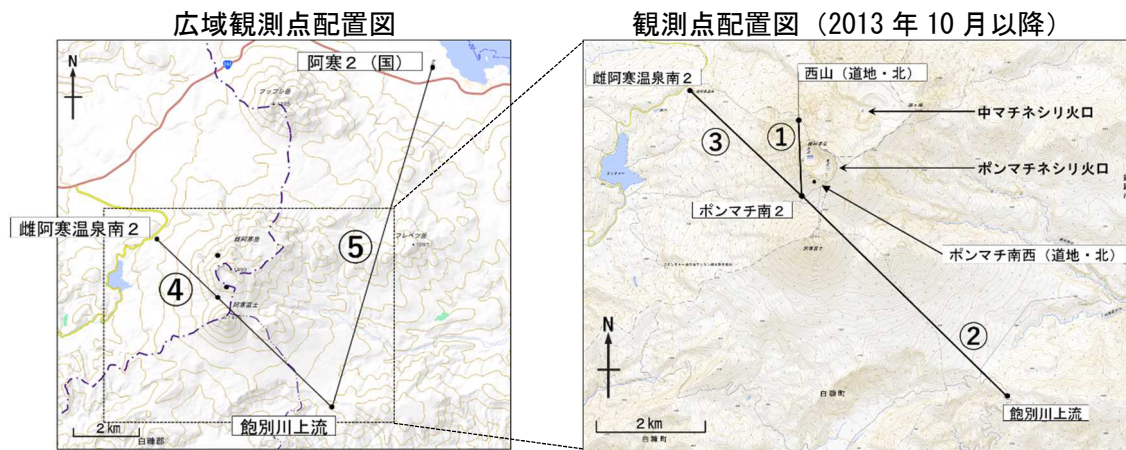
図7 雌阿寒岳 GNSS連続観測による基線長変化（2006年4月～2019年12月）及び観測点配置図
