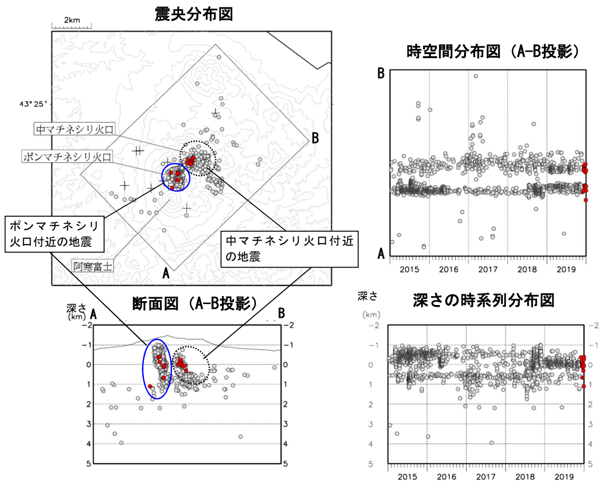
図6 雌阿寒岳 火山性地震の震源分布（2015年1月～2019年12月）
