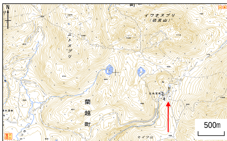
図 1 ニセコ 周辺図と写真の撮影方向（矢印）
