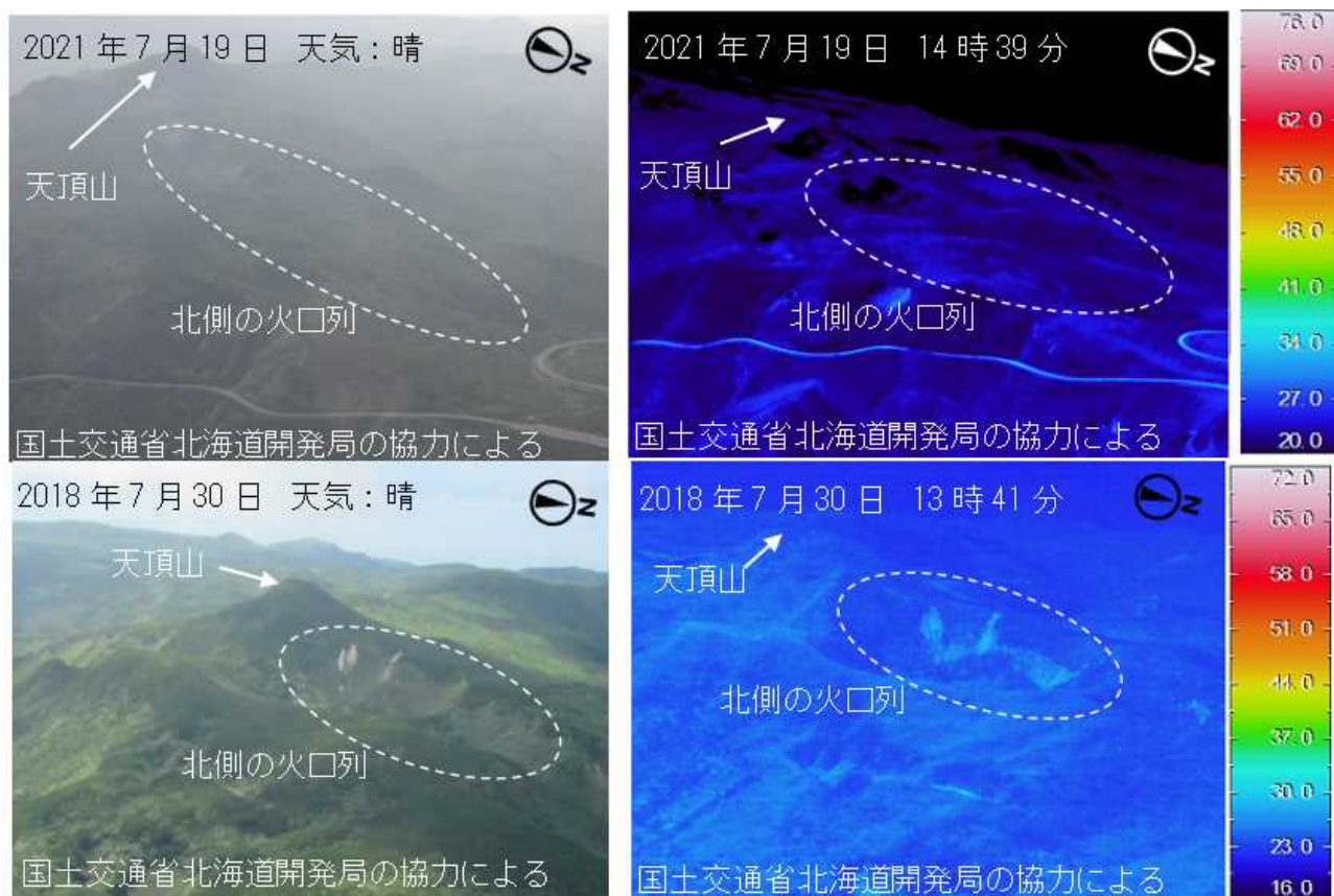
図 3 天頂山 赤外熱映像装置による山頂付近及び北側の火口列の地表面温度分布
