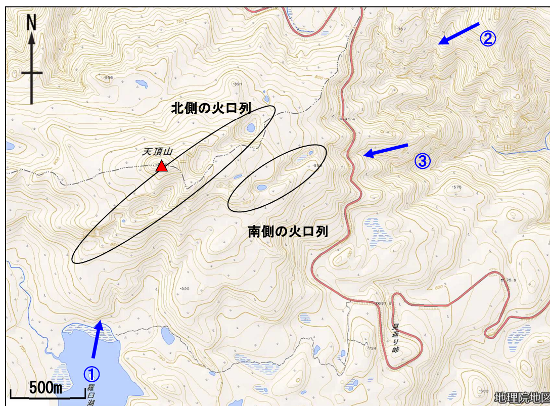
図1 天頂山 周辺図と赤外熱映像及び写真の撮影方向（青矢印）
