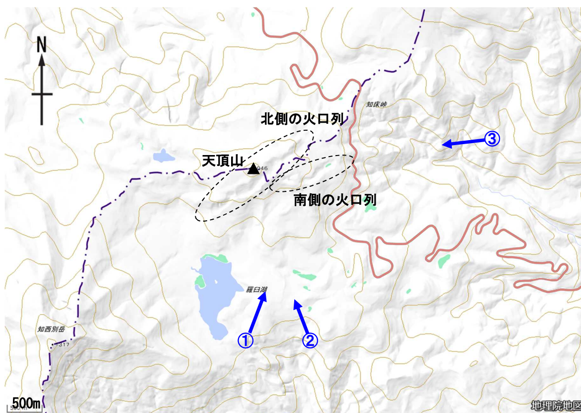
図1 天頂山 周辺図と赤外熱映像及び写真の撮影方向（青矢印）
