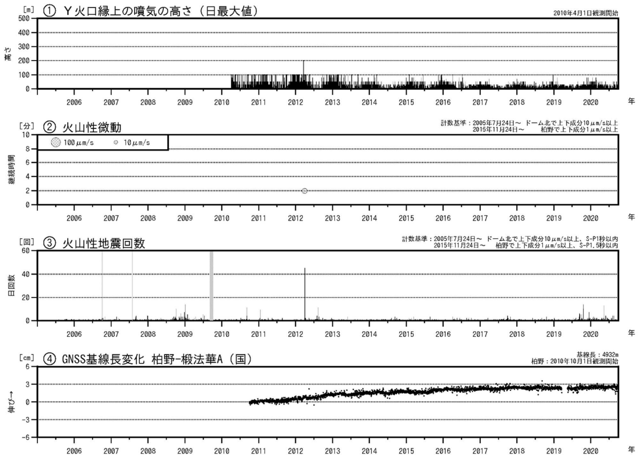
図2 恵山 火山活動経過図（2005年7月～2020年9月）
