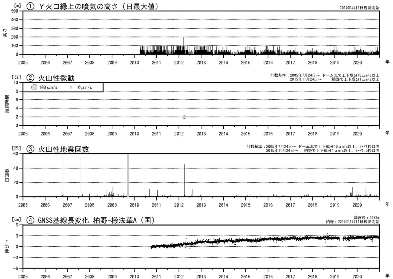
図2 恵山 火山活動経過図（2005年7月～2020年11月）
