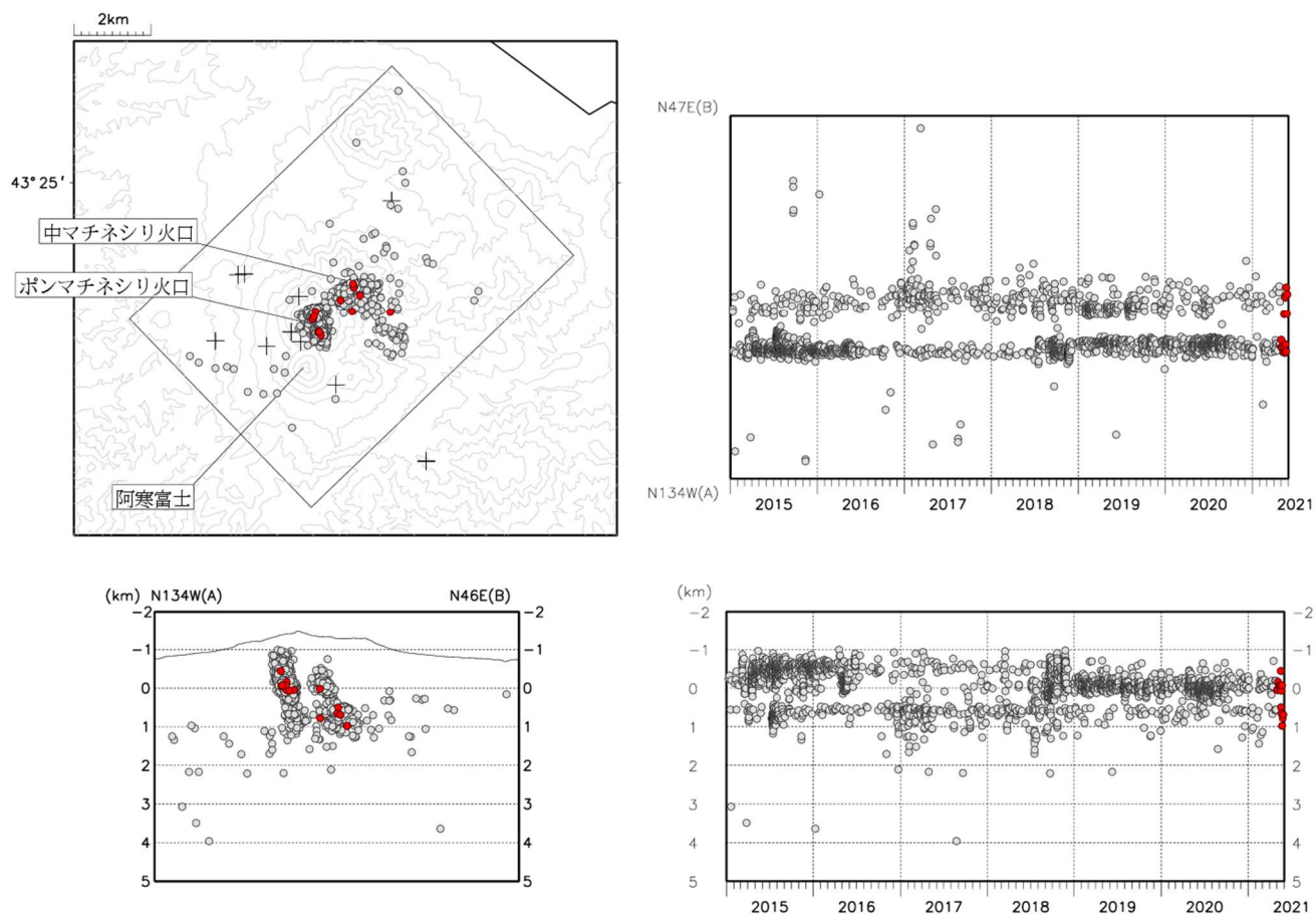
図8 雌阿寒岳 火山性地震の震源分布（2015年1月～2021年5月）
