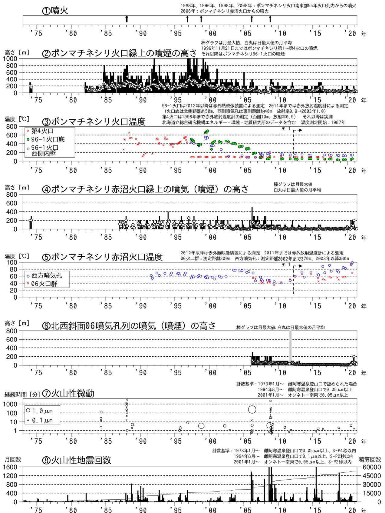
図1 雌阿寒岳 火山活動経過図（1973年1月～2021年5月）
