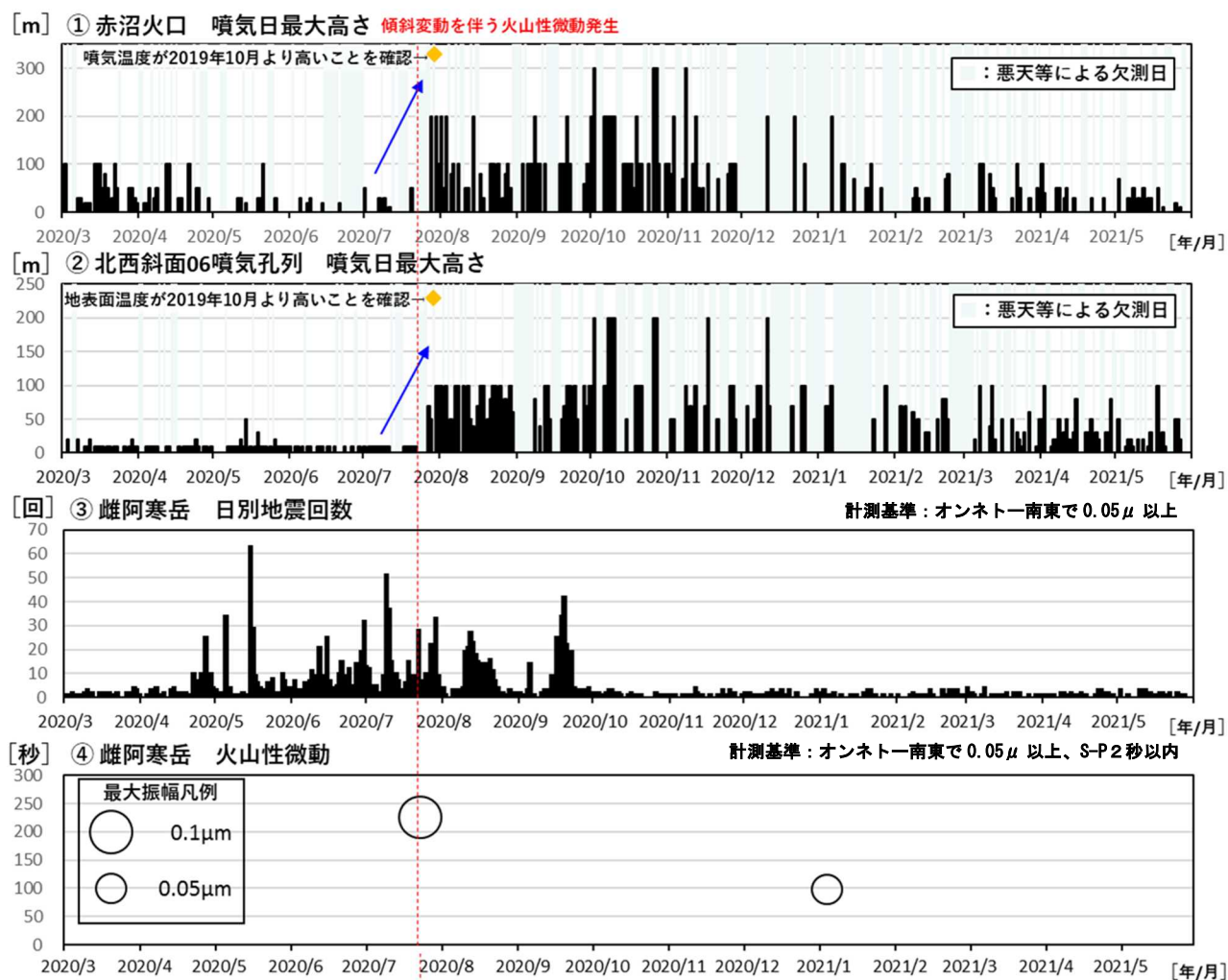
図5 雌阿寒岳 2020年7月以降の噴気活動及び地震活動等の活動経過（2020年3月～2021年5月）
