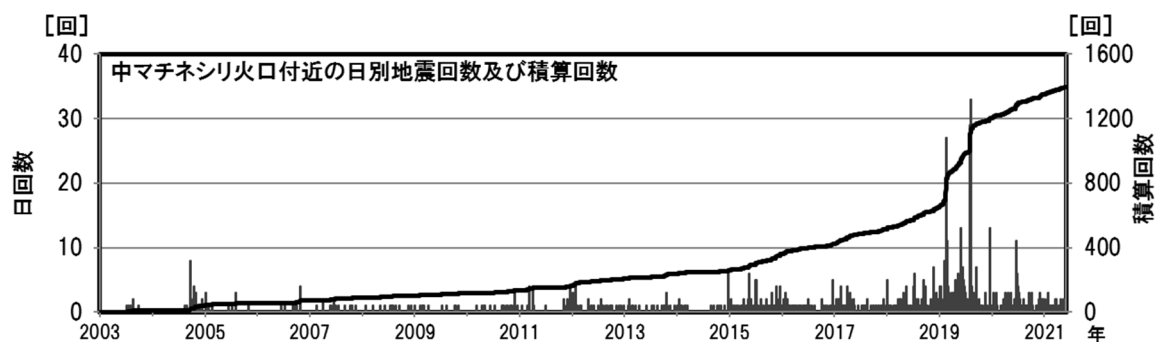
図7 雌阿寒岳 中マチネシリ火口付近の日別地震回数（2003年～2021年5月）
