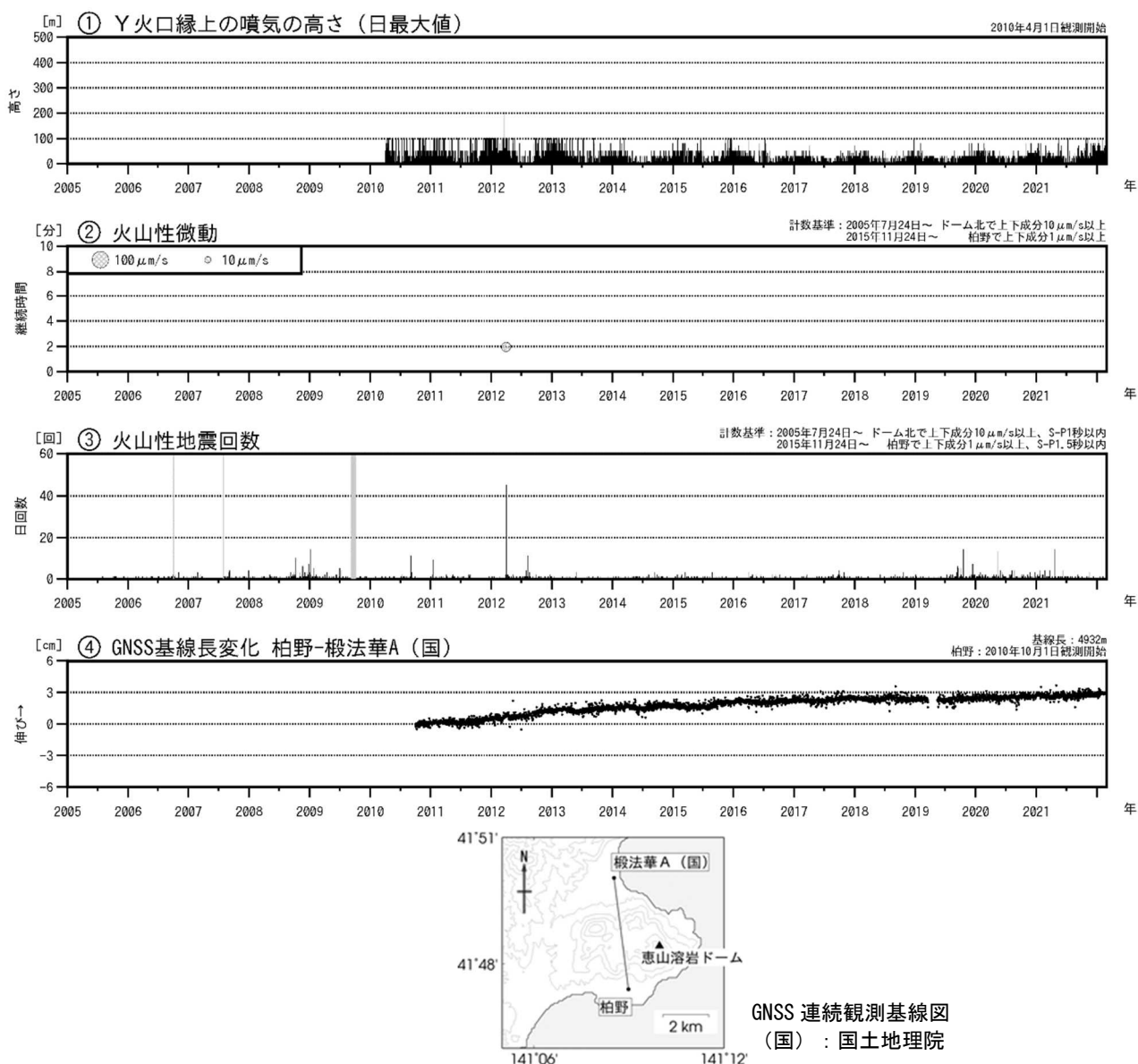
図2 恵山 火山活動経過図（2005年7月～2022年2月）
