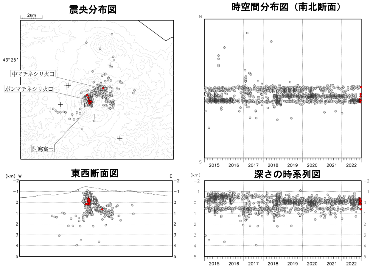
図5 雌阿寒岳 火山性地震の震源分布（2015年1月～2022年12月）
