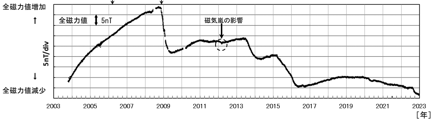
図4 雌阿寒岳 ポンマチネシリ96-1火口の噴煙の長さ と全磁力値の経過及び全磁力観測点配置図 (2003年～2022年12月)
